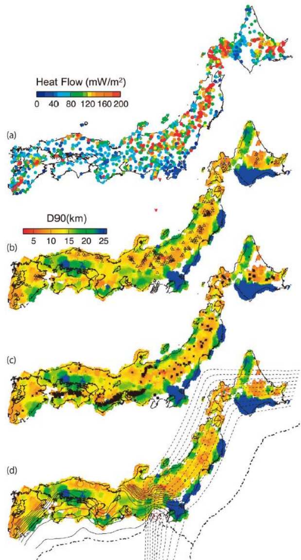
図 17 (a) 地殻熱流量の分布 (Tanaka et al. , 2004). 地殻熱流量をカラースケールで示す。(b) D90 と第四紀火山、(c) D90 と深部低周波地震、(d) D90 と M > 6.5 の地震の分布 (Omuralieva et al. , submitted). D90 をカラースケールで、第四紀火山を三角で、深部低周波地震を×で、 M > 6.5 の地震を赤丸で示す。太平洋スラブおよびフィリピン海スラブ上面の深さを破線および実線のコンターで示す。
