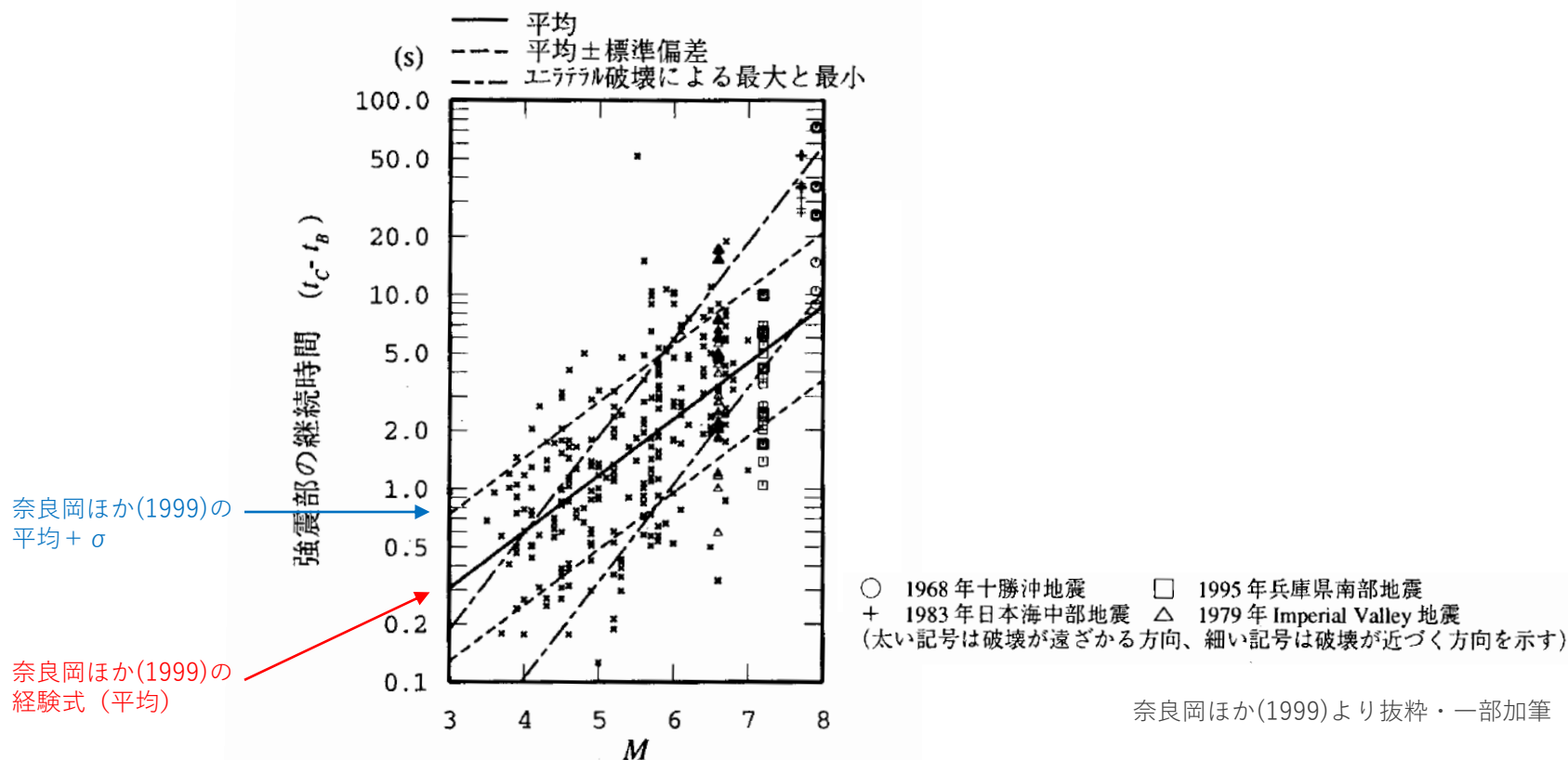
奈良岡ほか(1999)による強震部の継続時間と地震規模Mとの関係（水平動）
