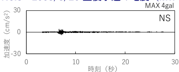
No.3 : 2003/3/26 豊後水道の地震 (Mw4.2)
