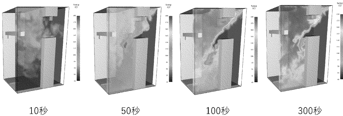
図 5 温度の挙動
