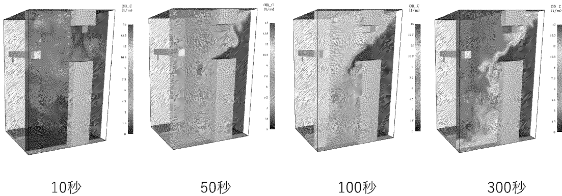
図 4 煙濃度の挙動
