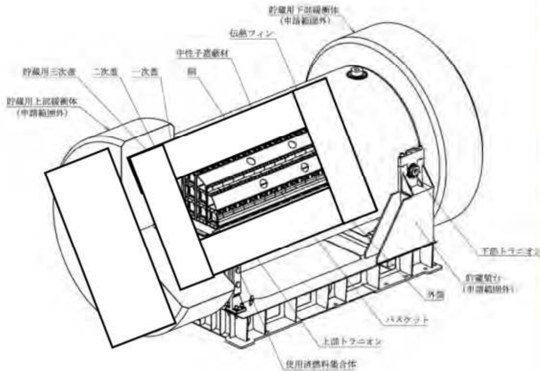
蓋部が金属部へ衝突しない設置方法(横置き) 【認可済みの設置方法】
