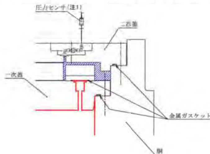
閉じ込め機能の監視構造
