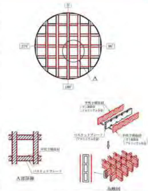
バスケット構造図
