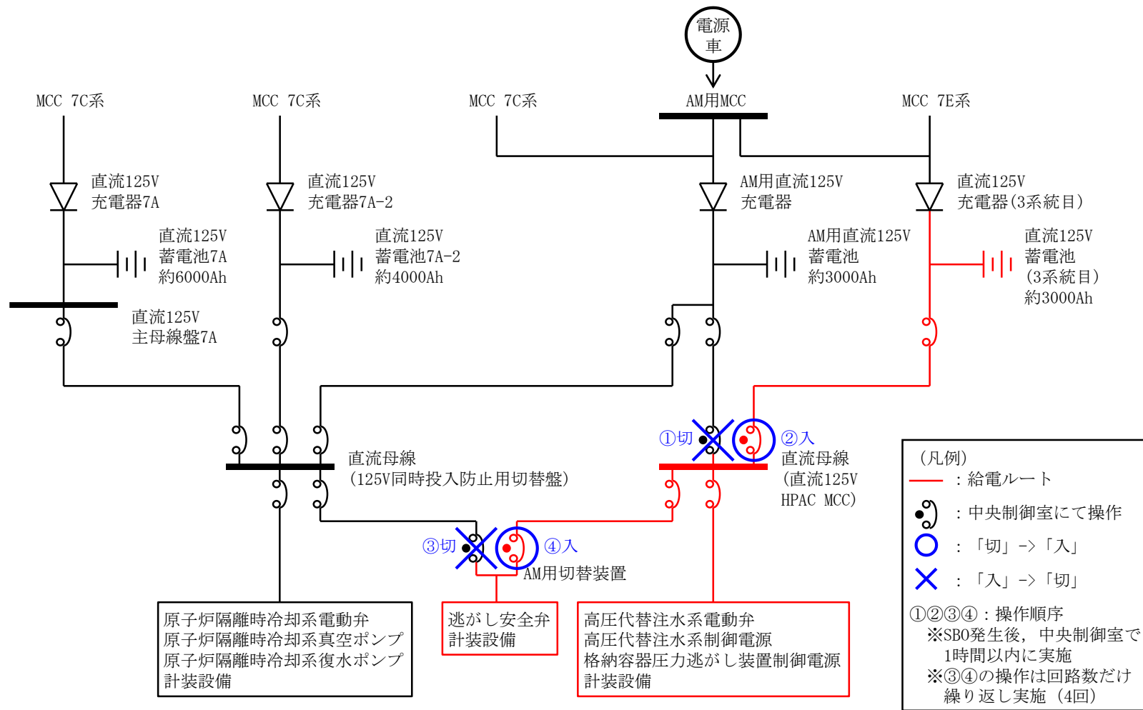
第 57-4-4 図 所内常設直流電源設備 (3 系統目) から給電される系統 (7 号炉)
