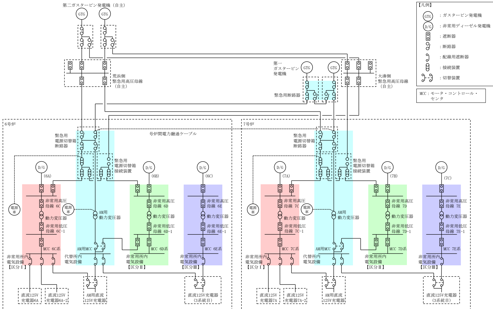
第 57-4-7 図 直流電源設備の受電元系統図
