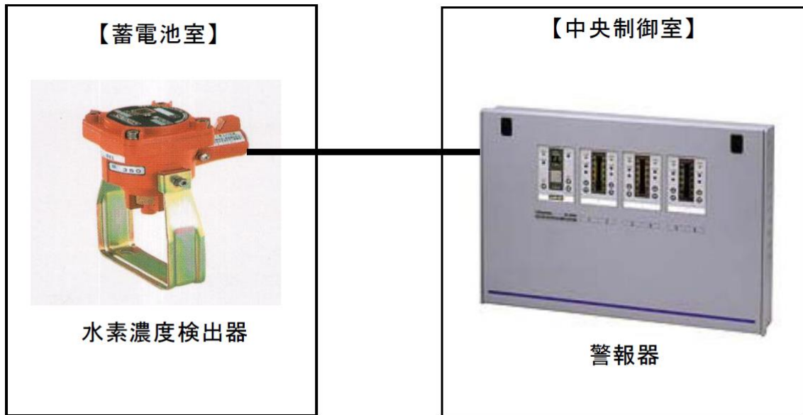
第 41-2-1 図 水素濃度検出設備の例
