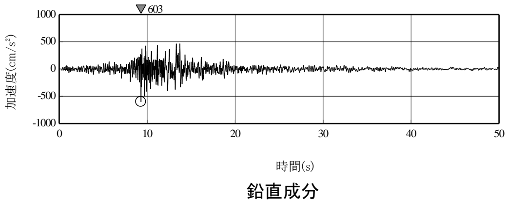
解放基盤表面における標準応答スペクトルを考慮した地震動(実位相による検討) 加速度波形
