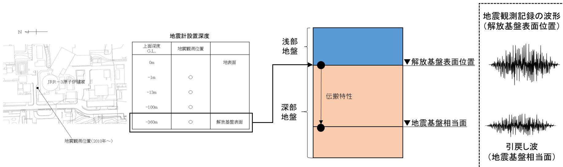
JRR-3 地震観測位置
