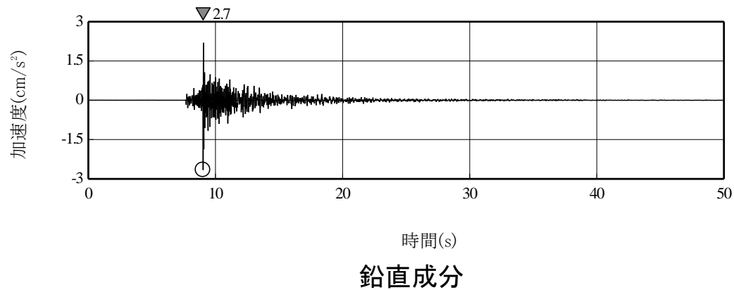
地震基盤相当面における地震観測記録(2011年7月16日(Mw3.8)) 加速度波形
