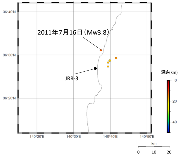
震央分布図
