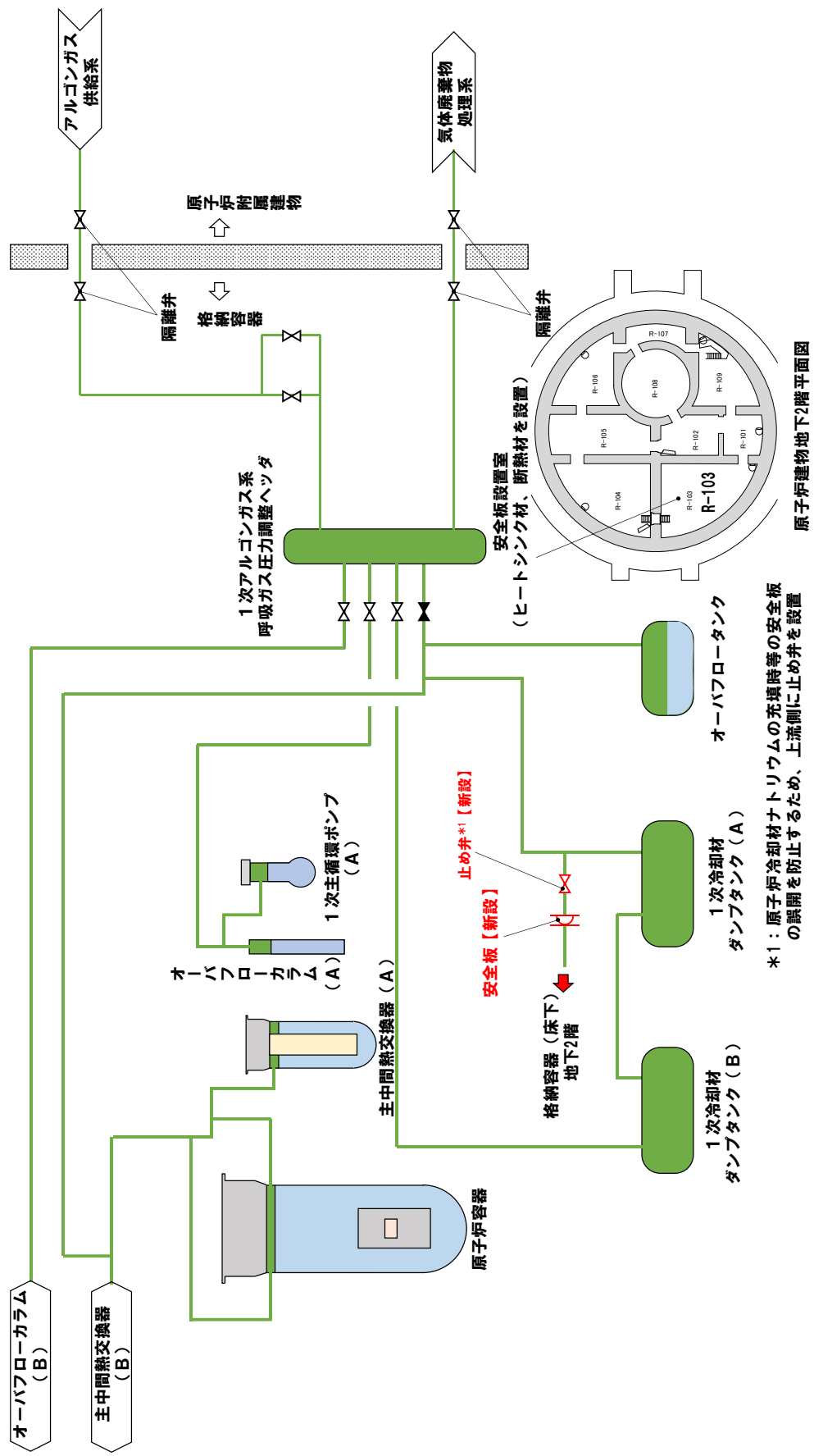
第3.6.1.3.1 図 コンクリート遮へい体冷却系による安全容器外面冷却の補足 (3/3: 1次アルゴンガス系安全板の概念図)
