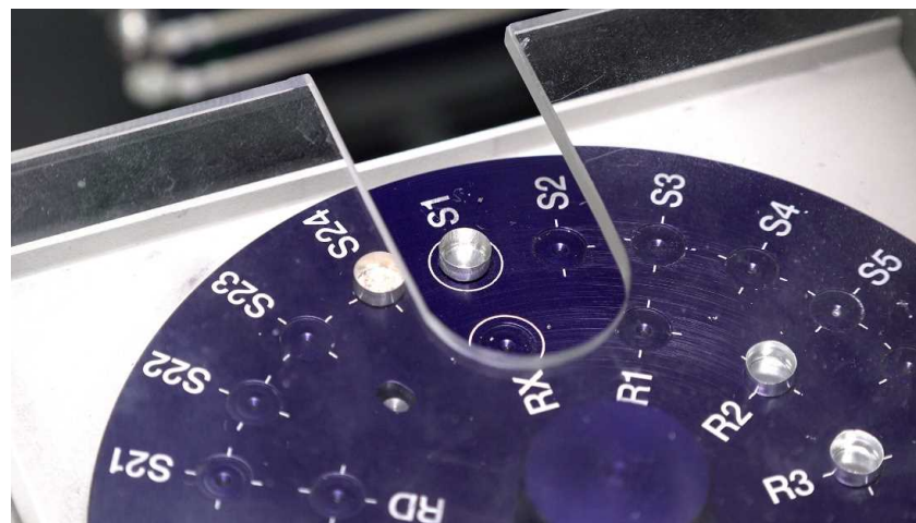
試料加熱後の状態
