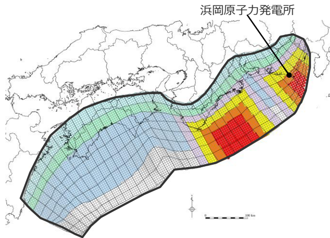
検討波源モデルDの敷地に近い大すべり域の位置を東へ20km、大すべり域間の距離を20kmとしたケース
