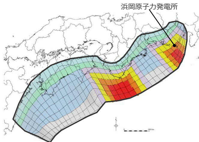
検討波源モデルDの敷地に近い大すべり域の位置を基準位置、大すべり域間の距離を80kmとしたケース
