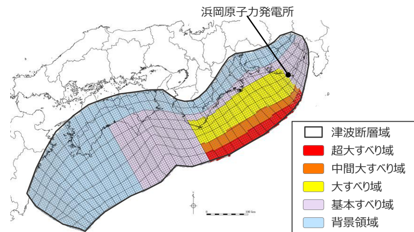
日本海溝の津波評価手法モデル③ (Δσ3.0MPa、RT150s) の大すべり域の位置を西へ50kmとしたケース
