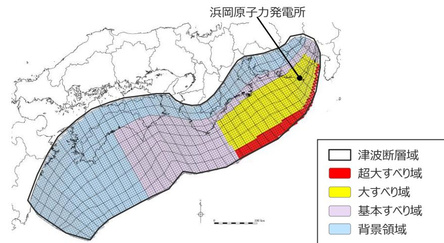
日本海溝の津波評価手法モデル② ( \Delta\sigma 3.0\text{MPa} 、RT150s) の大すべり域の位置を東へ10kmとしたケース
