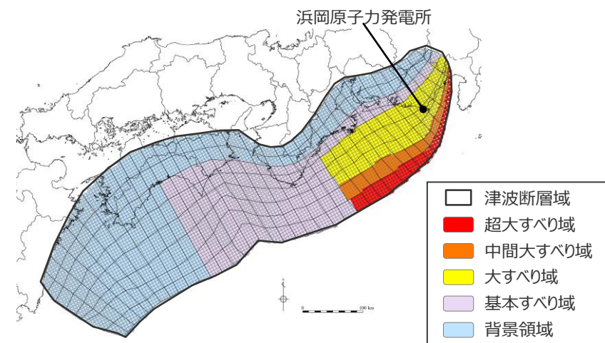
日本海溝の津波評価手法モデル③ ( \Delta\sigma 3.0\text{MPa} 、 RT150\text{s} ) の大すべり域の位置を東へ40kmとしたケース
