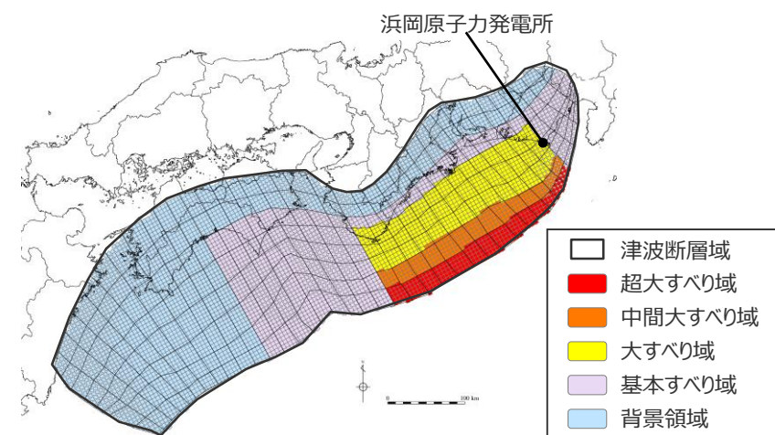
日本海溝の津波評価手法モデル③ ( \Delta\sigma 3.0\text{MPa} 、 RT150\text{s} ) の大すべり域の位置を西へ40kmとしたケース
