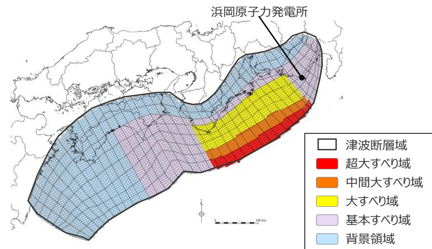
日本海溝の津波評価手法モデル③ ( \Delta\sigma 3.0\text{MPa} 、 RT150\text{s} ) の大すべり域の位置を西へ70kmとしたケース
