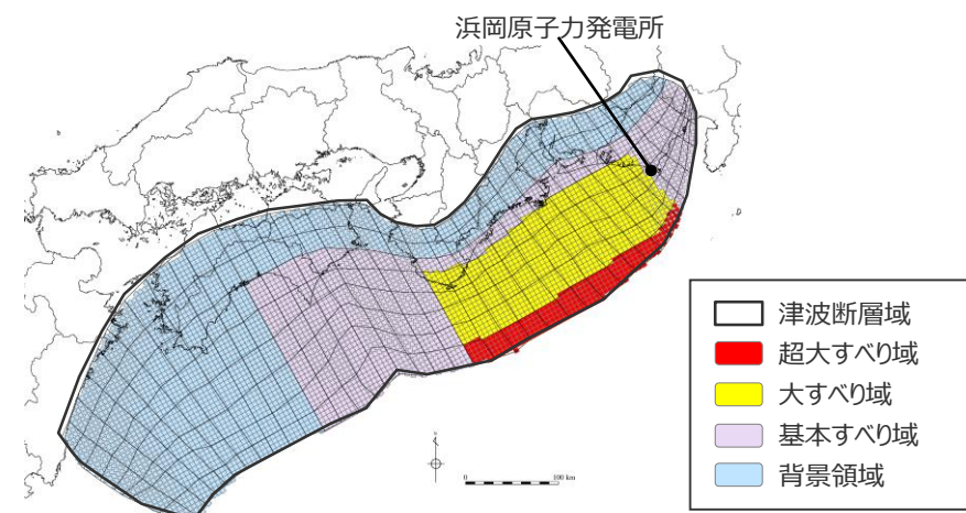
日本海溝の津波評価手法モデル② ( \Delta\sigma 3.0\text{MPa} 、RT150s) の大すべり域の位置を西へ50kmとしたケース
