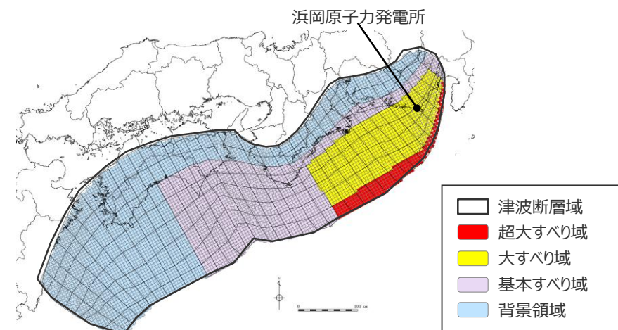
日本海溝の津波評価手法モデル② ( \Delta\sigma 3.0\text{MPa} 、 RT150\text{s} ) の大すべり域の位置を東へ20kmとしたケース
