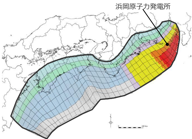
検討波源モデルDの大すべり域の位置を東へ90kmとしたケース
