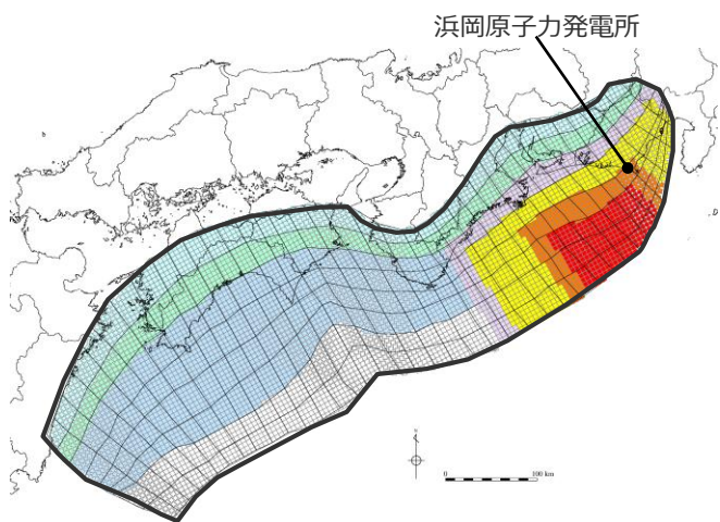
検討波源モデルDの大すべり域の位置を東へ30kmとしたケース
