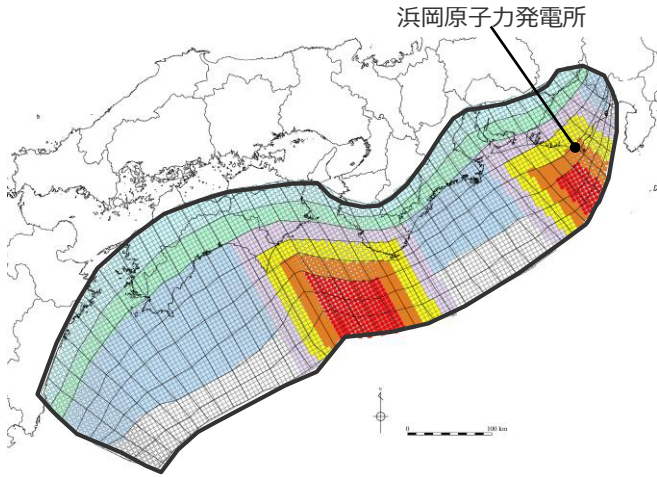
検討波源モデルDの敷地に近い大すべり域の位置を西へ10km、大すべり域間の距離を120kmとしたケース
