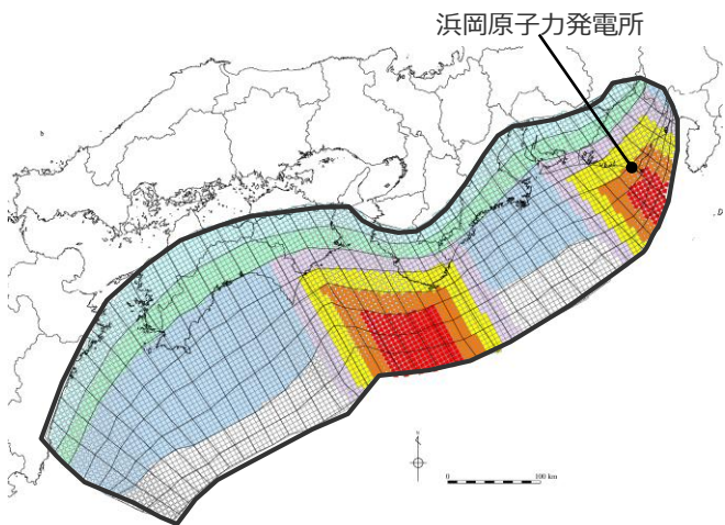
検討波源モデルDの敷地に近い大すべり域の位置を東へ10km、大すべり域間の距離を120kmとしたケース
