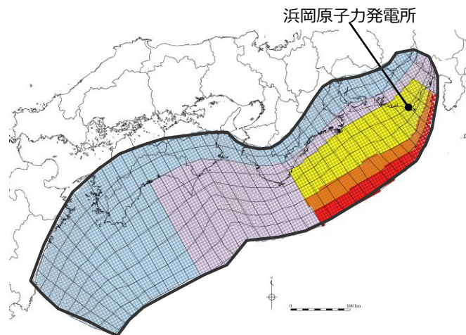
日本海溝の津波評価手法モデル③ (Δσ3.0MPa、RT150s) の大すべり域の位置を基準位置としたケース
