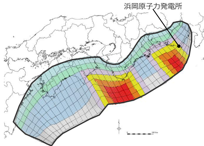
検討波源モデルDの敷地に近い大すべり域の位置を西へ40km、大すべり域間の距離を60kmとしたケース
