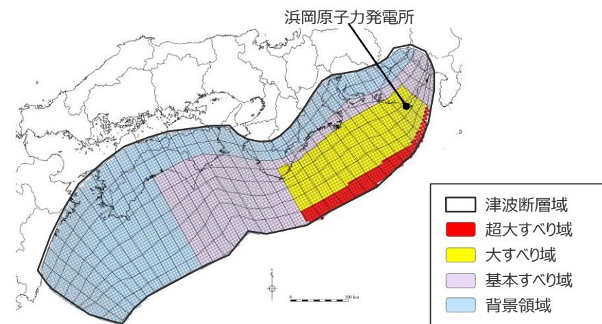
日本海溝の津波評価手法モデル② ( \Delta\sigma 3.0\text{MPa} 、 RT150\text{s} ) の大すべり域の位置を西へ20kmとしたケース
