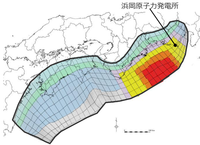
検討波源モデルDの大すべり域の位置を西へ20kmとしたケース
