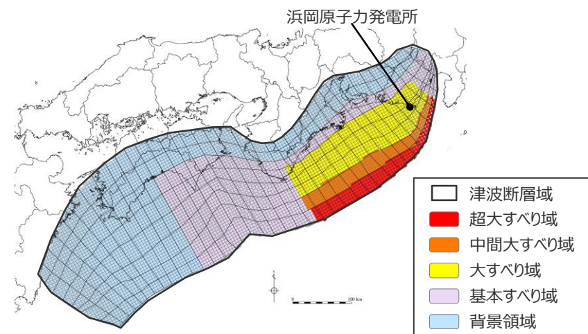
日本海溝の津波評価手法モデル③ ( \Delta\sigma 3.0\text{MPa} 、 RT150\text{s} ) の大すべり域の位置を西へ10kmとしたケース
