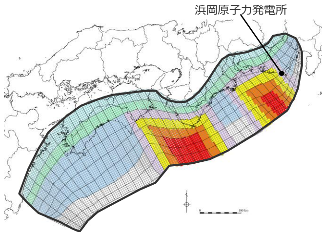
検討波源モデルDの敷地に近い大すべり域の位置を西へ50km、大すべり域間の距離を50kmとしたケース
