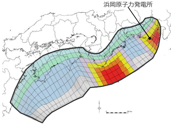
検討波源モデルDの敷地に近い大すべり域の位置を東へ40km、大すべり域間の距離を80kmとしたケース
