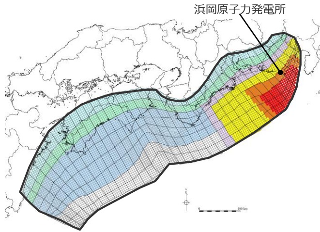
検討波源モデルDの大すべり域の位置を東へ70kmとしたケース
