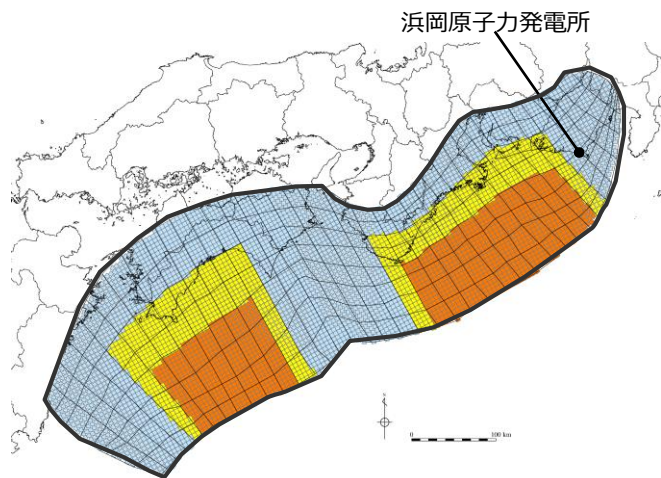
日本海溝の津波評価手法モデル① ( \Delta\sigma 3.0\text{MPa} 、 RT150\text{s} ) の大すべり域の位置を西へ60kmとしたケース
