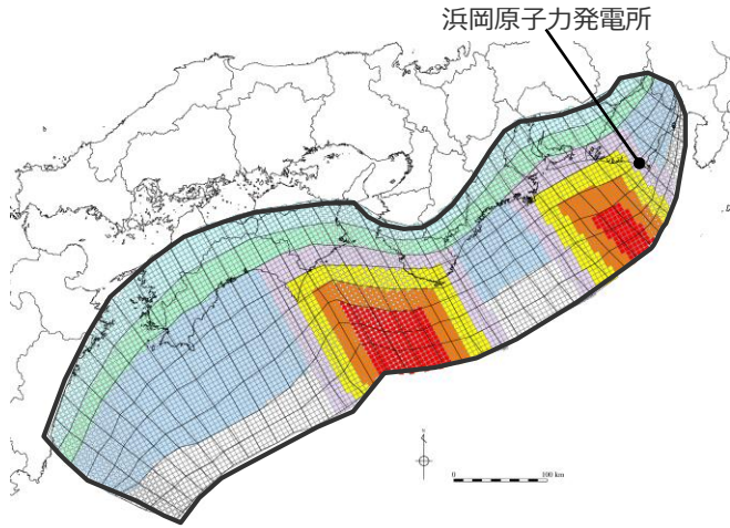
検討波源モデルDの敷地に近い大すべり域の位置を西へ50km、大すべり域間の距離を80kmとしたケース
