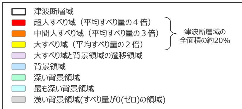
西 ← 検討波源モデルDの大すべり域の位置を西へ50kmとしたケースの小断層のすべり量分布 (m) ⇨ 東
