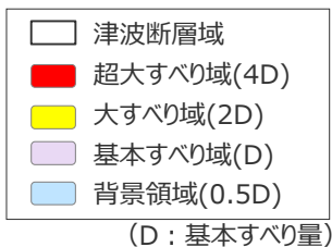
日本海溝の津波評価手法モデル②
