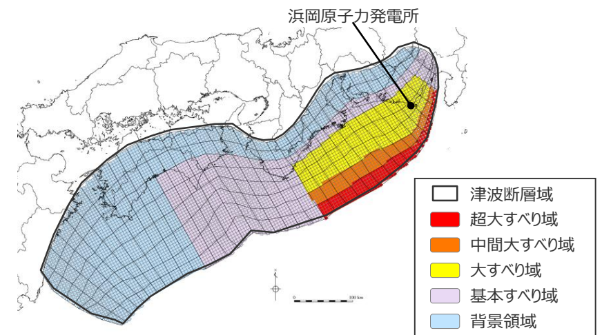
日本海溝の津波評価手法モデル③ (Δσ3.0MPa、RT150s)
