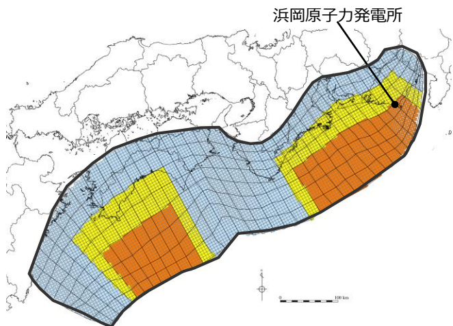
日本海溝の津波評価手法モデル①の 大すべり域の位置を基準位置としたケース
