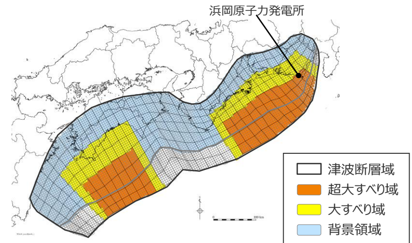
検討波源モデルCの大すべり域の位置を基準位置としたケース
