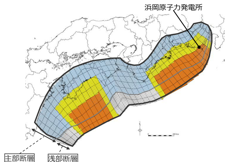
検討波源モデルC の大すべり域の位置を基準位置としたケース
