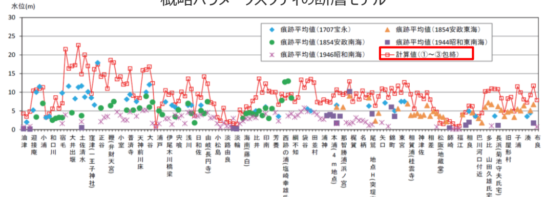
概略パラメータスタディの計算結果包絡値と津波痕跡高との比較
