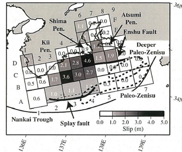
Baba et al.(2006)による波源モデル
