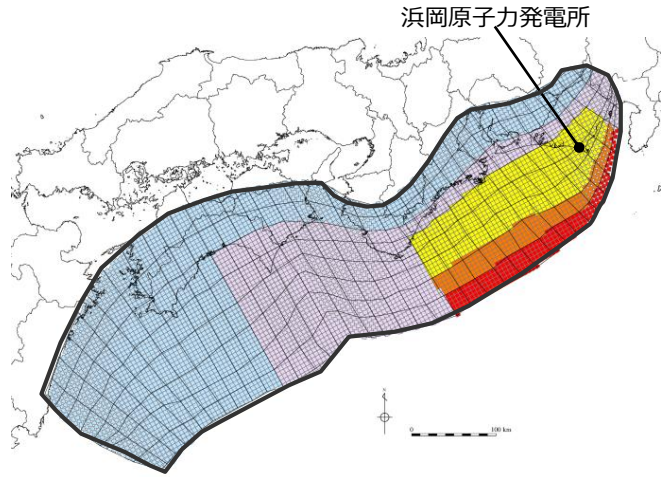
日本海溝の津波評価手法モデル③ ( \Delta\sigma 3.0\text{MPa} 、RT150s)
