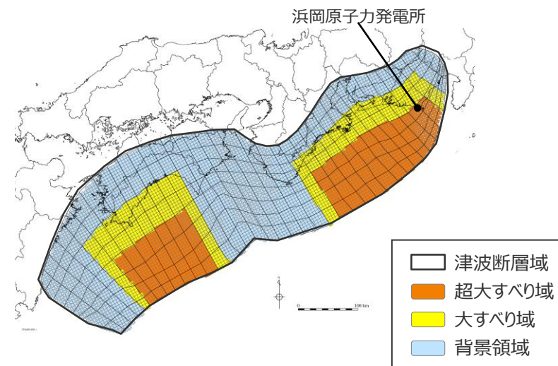
日本海溝の津波評価手法モデル① ( \Delta\sigma 3.0\text{MPa} 、RT150s)
