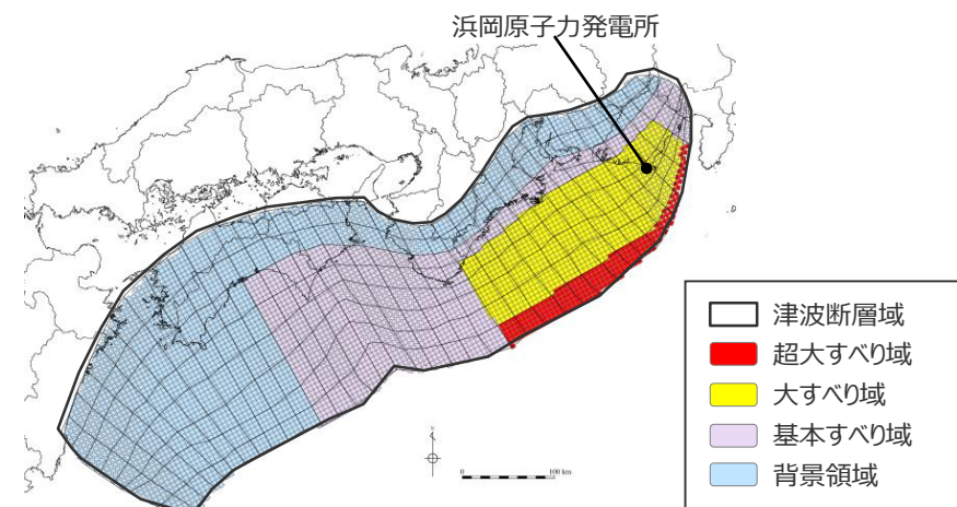
日本海溝の津波評価手法モデル② ( \Delta\sigma 3.0MPa、RT150s)
