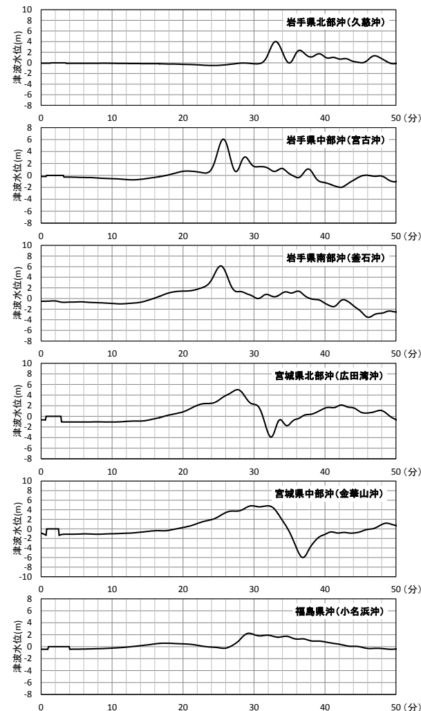
再現対象とするGPS波浪計地点における 東北沖地震時の津波観測波形
