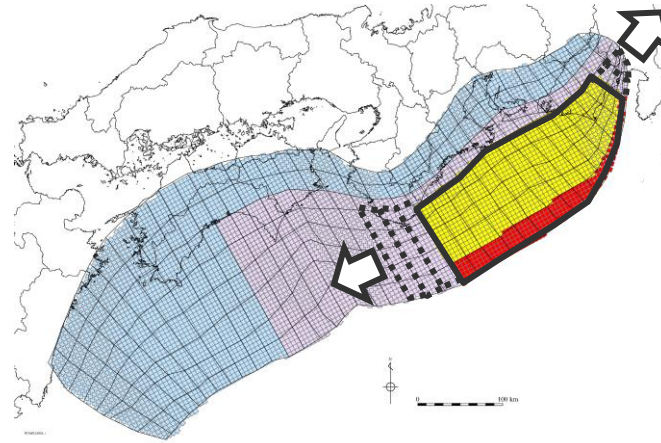
日本海溝の津波評価手法モデル② ( \Delta\sigma 3.0\text{MPa} , RT150s)
