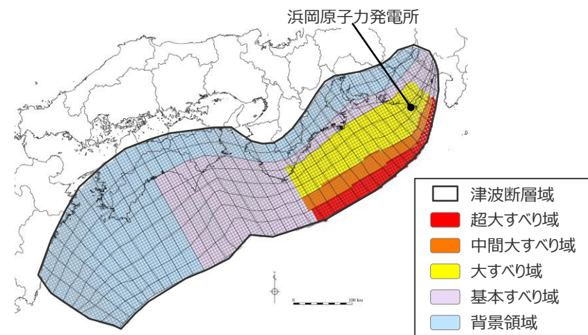
日本海溝の津波評価手法モデル③ の大すべり域の位置を西へ10kmとしたケース
