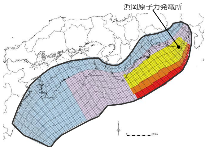
日本海溝の津波評価手法モデル③ の大すべり域の位置を西へ10kmとしたケース
