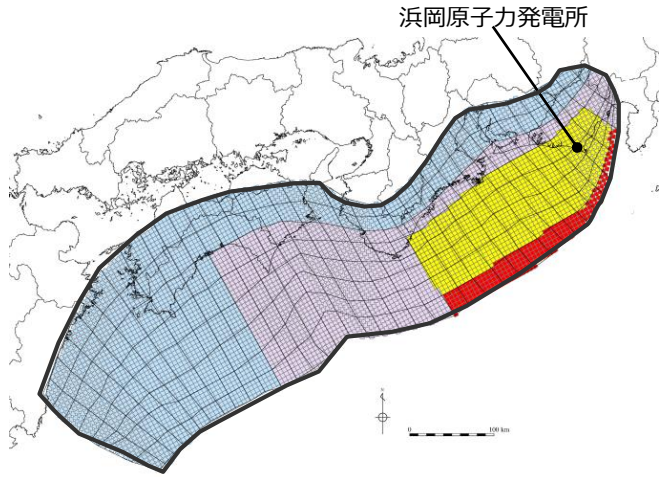
日本海溝の津波評価手法モデル② ( \Delta\sigma 3.0\text{MPa} 、RT150s)
