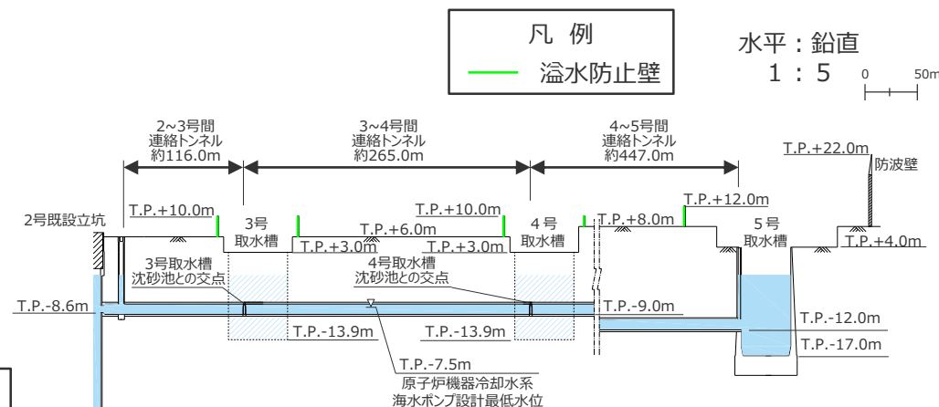
連絡トンネル縦断面図
