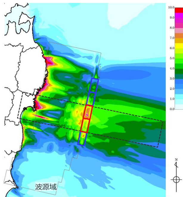
(b)海溝軸付近の大きくすべった領域のすべり分布が不均質なケース
