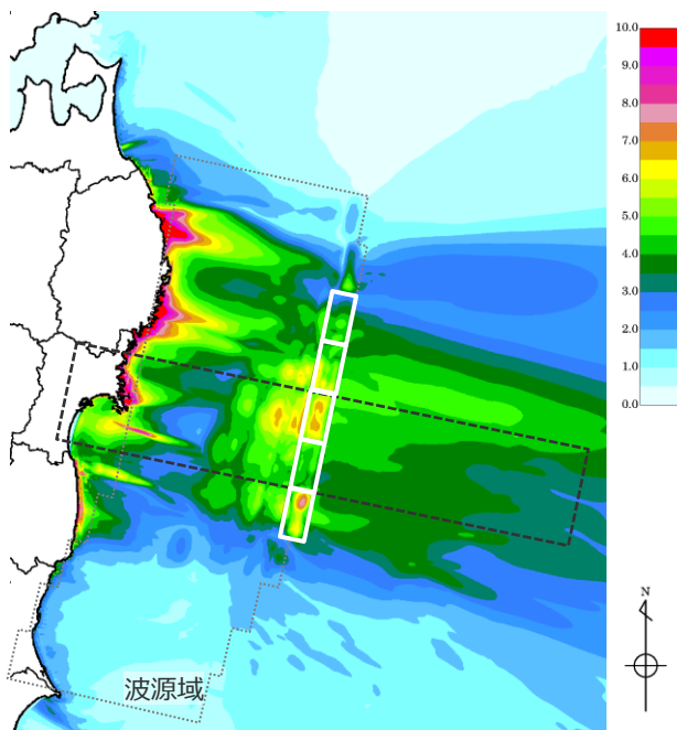
(a)海溝軸付近の大きくすべった領域のすべり分布が一様なケース
