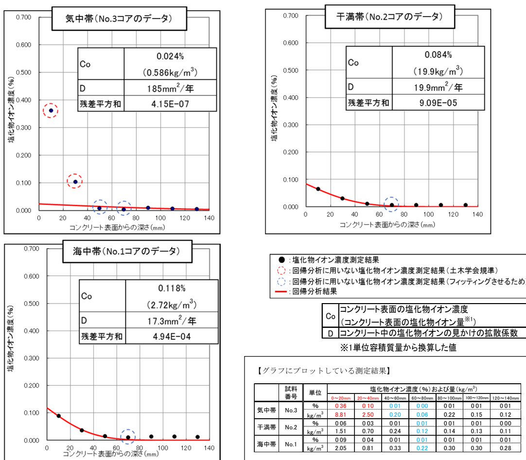
図13-1 拡散方程式の回帰分析結果
