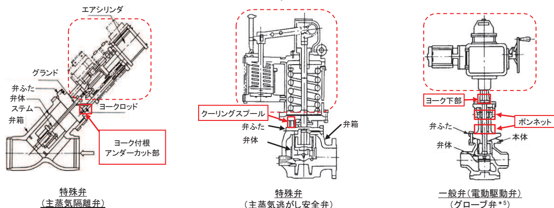
図5-2-2 主な詳細検討対象弁の構造概要
