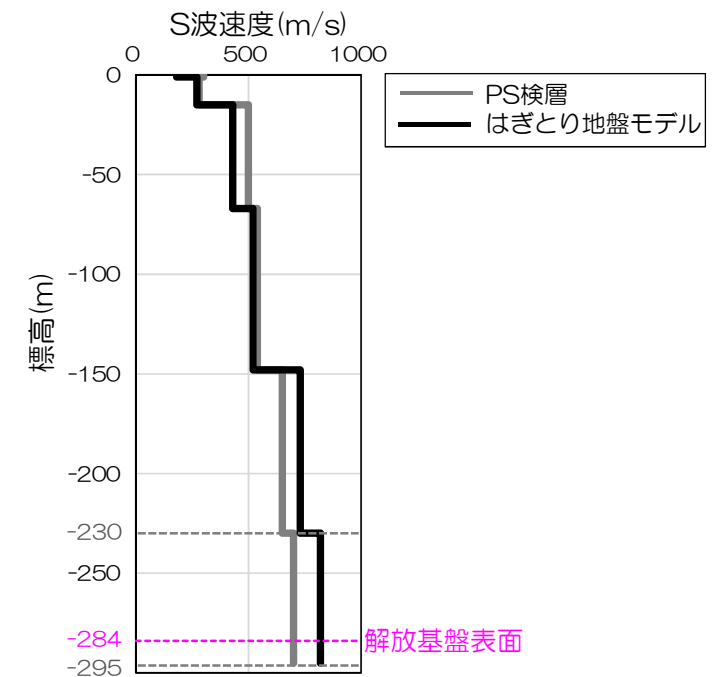
鉛直アレイ観測点のPS検層及びはぎとり地盤モデル
