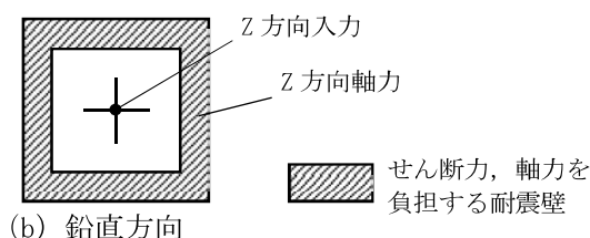
図4-1 入力方向ごとの耐震要素
