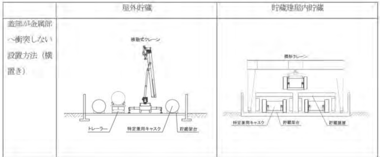
第12図 特定兼用キャスク貯蔵施設概要図 (例)
