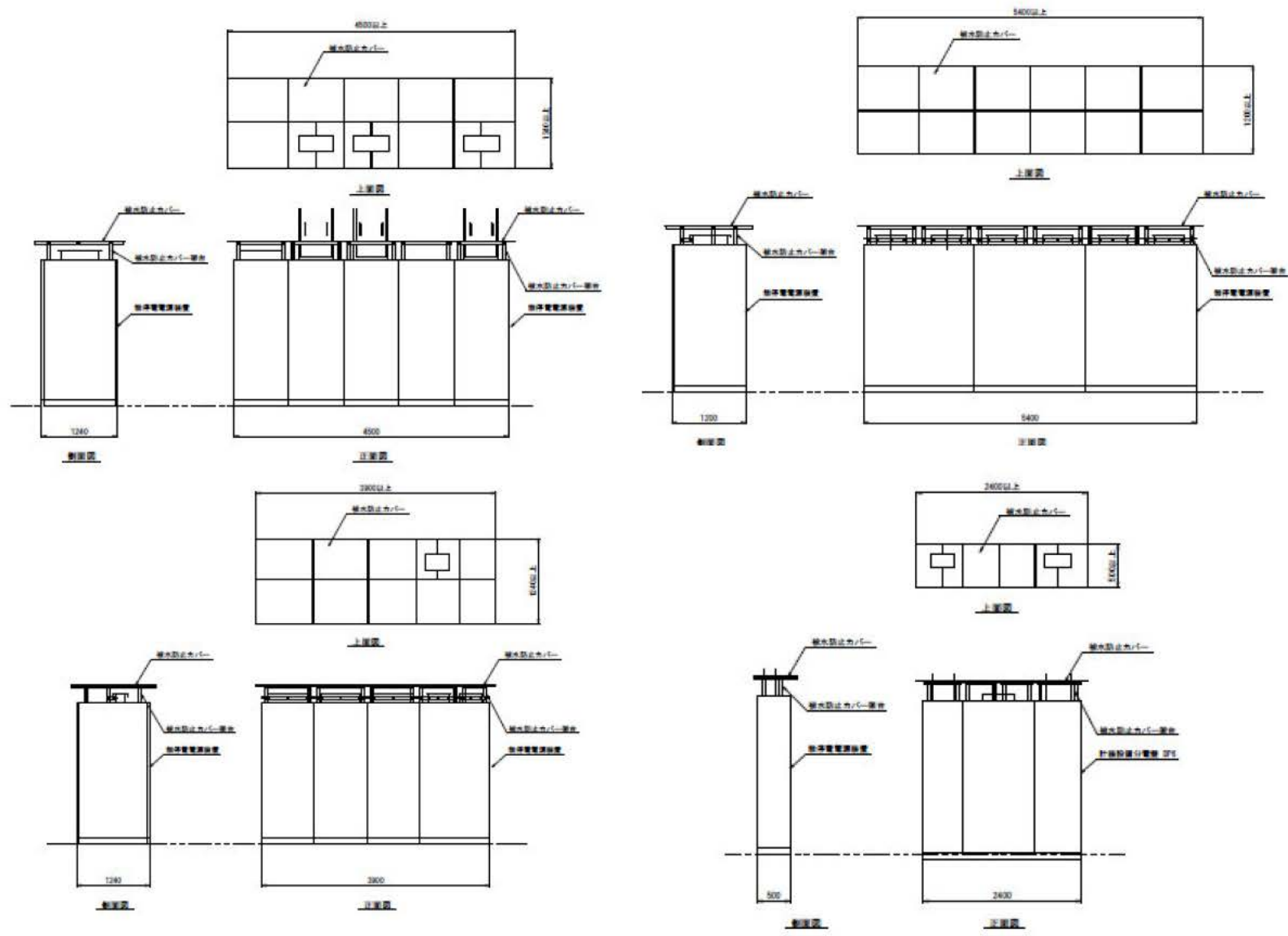
別図-8 被水防止板の概要 (3階 無停電電源装置、計装用分電盤 DP6) (6/6)
