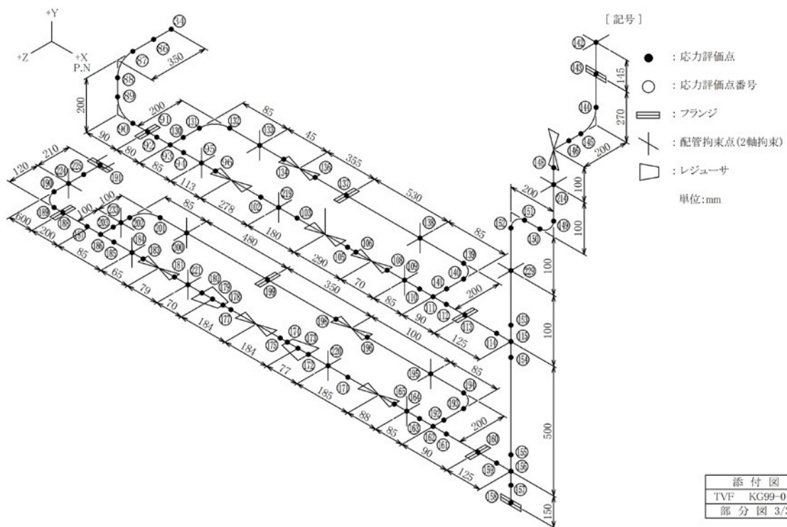
図-4-14 蒸気配管（空調設備）（KG99-018）の解析モデル（3/3）
