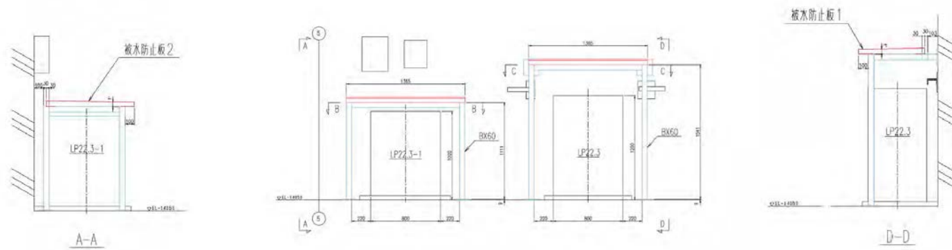
別図－8 被水防止板の概要（地下2階 重量計盤）（3/6）
