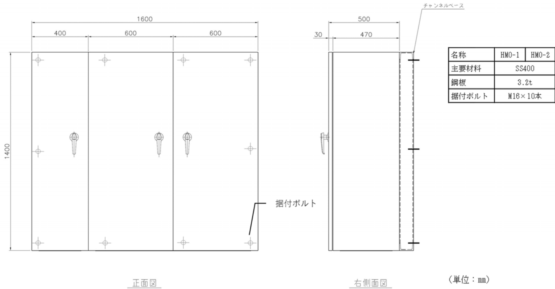
別図-8 緊急電源接続盤の概要
