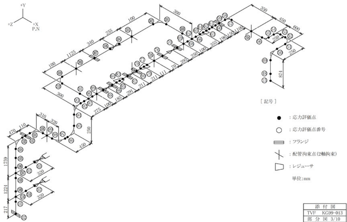
図-4-11 蒸気配管（空調設備）（KG99-013）の解析モデル（3/10）
