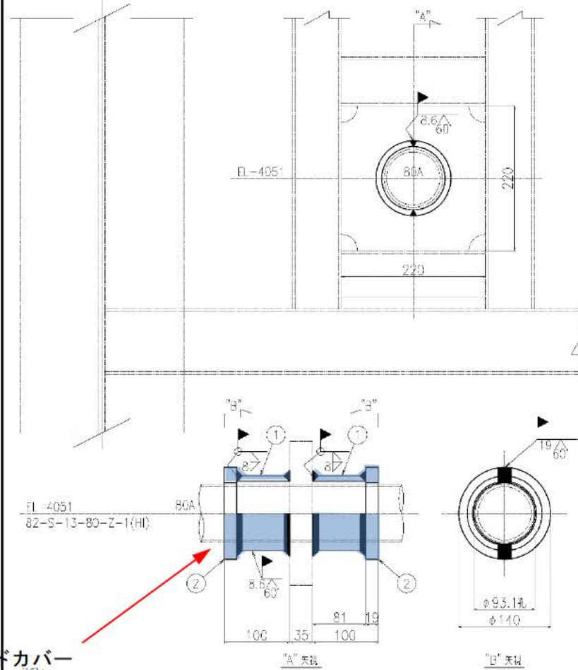
ターミナルエンドカバー図面
