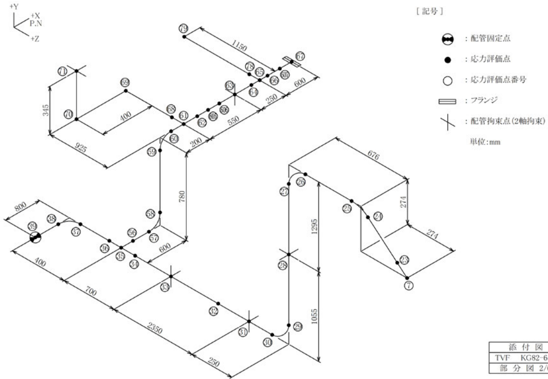
図-4-5 蒸気配管 (KG82-612) の解析モデル (2/6)
