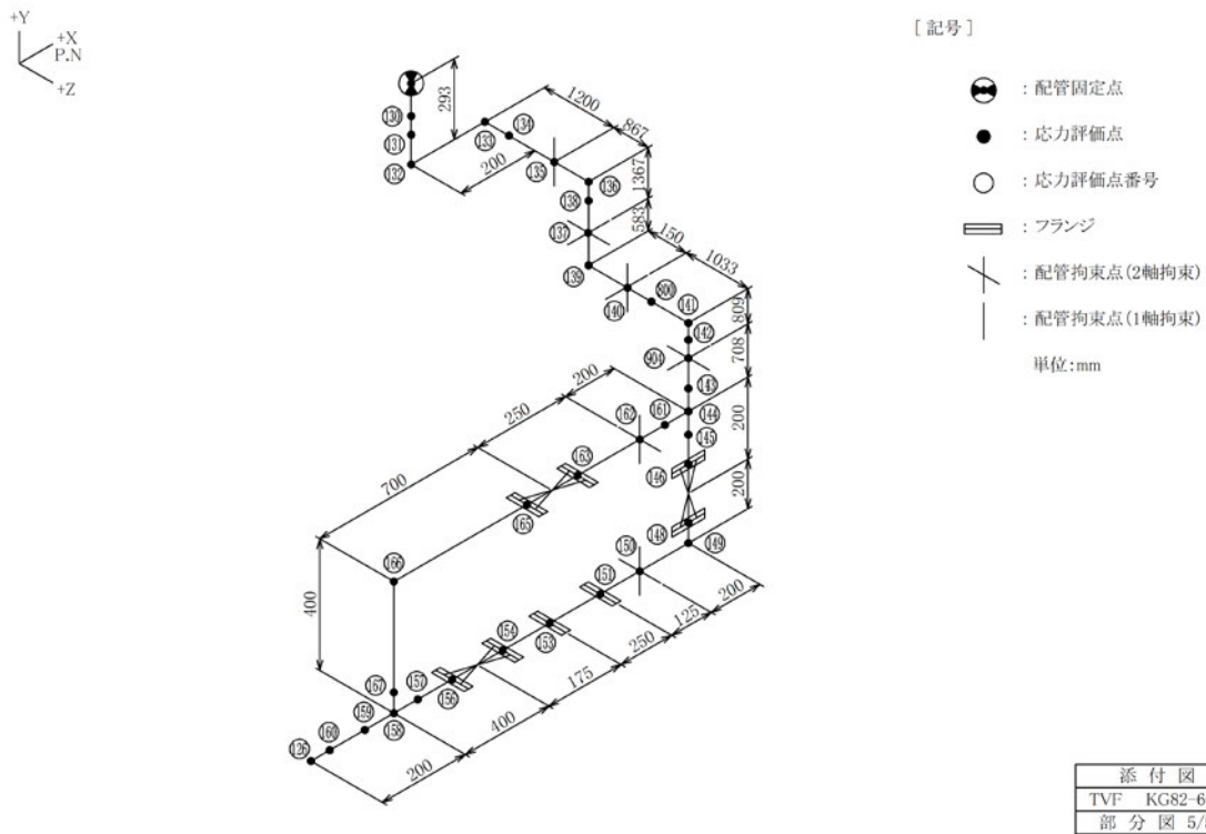
図-4-4 蒸気配管 (KG82-607) の解析モデル (5/5)
