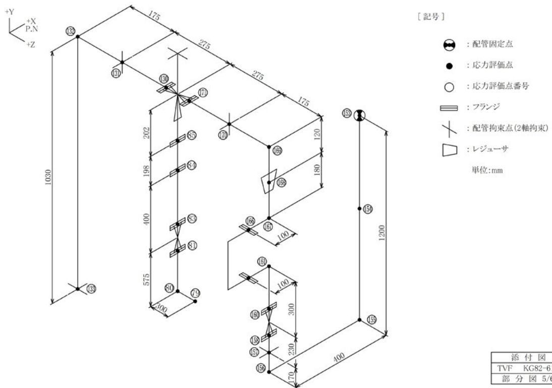
図-4-5 蒸気配管 (KG82-612) の解析モデル (5/6)
