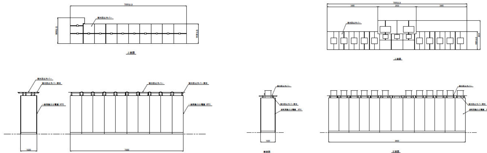
別図－8 被水防止板の概要（3階 VFP3）（4/6）
