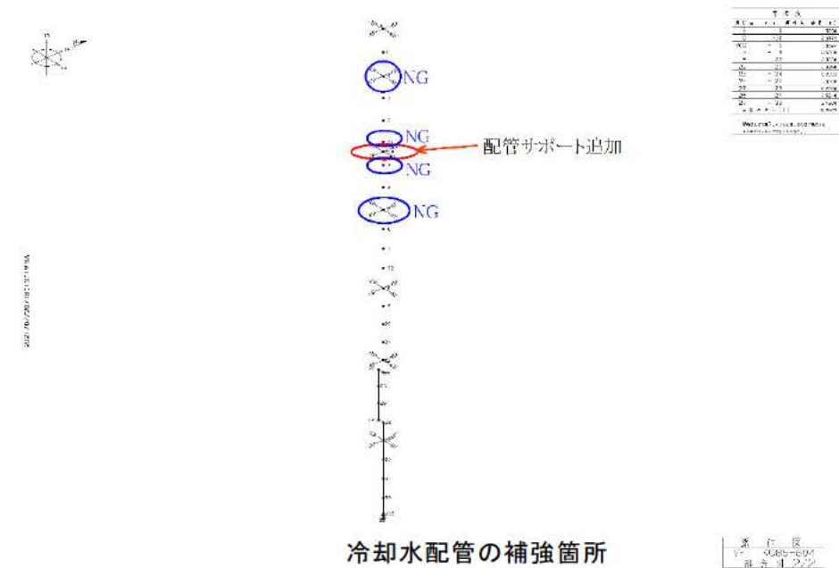
別図-1 配管の補強対策の概要
