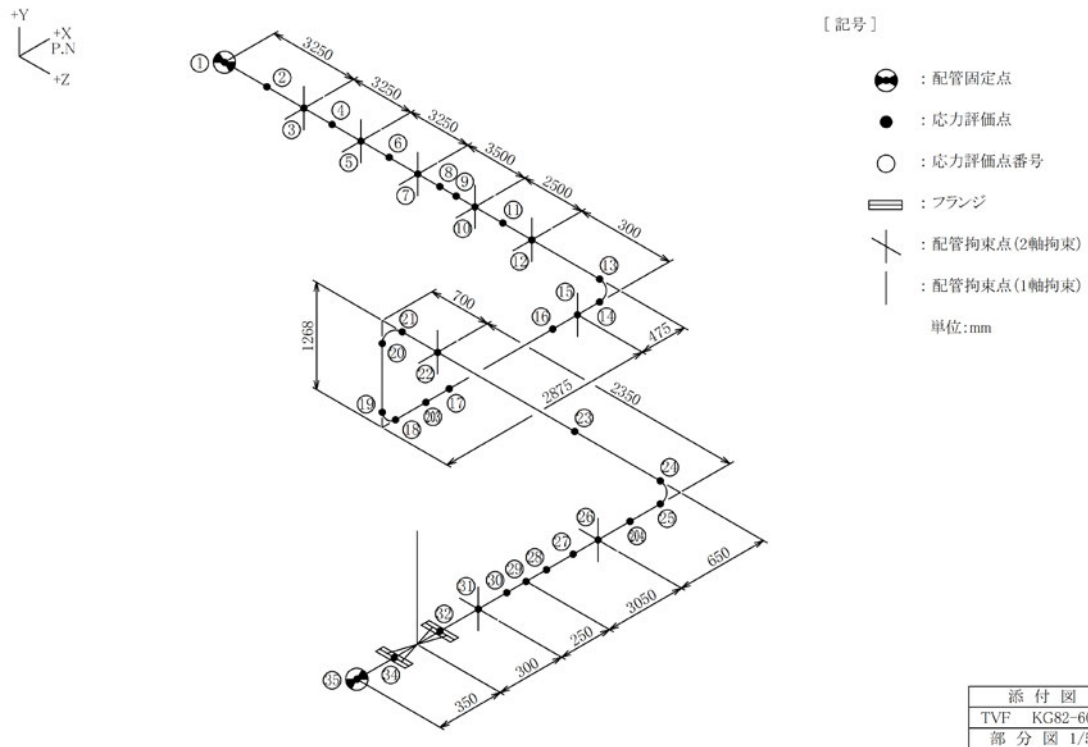
図-4-4 蒸気配管 (KG82-607) の解析モデル (1/5)
