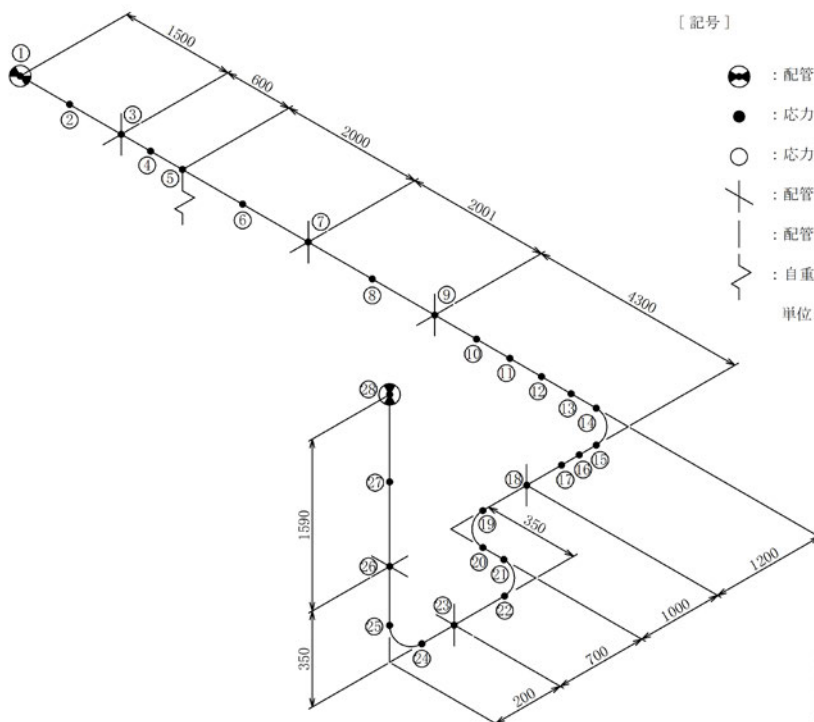
図-4-10 蒸気配管 (空調設備) (KG99-010) の解析モデル
