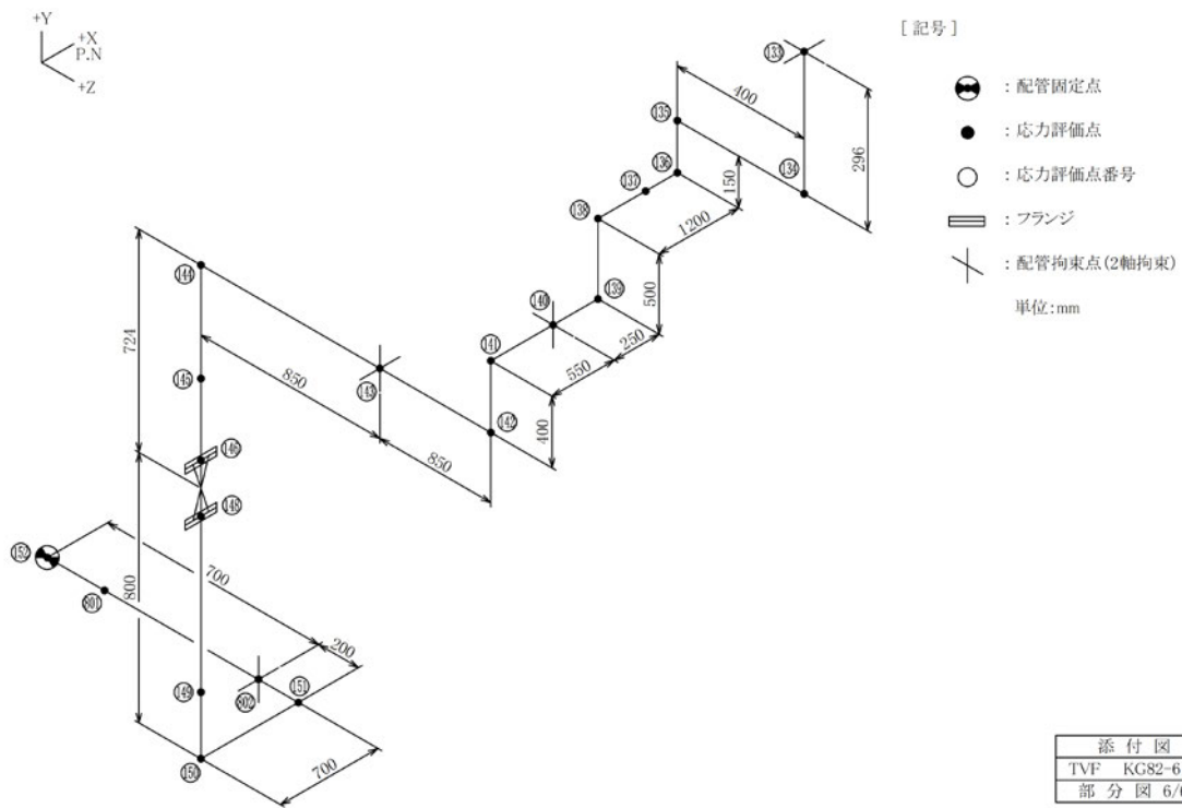
図-4-5 蒸気配管 (KG82-612) の解析モデル (6/6)
