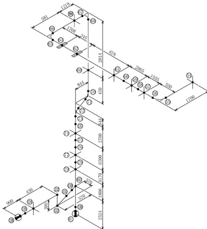
図-4-6 冷却水配管 (KG83-652) の解析モデル (3/3)
