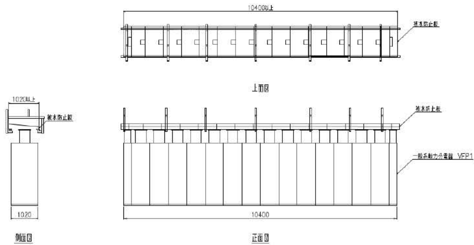
別図－8 被水防止板の概要（地下2階 VFP1）（1/6）
