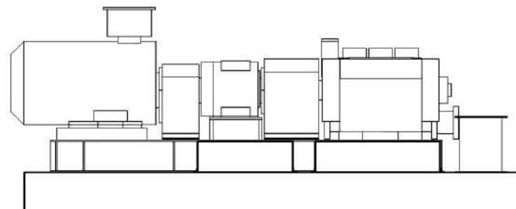
別図-14 オイルパン設置概略図 (ポンプ G22P11)
