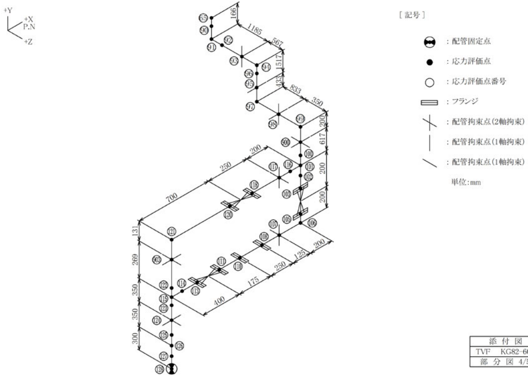
図-4-4 蒸気配管 (KG82-607) の解析モデル (4/5)
