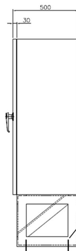
右側面図
