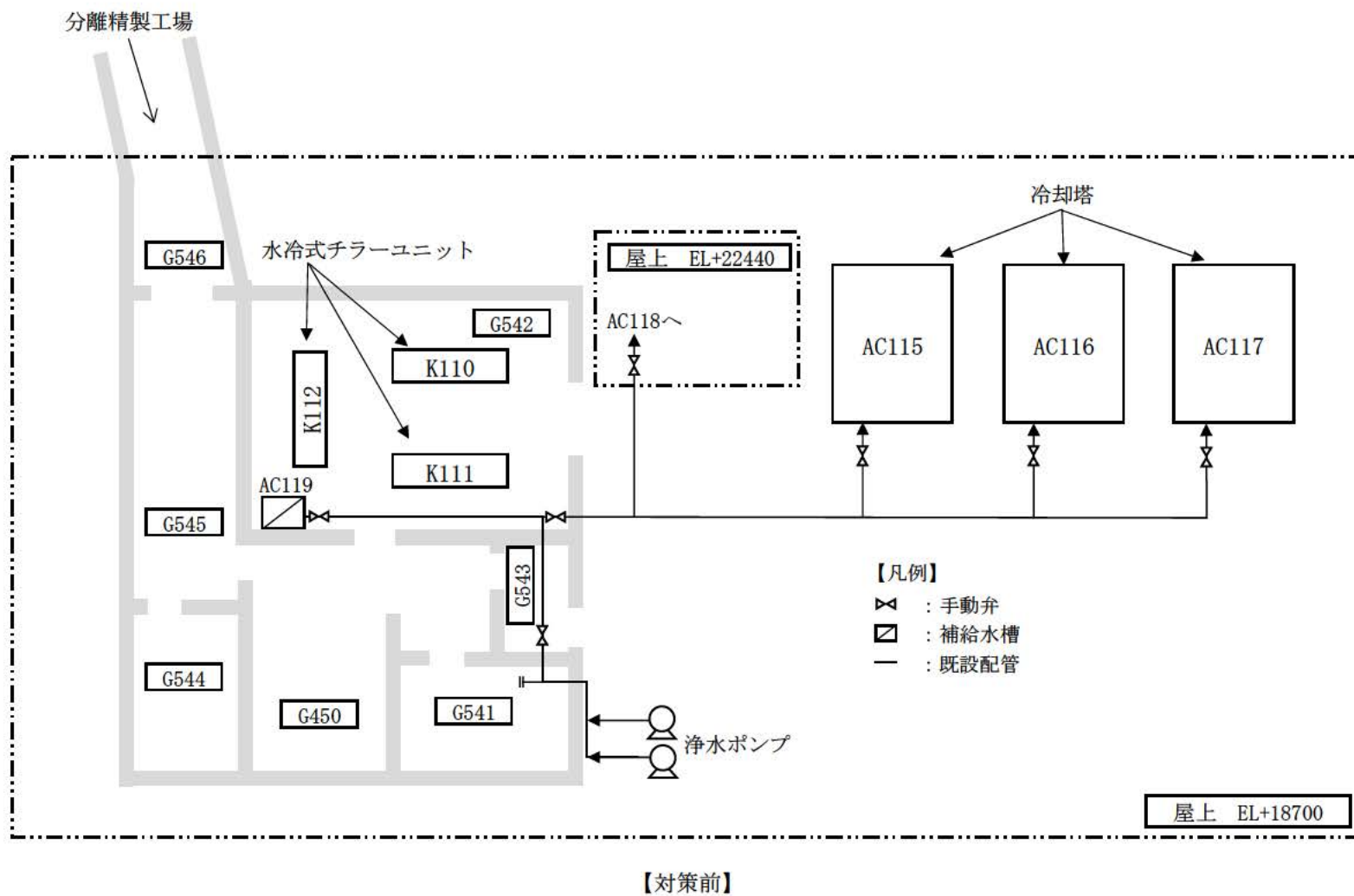
別図-2 浄水配管の一部改造に伴う配管系統概要図(1/2)
