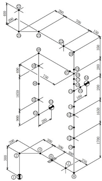
図-4-9 消火水配管 (KG99-005) の解析モデル (1/2)
