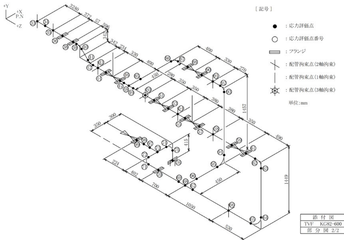
図-4-1 蒸気配管 (KG82-600) の解析モデル (2/2)
