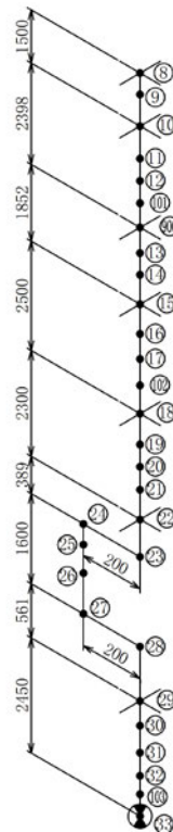
図-4-7 消火水配管 (KG85-604) の解析モデル (2/2)
