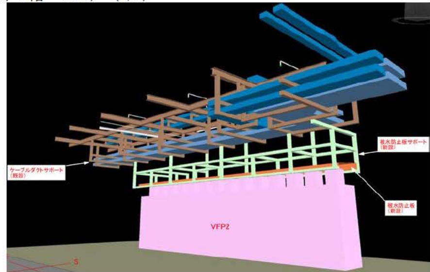
別図－8 被水防止板の概要（地下1階 VFP2）（2/6）
