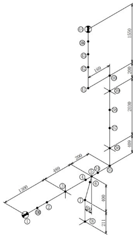
図-4-7 消火水配管 (KG85-604) の解析モデル (1/2)
