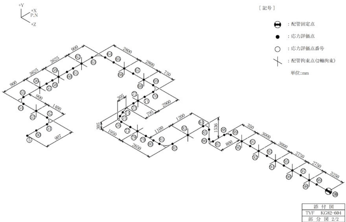
図-4-3 蒸気配管 (KG82-604) の解析モデル (2/2)
