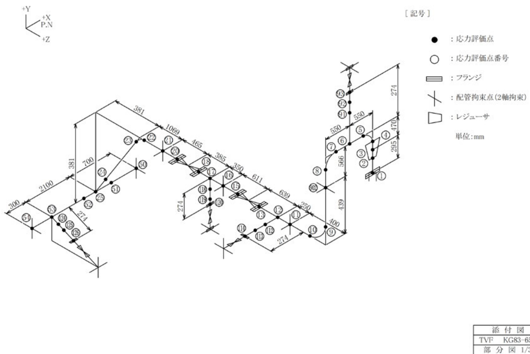
図-4-6 冷却水配管 (KG83-652) の解析モデル (1/3)
