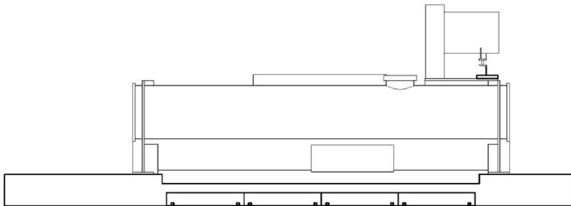
別図-13 オイルパン設置概略図 (冷凍機 G07CH02)
