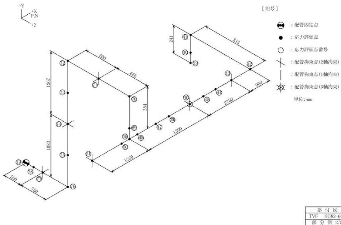
図-4-4 蒸気配管 (KG82-607) の解析モデル (2/5)
