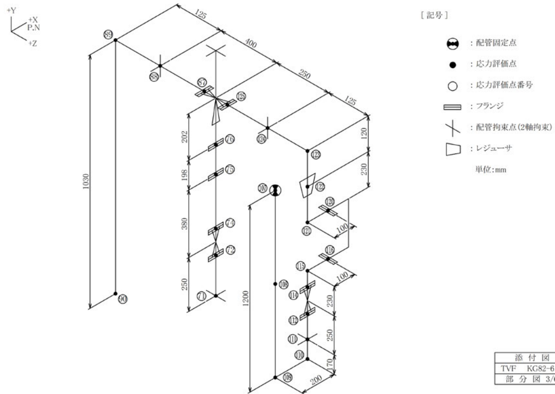
図-4-5 蒸気配管 (KG82-612) の解析モデル (3/6)
