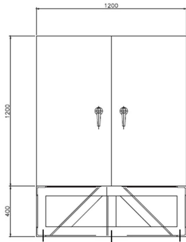
正面図
