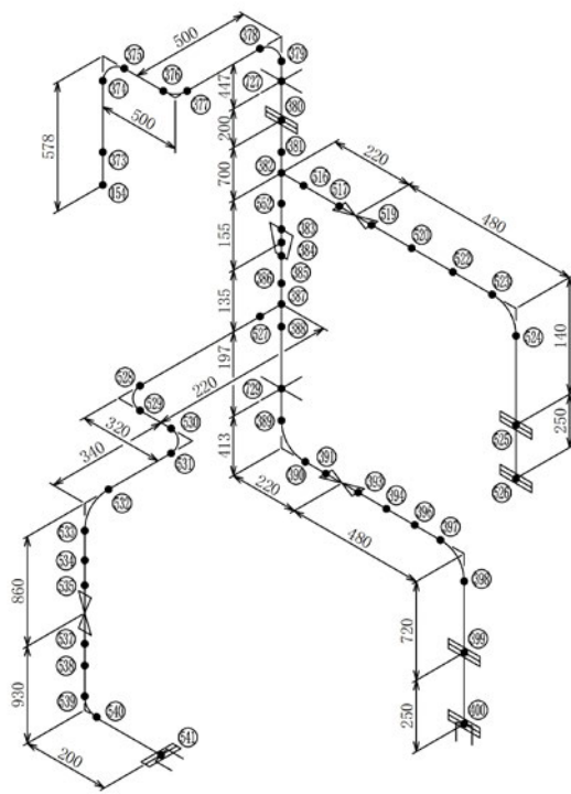
図-4-11 蒸気配管（空調設備）（KG99-013）の解析モデル（7/10）
