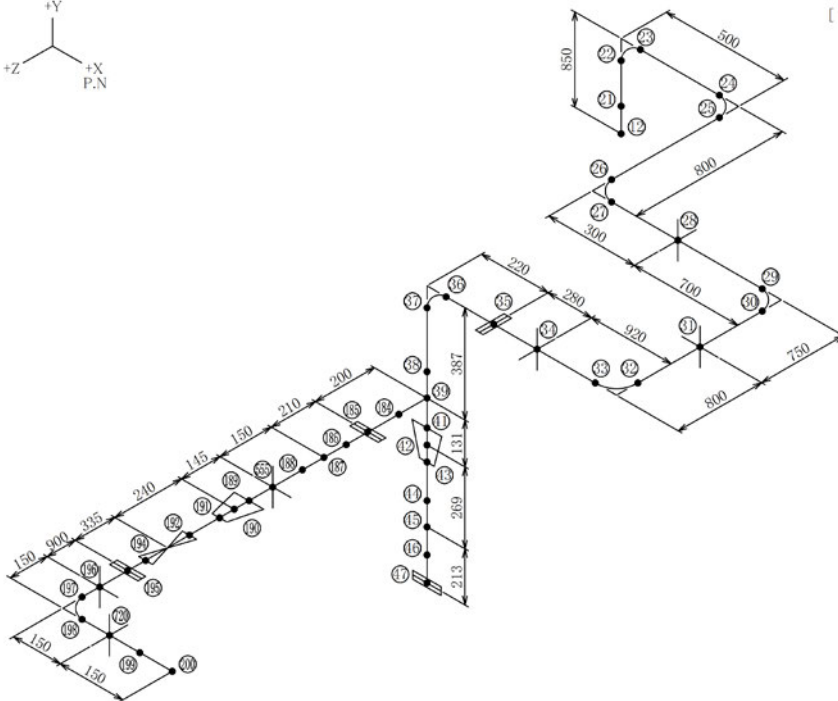
図-4-11 蒸気配管（空調設備）（KG99-013）の解析モデル（2/10）
