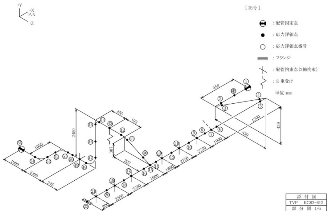
図-4-5 蒸気配管 (KG82-612) の解析モデル (1/6)
