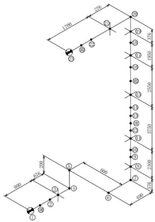
図-4-8 消火水配管 (KG85-621) の解析モデル
