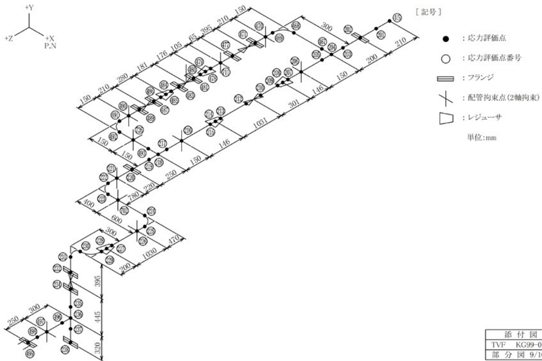
図-4-11 蒸気配管（空調設備）（KG99-013）の解析モデル（9/10）
