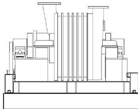
別図-11 オイルパン設置概略図 (排風機 G41K92)
