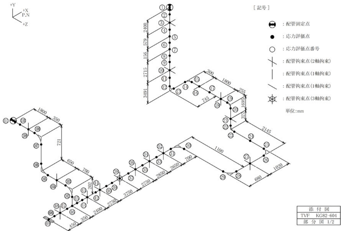
図-4-3 蒸気配管 (KG82-604) の解析モデル (1/2)
