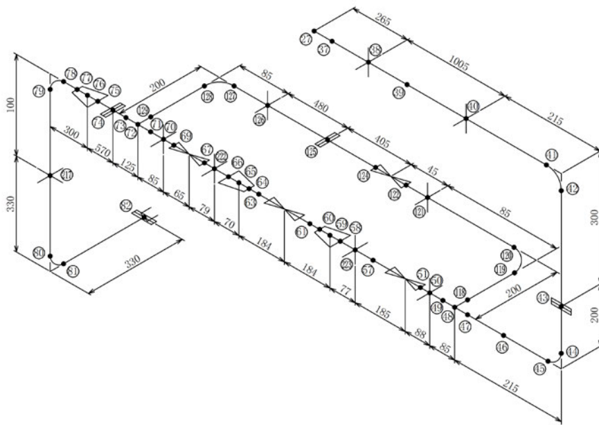
図-4-14 蒸気配管（空調設備）（KG99-018）の解析モデル（2/3）
