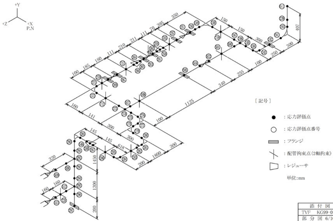
図-4-11 蒸気配管（空調設備）（KG99-013）の解析モデル（6/10）
