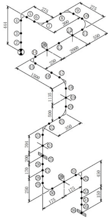
図-4-14 蒸気配管（空調設備）（KG99-018）の解析モデル（1/3）
