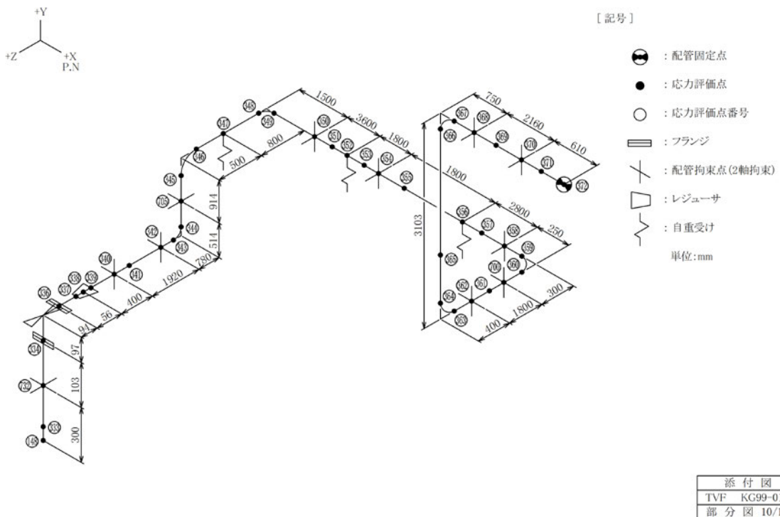
図-4-11 蒸気配管（空調設備）（KG99-013）の解析モデル（10/10）
