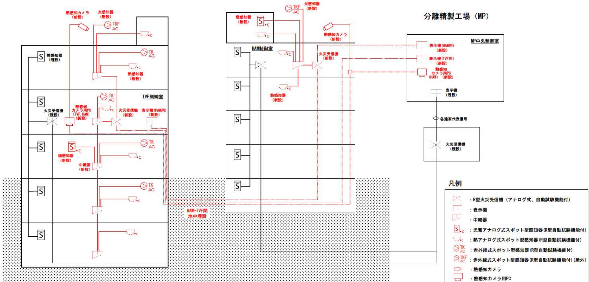
別図-15 火災感知設備のシステム構成の概要
