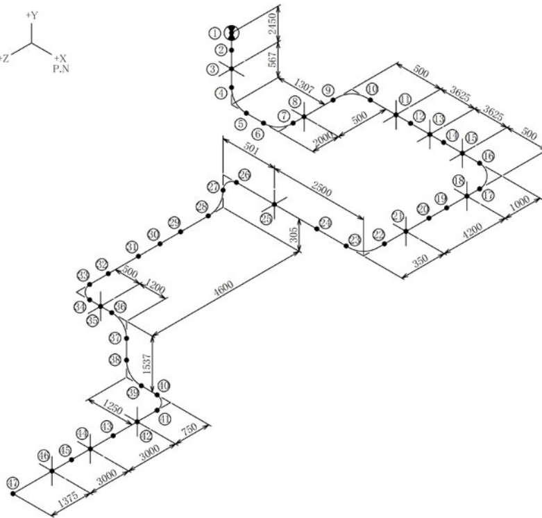
図-4-2 蒸気配管 (KG82-601) の解析モデル (1/2)
