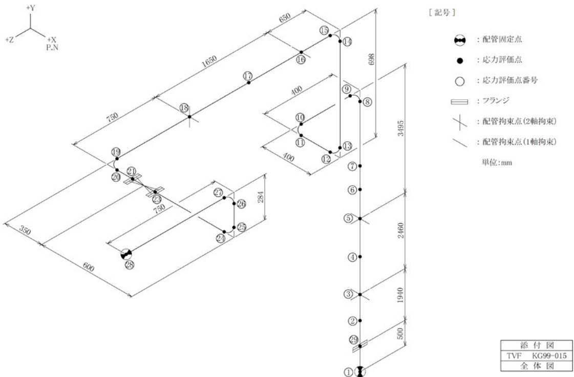
図-4-12 蒸気配管（空調設備）（KG99-015）の解析モデル
