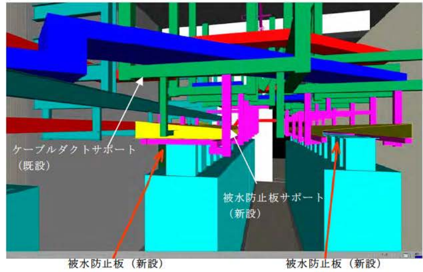
別図－8 被水防止板の概要（地下2階 VFP1）（1/6）
