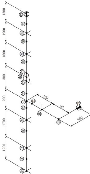
図-4-9 消火水配管 (KG99-005) の解析モデル (2/2)
