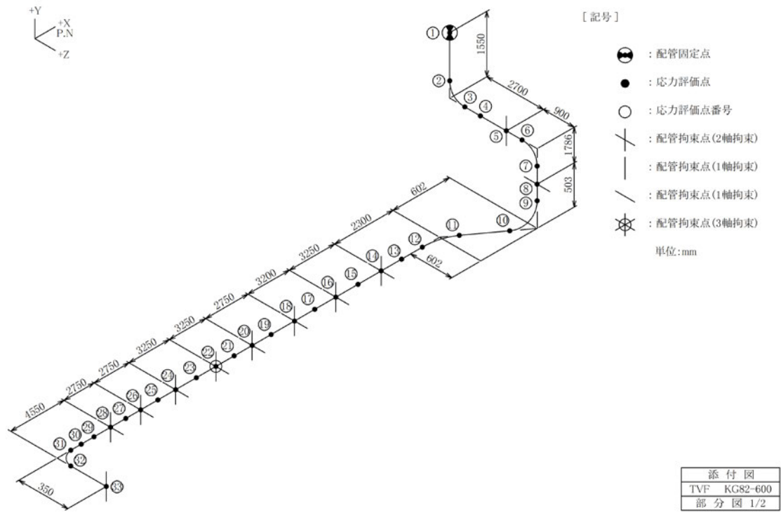
図-4-1 蒸気配管 (KG82-600) の解析モデル (1/2)
