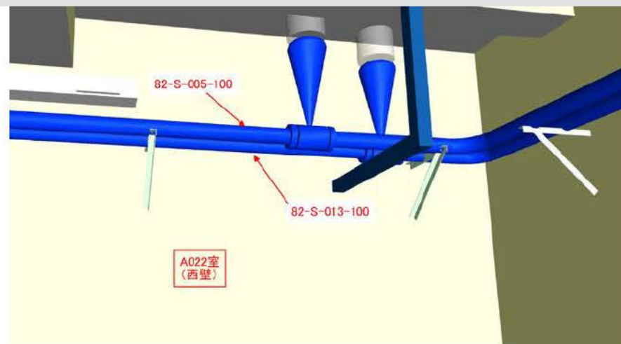
別図－10 蒸気遮断弁の設置の概要
