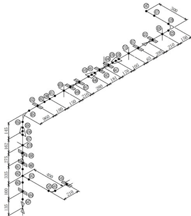
図-4-11 蒸気配管（空調設備）（KG99-013）の解析モデル（8/10）
