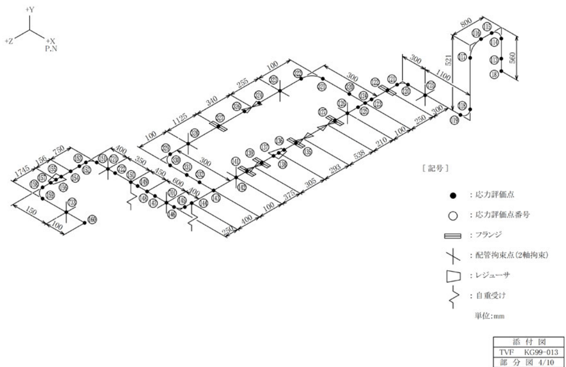
図-4-11 蒸気配管（空調設備）（KG99-013）の解析モデル（4/10）
