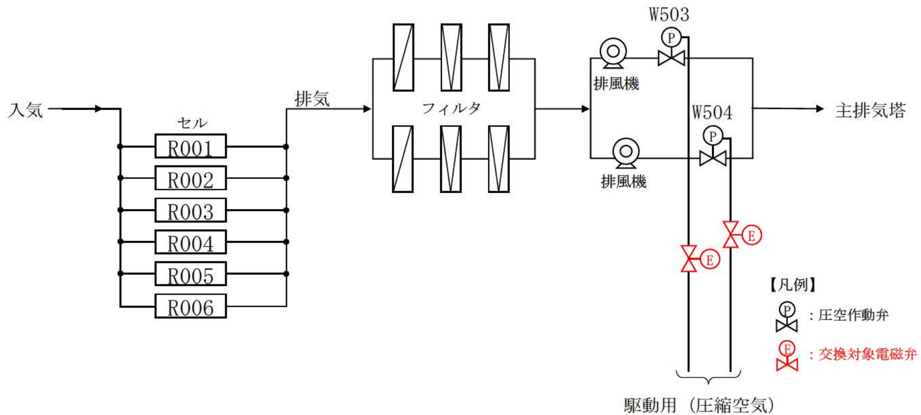
別図-8 電磁弁の更新の概要図
