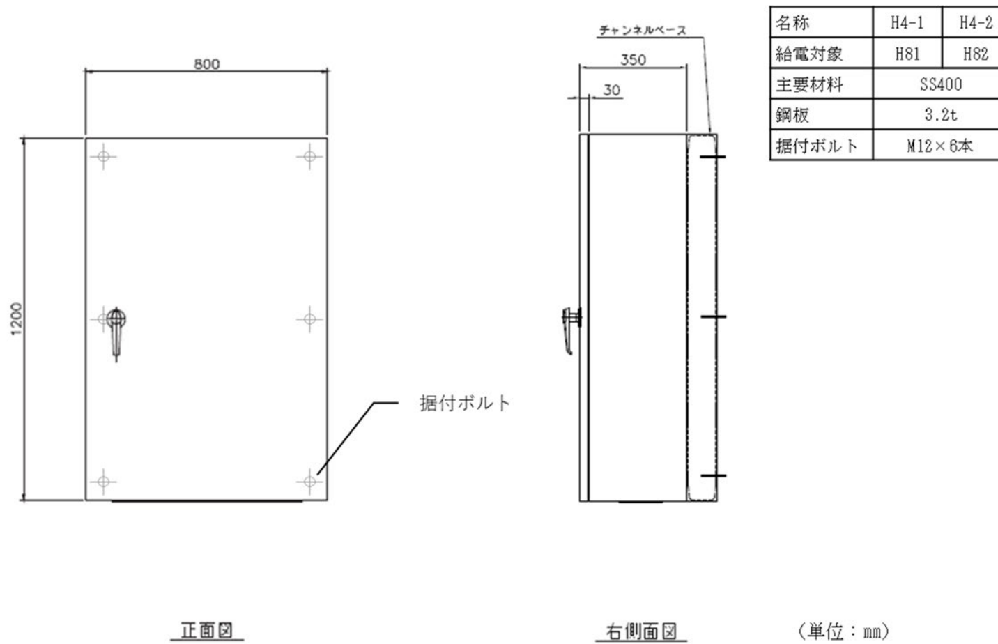
別図-7 電源切替盤の概要 (4/7)
