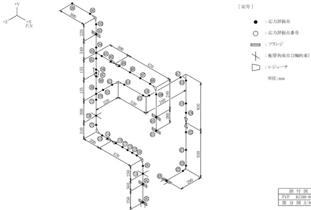
図-4-11 蒸気配管（空調設備）（KG99-013）の解析モデル（5/10）
