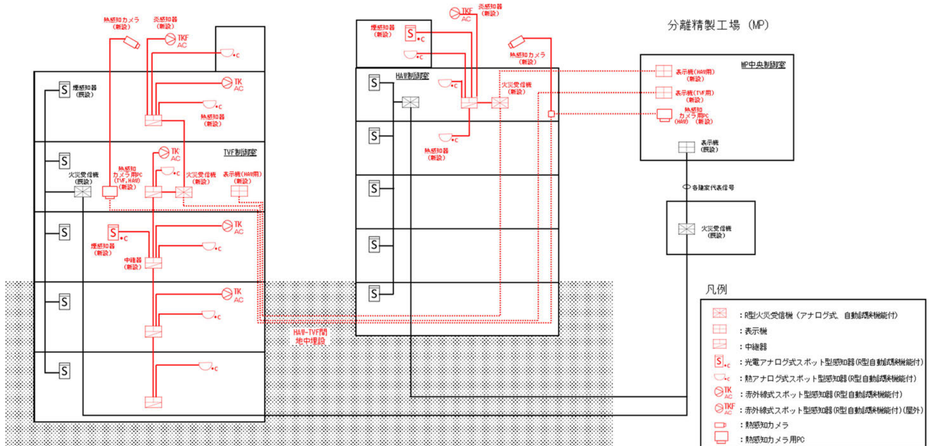
別図-3 火災感知設備のシステム構成の概要
