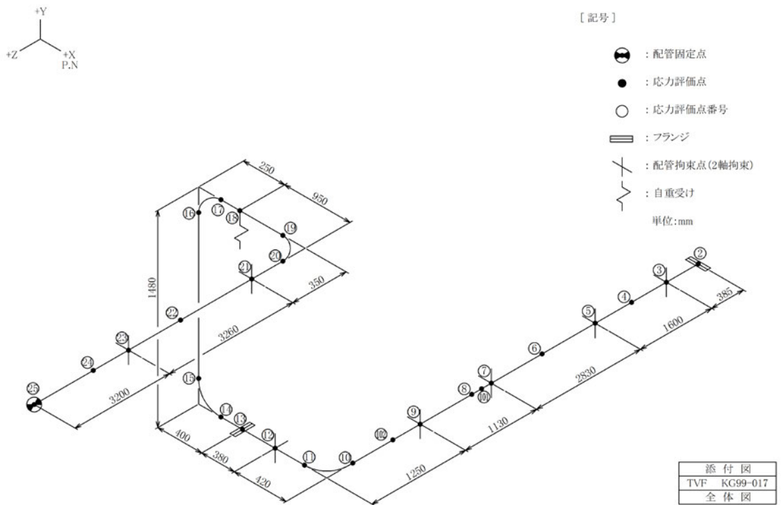
図-4-13 蒸気配管（空調設備）（KG99-017）の解析モデル
