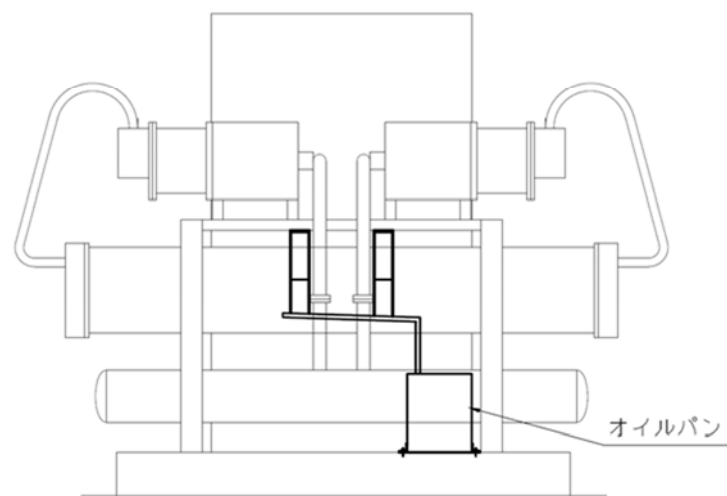
別図-2 オイルパン設置概略図 (冷凍機)
