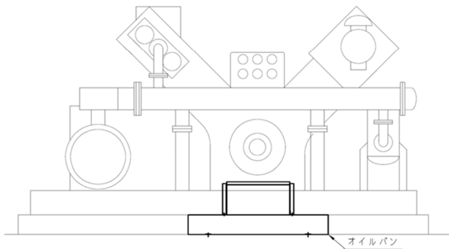
別図-1 オイルパン設置概略図 (空気圧縮機)
