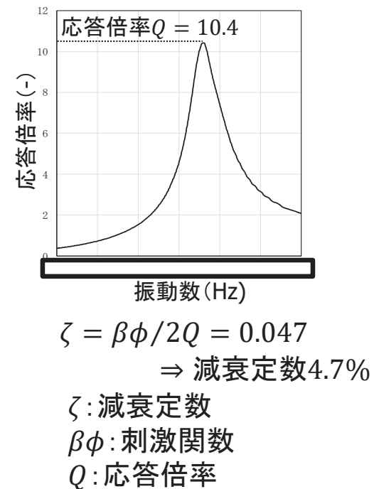
減衰定数 \zeta の算出例
