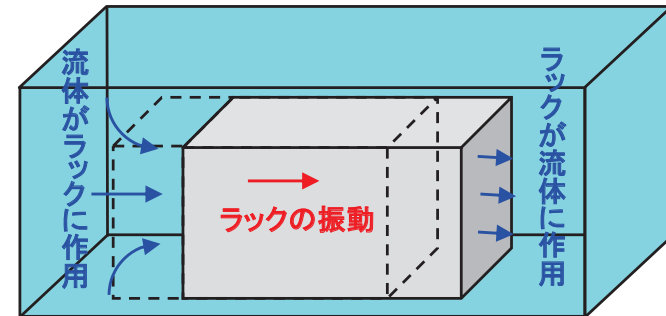
流体－構造連成による応答低減効果
