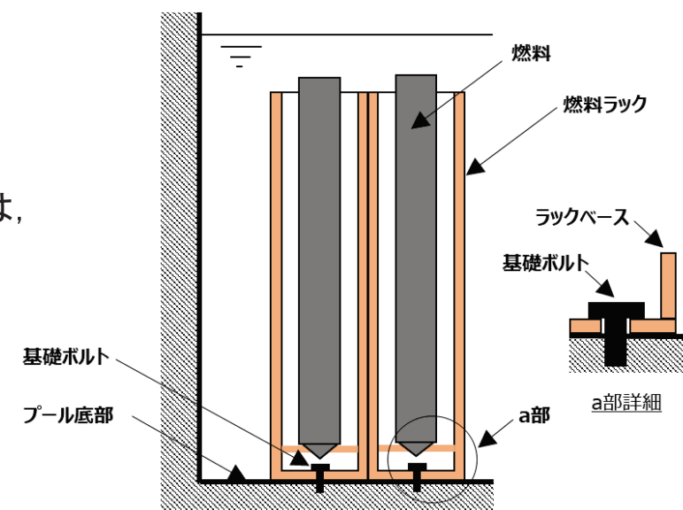
燃料ラック概略構造
