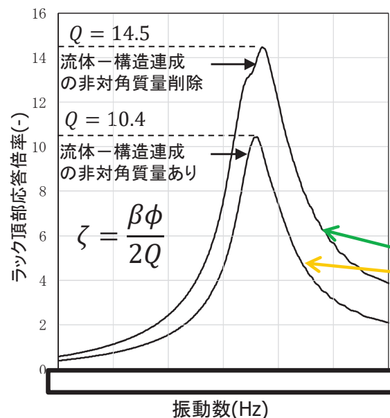
ラック頂部の応答倍率比較
