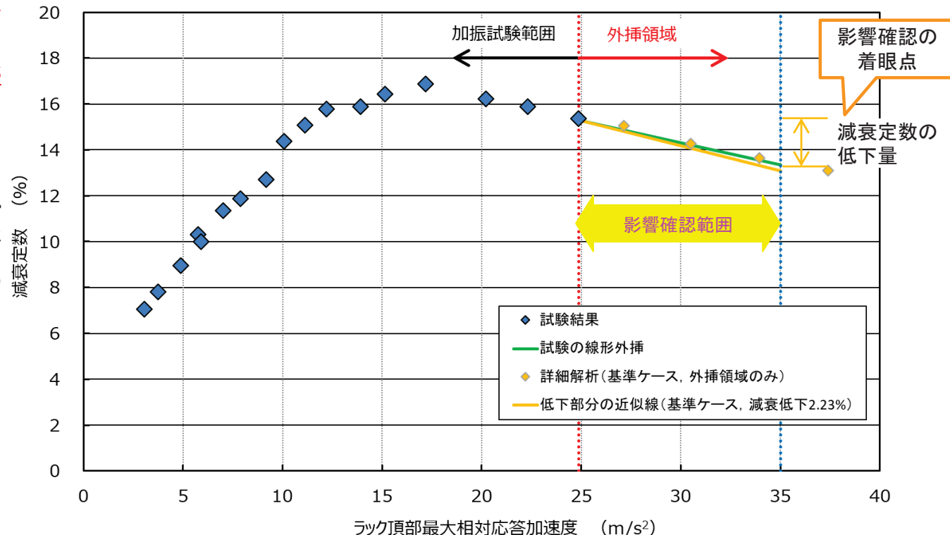
減衰定数-応答加速度の関係(外挿領域における減衰定数の低下量)
