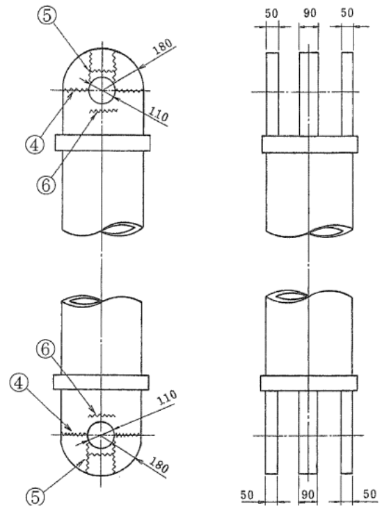
(c) サポートパイプ側ヒンジ (単位：mm)
