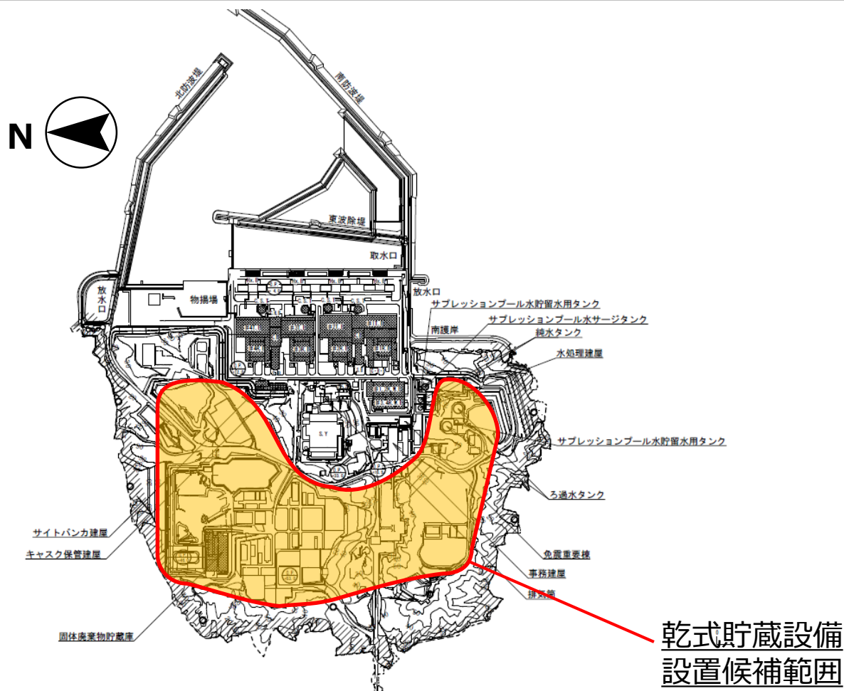
福島第二原子力発電所敷地図
