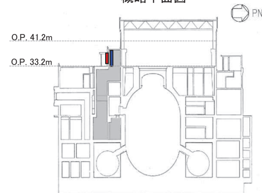
原子炉建屋原子炉棟断面図
