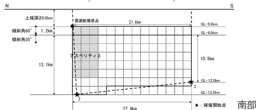
（展開図）
