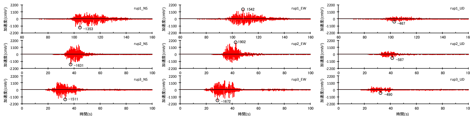
(アスぺリティ面積比22%、平均応力降下量3.1MPaで設定した震源モデル（地震動の顕著な増幅を考慮）を用いた場合)
