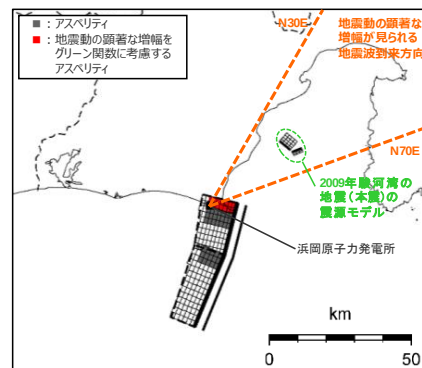
内陸地殻内地震（御前崎海溝西部の断層帯による地震）
