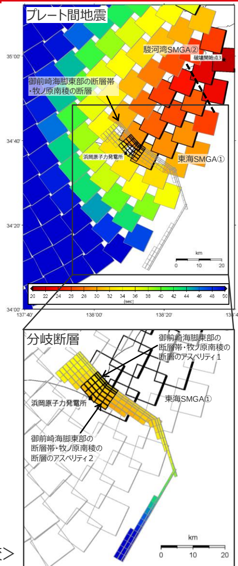
<S波到達時刻のアイソクロン>
