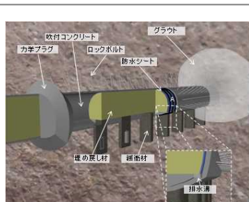
HLW 縦置き・ブロック方式
