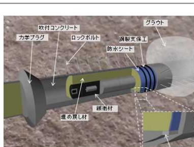
HLW 横置き・PEM方式
