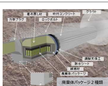
TRU等廃棄物 (緩衝材有り)
