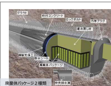
TRU等廃棄物 (緩衝材無し)
