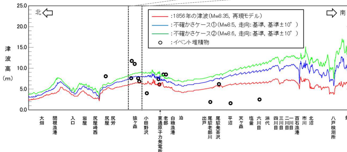
汀線位置における想定津波群(空間格子間隔278m※2)とイベント堆積物の比較
