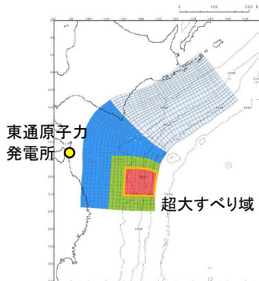
基準断層モデル② (特性化モデル③, 南へ約100km移動)
