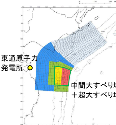
基準断層モデル③ (特性化モデル④, 南へ約40km移動)
