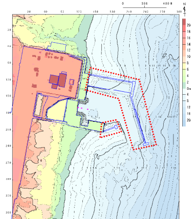
防波堤無し
