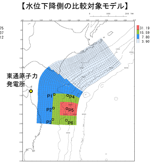
基準断層モデル ②
