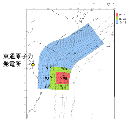
基準断層モデル①
