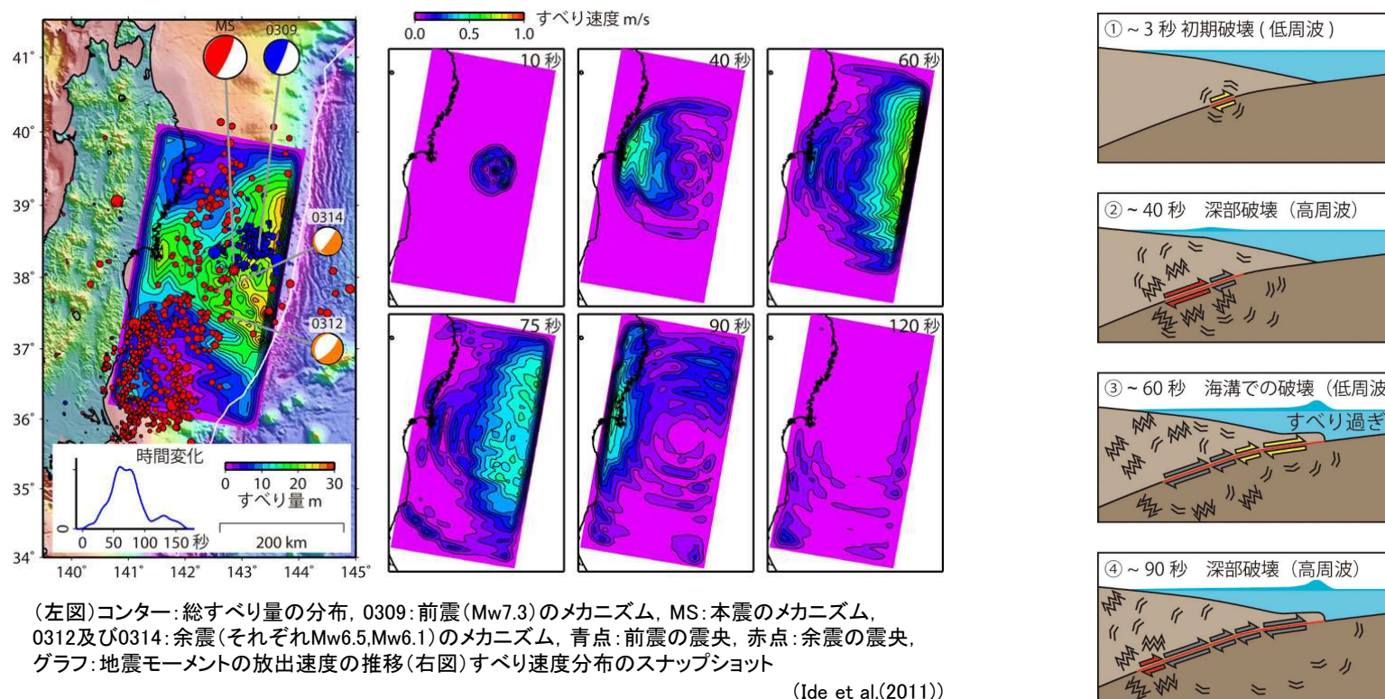
時間毎の破壊過程の模式図(井出(2011))
