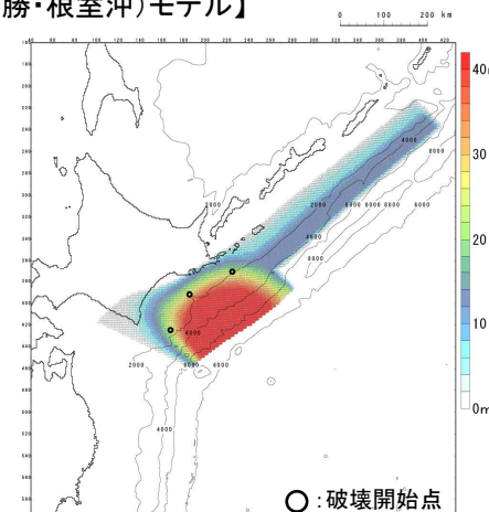
すべり量分布(合計)及び破壊開始点位置※2
