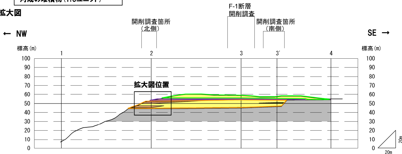
C' 断面図
