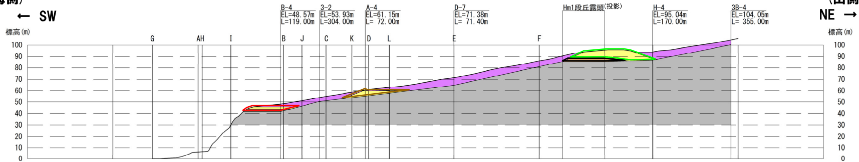
⑨断面図
