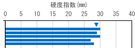
硬度測定結果 (測線:Ts2-1)
