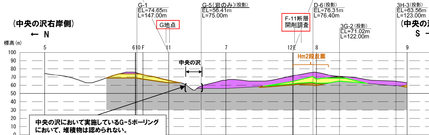
L断面図
