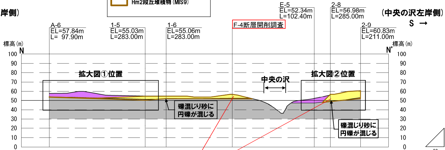
N断面図
