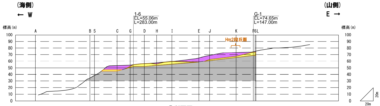
⑩断面図
