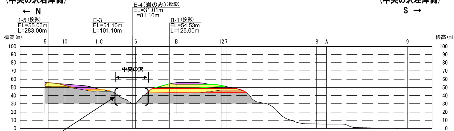
G断面図
