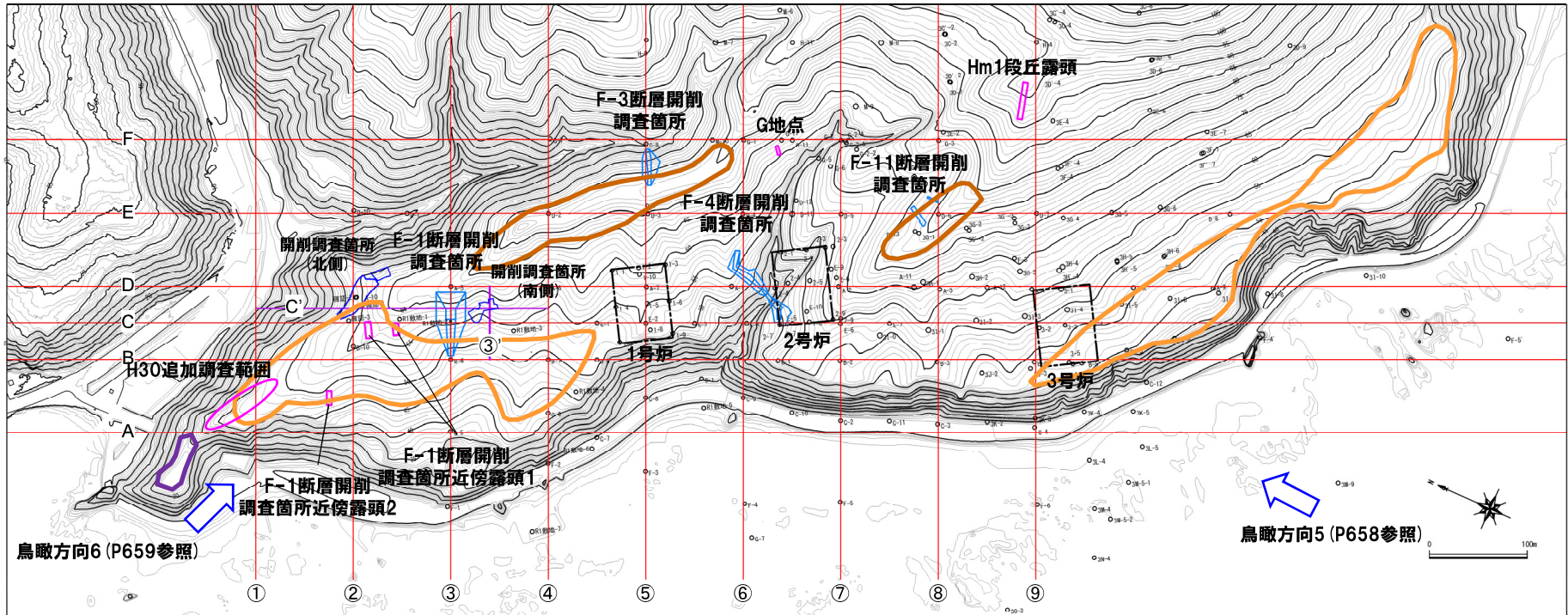
敷地平面図
