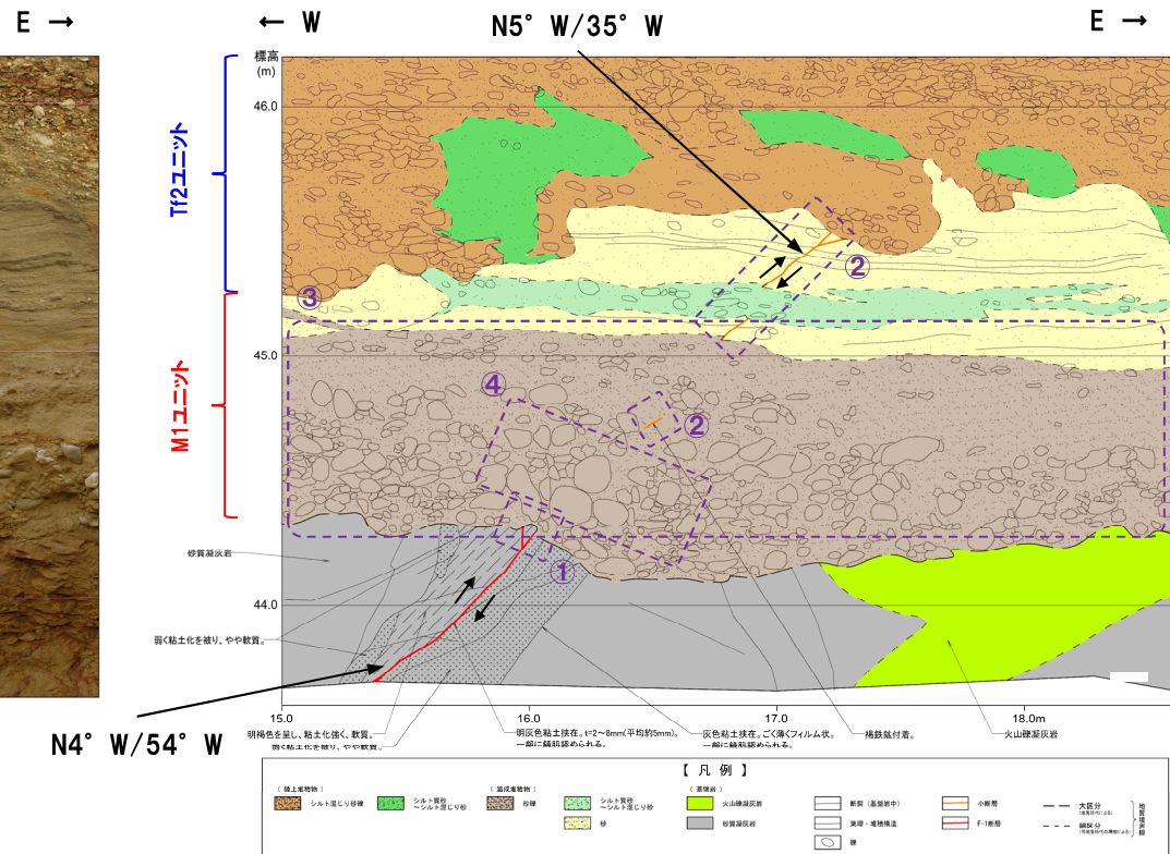
開削調査箇所(北側)北側壁面 F-1断層付近 詳細スケッチ
