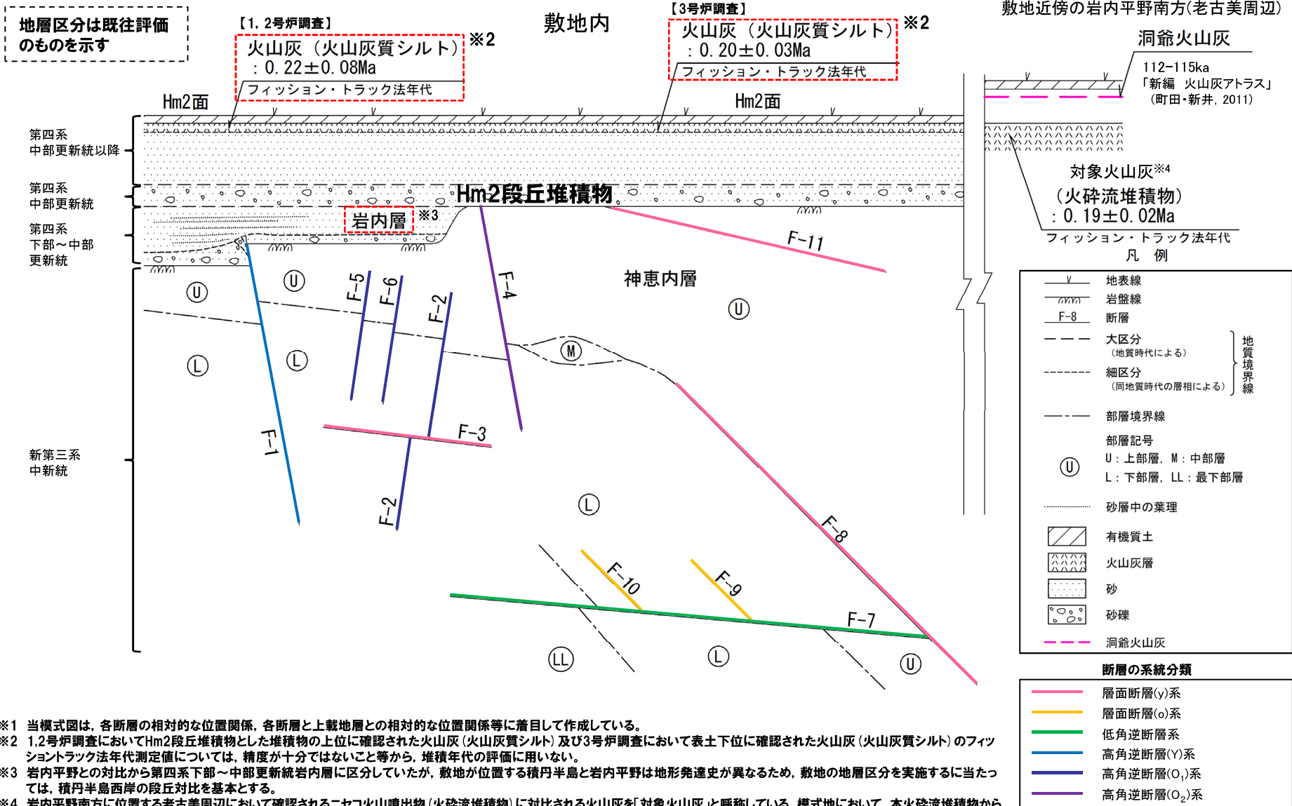
(参考) 敷地に認められる断層模式図 (既往評価)
