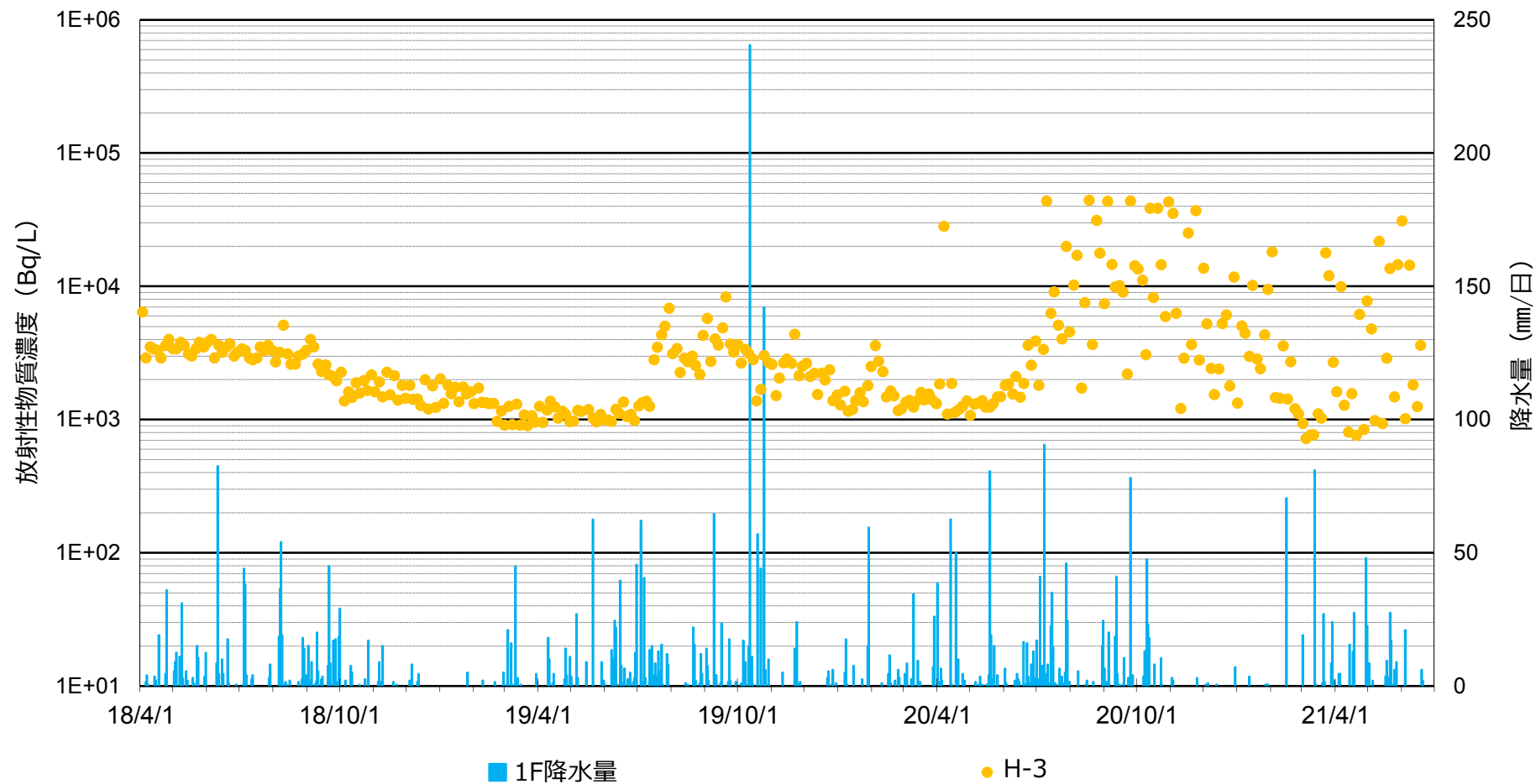
1,2号機取水口間地下水放射性物質濃度と降水量の推移 観測孔No.1-14
