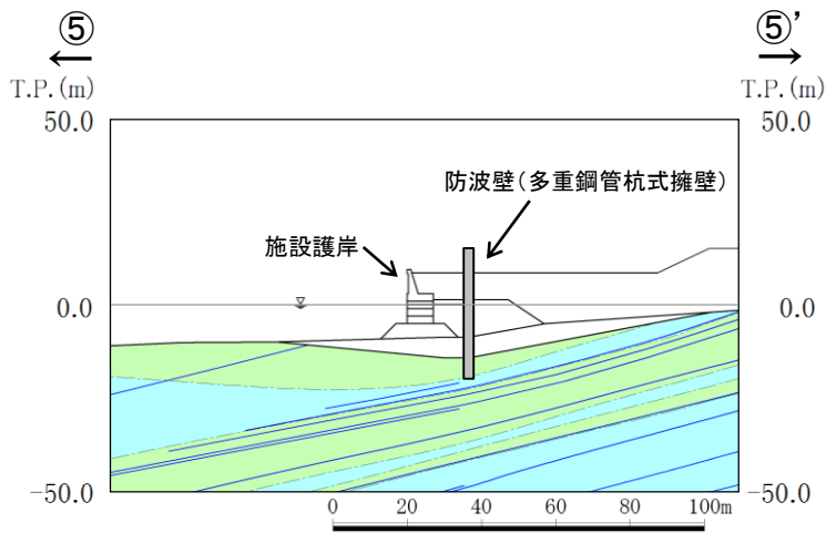
⑤-⑤' 断面図
