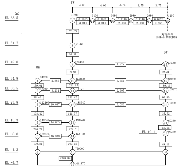
鉛直モデル
