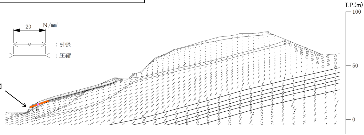
主応力分布図
