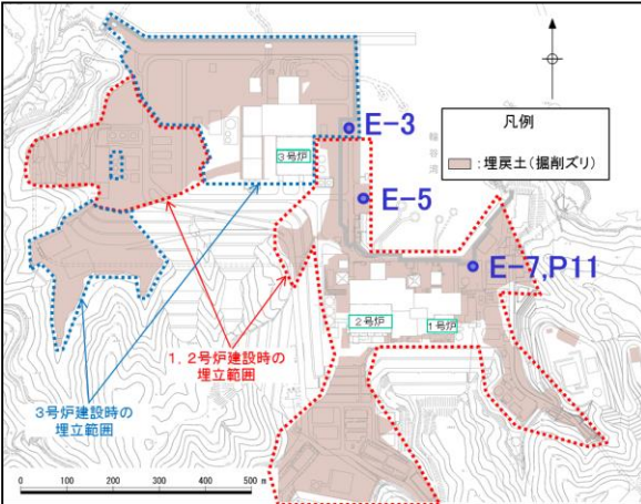
敷地平面図
