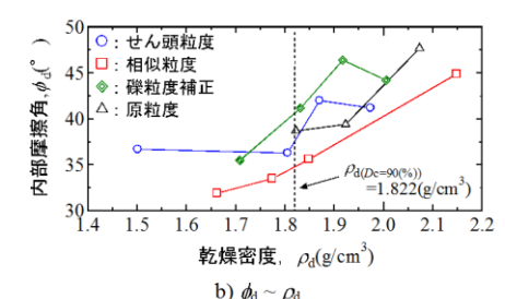
図9 内部摩擦角～締固め度, 乾燥密度の関係 (甲山試料)
