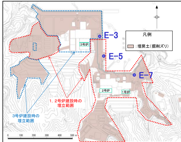
敷地平面図
