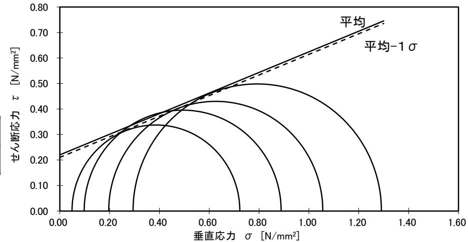
大型三軸圧縮試験結果(破壊包絡線)
