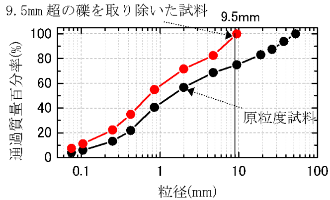
図1 実験試料の粒度分布
