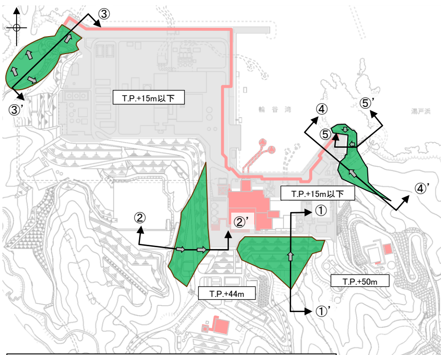
2号炉南側切取斜面(①-①'断面, 岩級・シーム)
