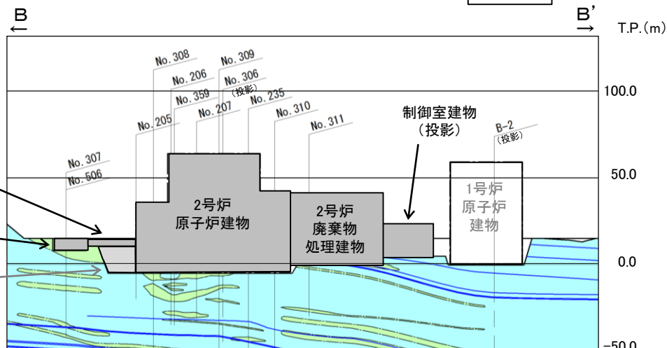
地質断面図(B-B'断面, 岩級・シーム)
