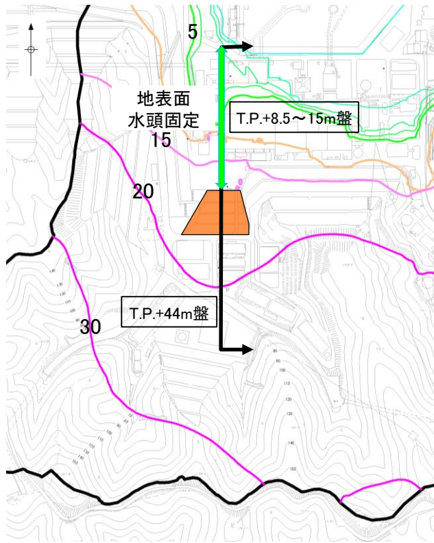
2号炉南側盛土斜面周辺の地形図 (3次元浸透流解析結果)
