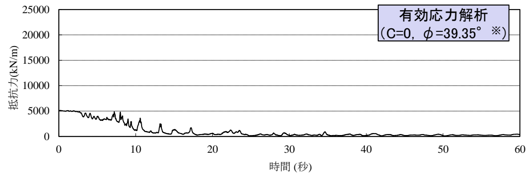
有効応力解析における液状化範囲内のすべり面上の抵抗力(S s -D(-, +)) ※FLIPのせん断強度、「防波壁の構造成立性」の審査において設定した値(P312参照)
