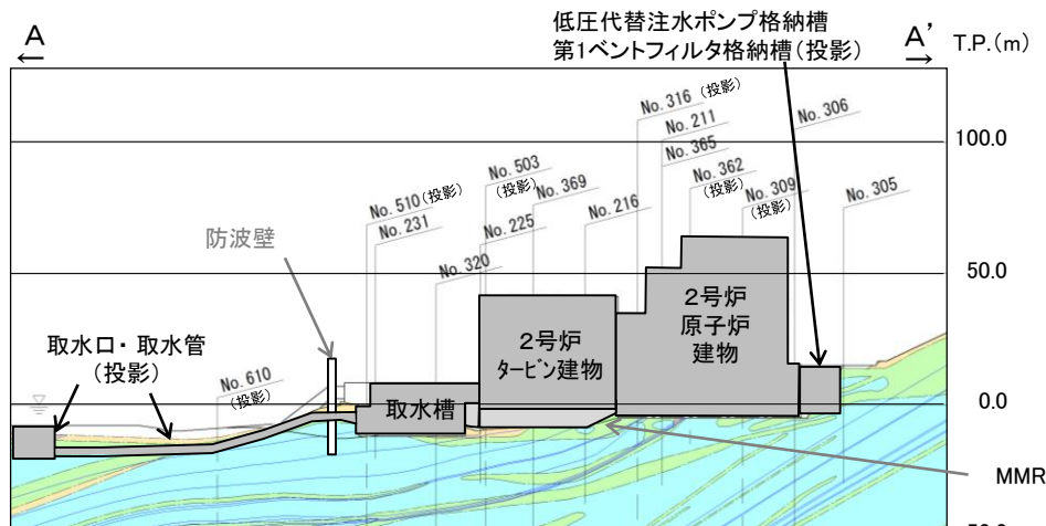
地質断面図(A-A'断面, 岩級・シーム)
