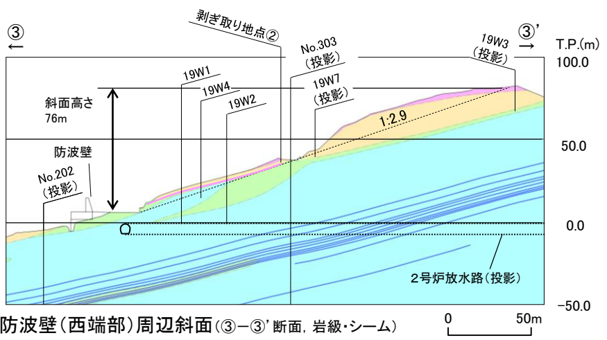
防波壁(西端部)周辺斜面(③-③'断面, 岩級・シーム)
