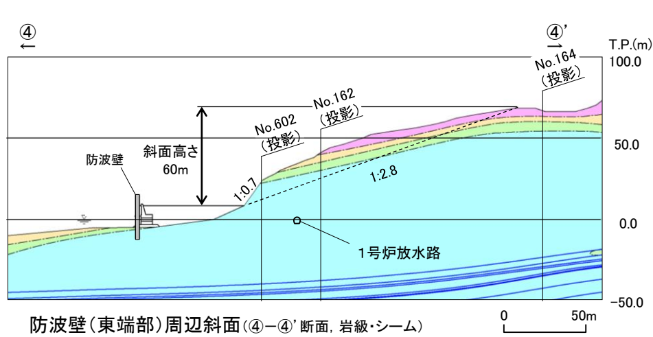
防波壁(東端部)周辺斜面(④-④'断面, 岩級・シーム)
