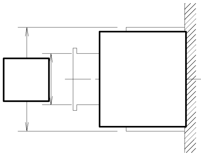
(b) 上部トラニオン (0° -180° 側)
