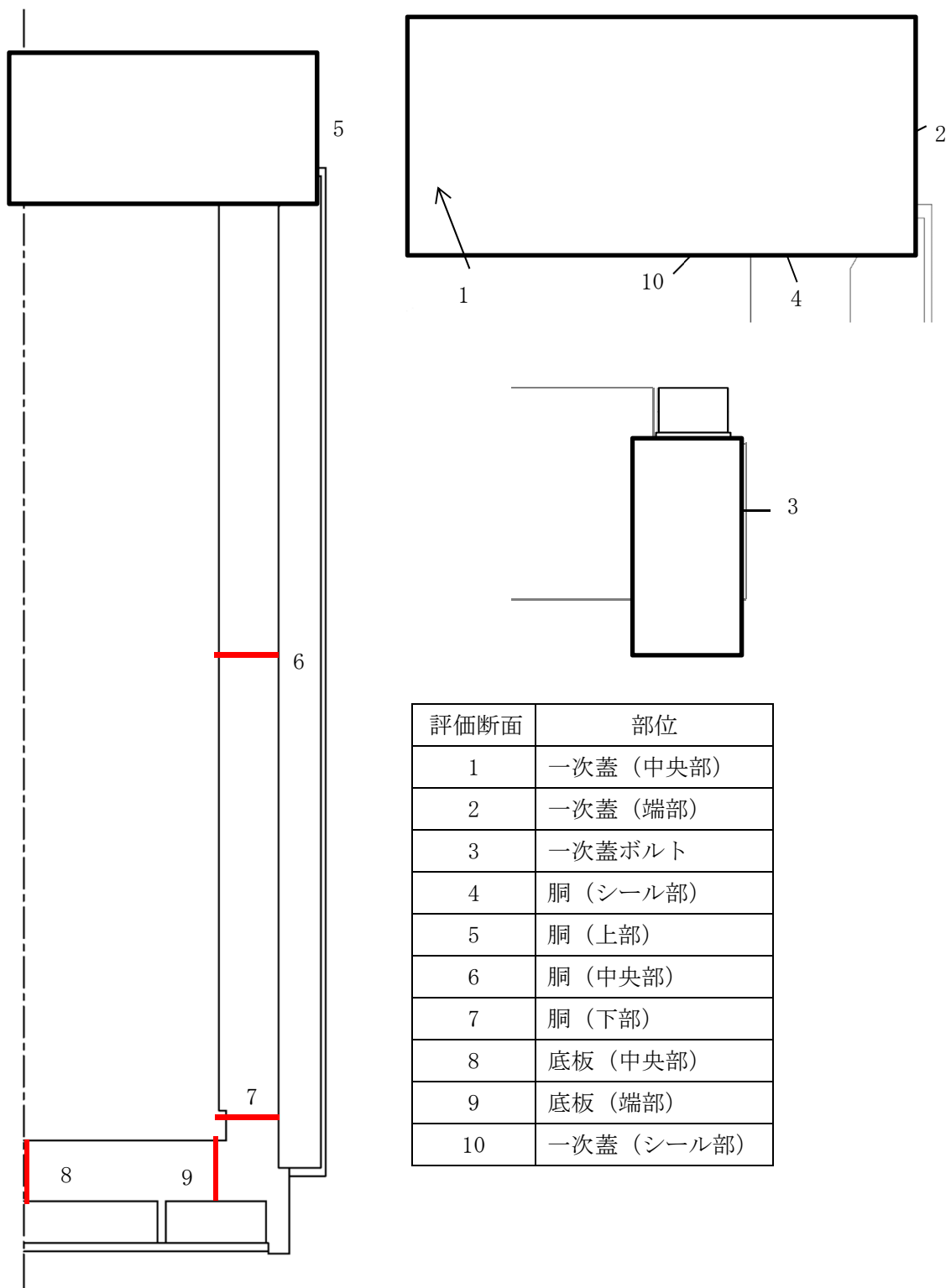
第3図 密封容器の応力評価位置
