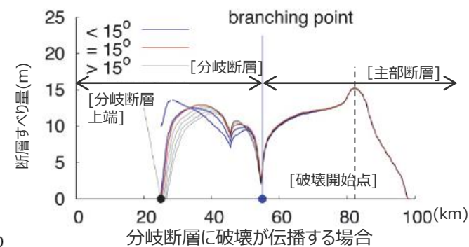
プレート境界面浅部に破壊が伝播する場合
