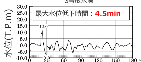
3号取水塔
