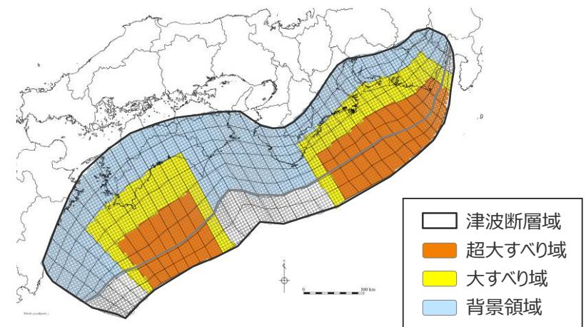
検討波源モデルC（土木学会(2016)手法） の大すべり域の位置を基準位置としたケース
