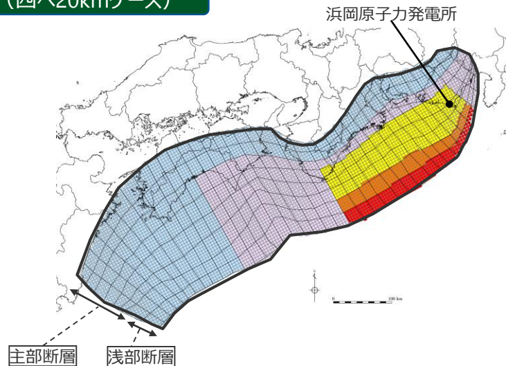
検討波源モデル③ (日本海溝の津波評価手法③) の大すべり域の位置を西へ20kmとしたケース
