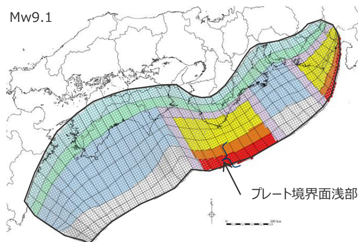
検討波源モデルA（プレート境界面浅部） （敷地に近い大すべり域の位置を東へ40km、大すべり域間の距離を100kmとしたケース）
