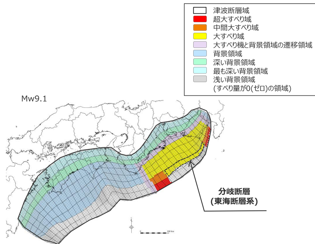
検討波源モデルB-1（プレート境界面浅部・東海断層系） （大すべり域の位置を東へ10kmとしたケース）
