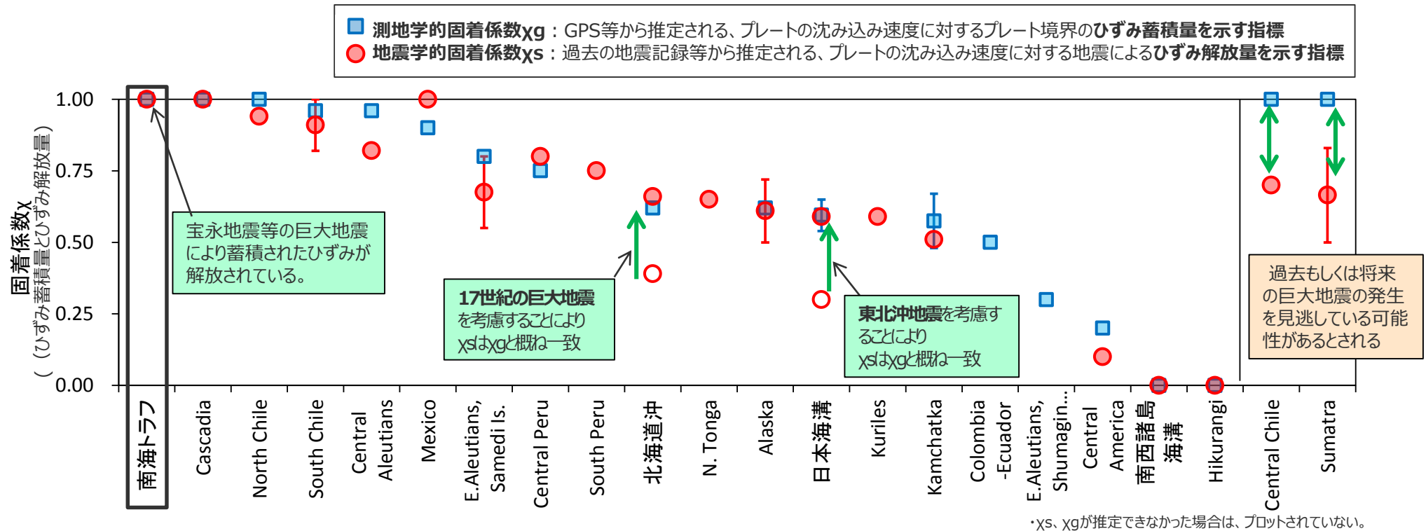
Scholz and Campos(2012)による世界の沈み込み帯のひずみ蓄積・解放の収支
