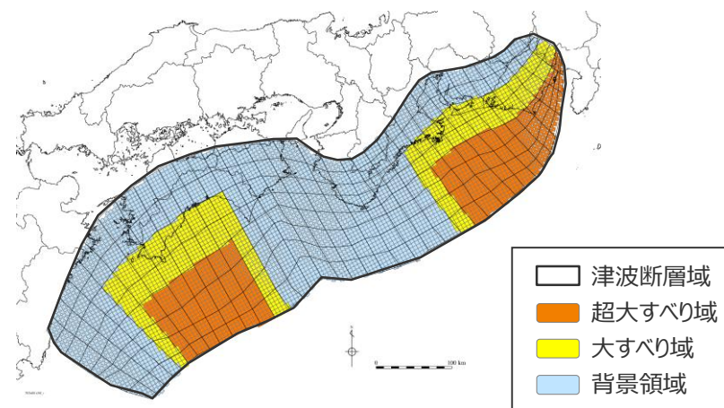
検討波源モデル①（日本海溝の津波評価手法①） の大すべり域の位置を東へ60kmとしたケース
