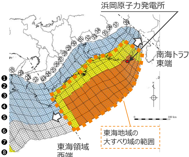
各小断層の配列 (検討波源モデルCの例)
