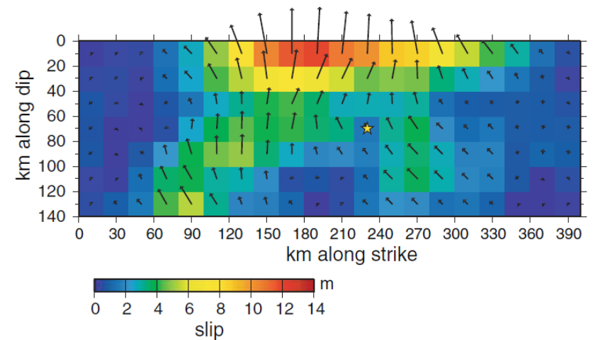
Baba et al.(2009)による波源モデル
