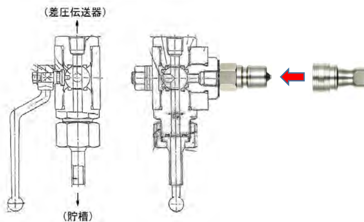
図3 既設三方弁へのカプラによる接続（イメージ）
