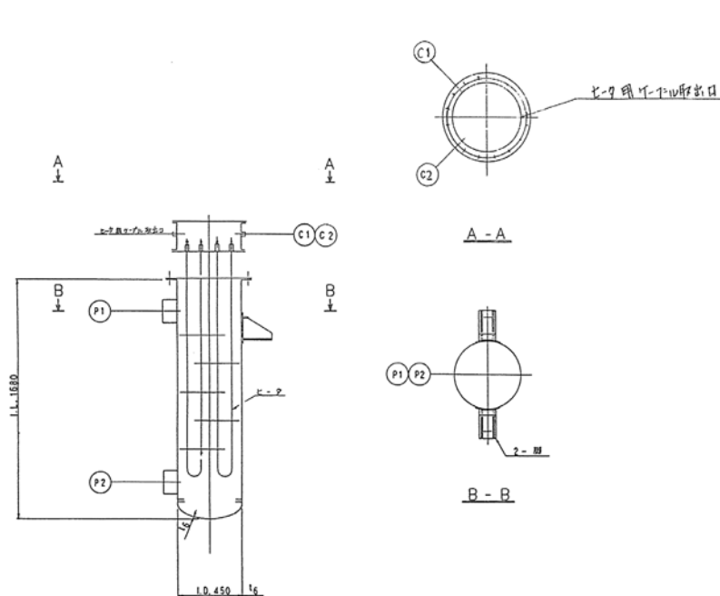
図 4 加熱器 (G41H84/H85) の概要図
