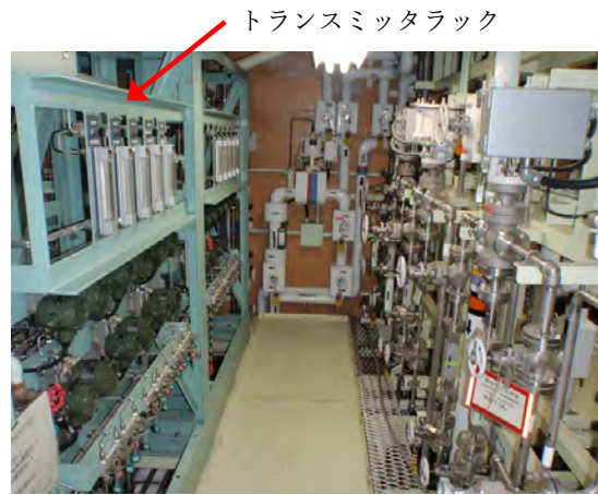
図-2 配管分岐室におけるトランスミッタラック等の設置状況
