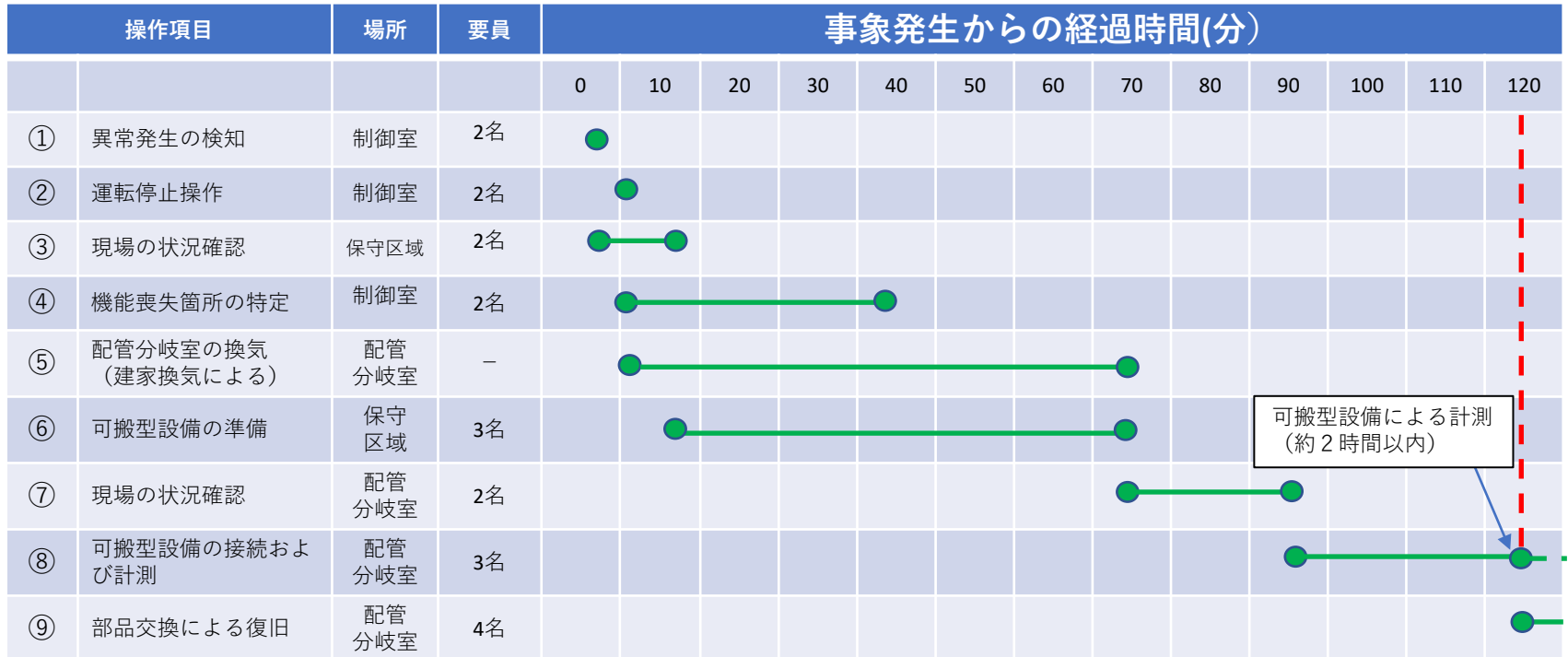
図5 可搬型設備による貯槽液位等の計測（タイムチャート）
