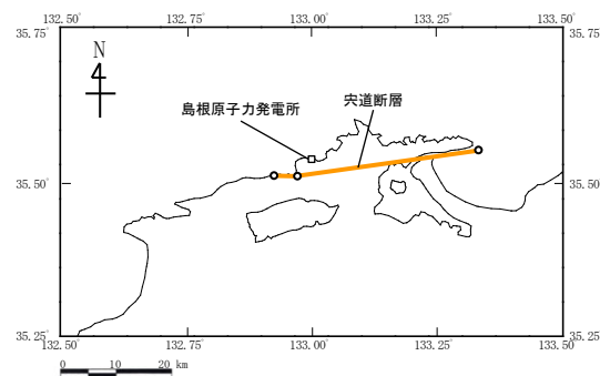
断層位置図
