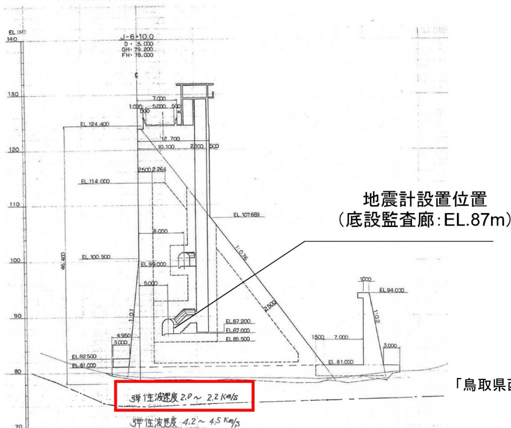
ダム断面図
