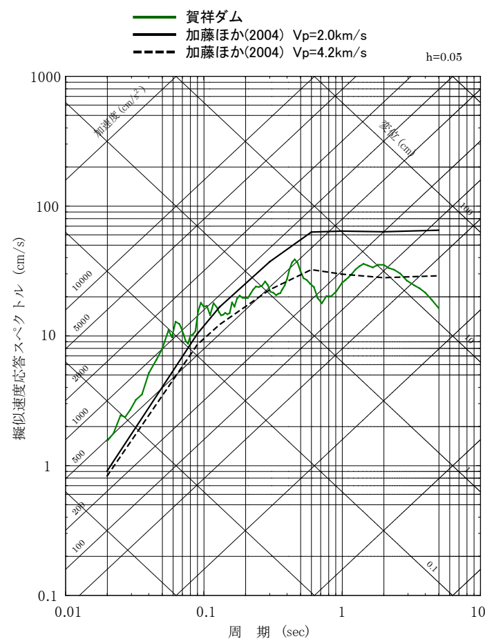
鉛直方向
