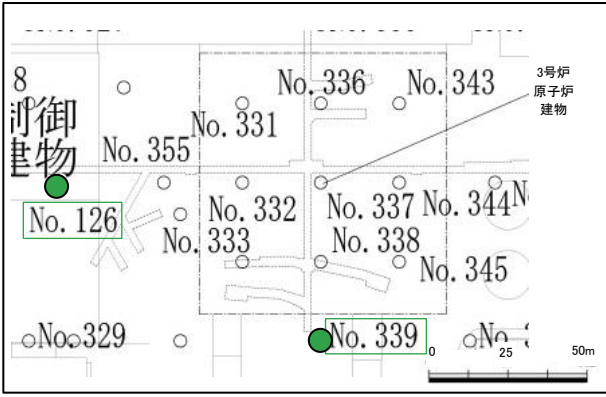
シーム及び周辺母岩のX線回折分析試料採取位置図
