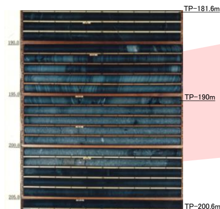
No.215コア写真
