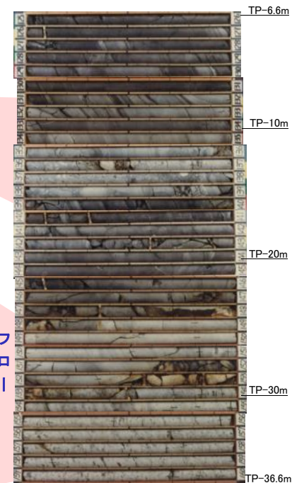
No.333コア写真
