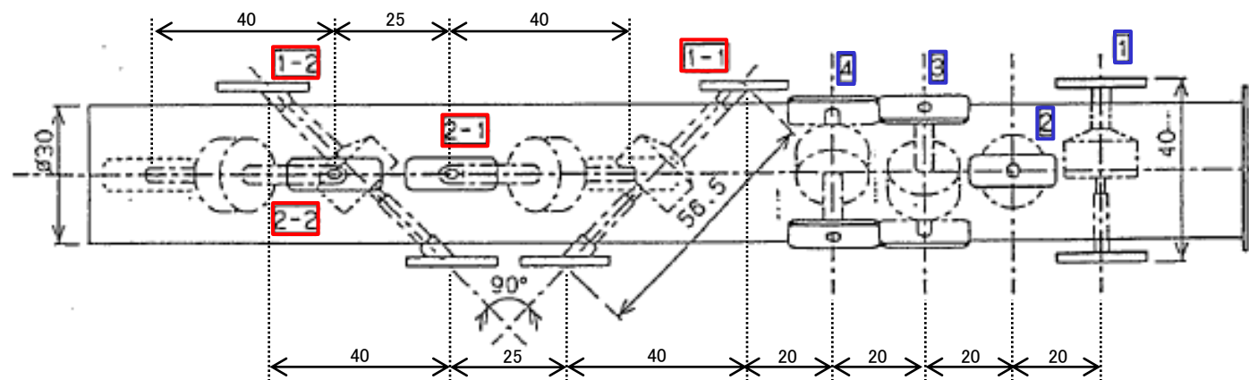
ひずみ計設置 側面透視図
