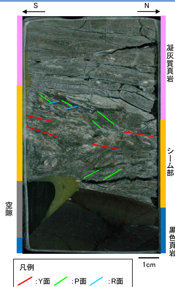
B23シーム研磨片写真
