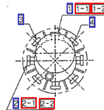
ひずみ計設置 正面図
