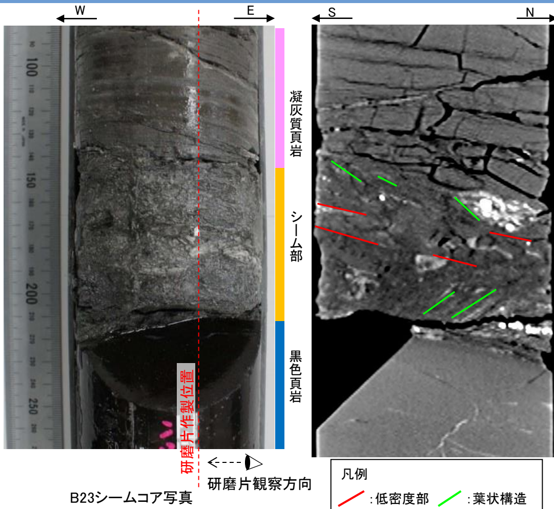
B23シームCT画像(研磨片作製断面)
