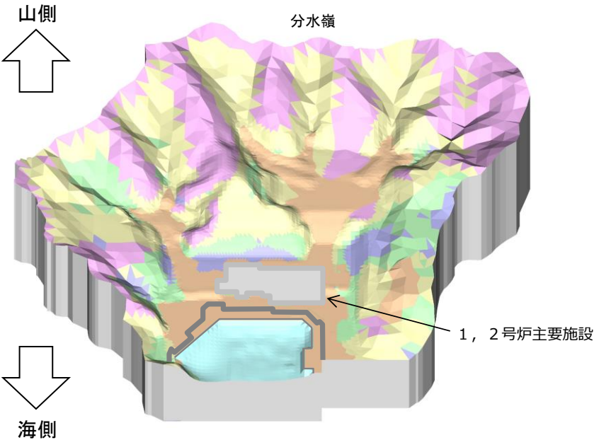
1, 2号炉エリア 解析モデル
