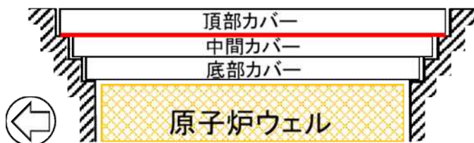
シールドプラグ (断面構造)
