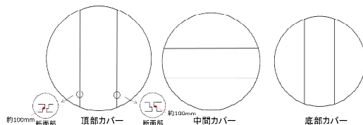
シールドプラグ (平面構造)
