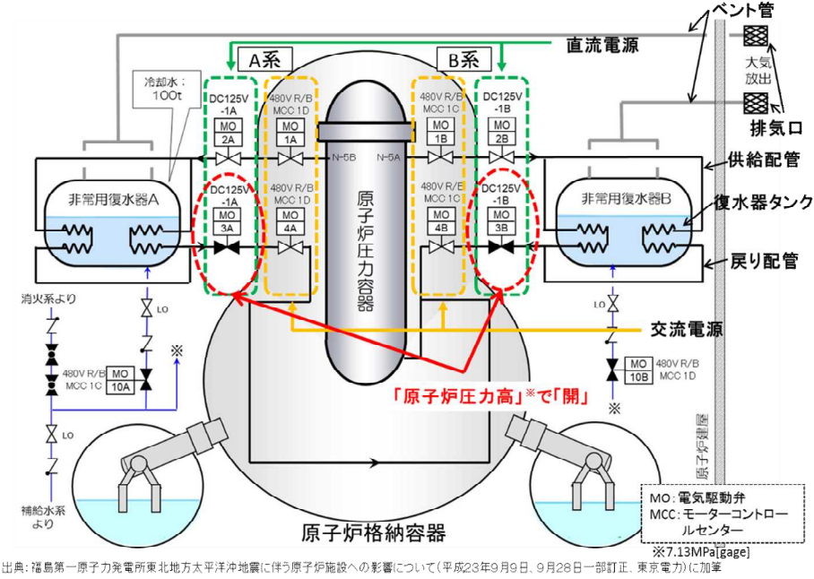
1号機非常用復水器の系統概要
