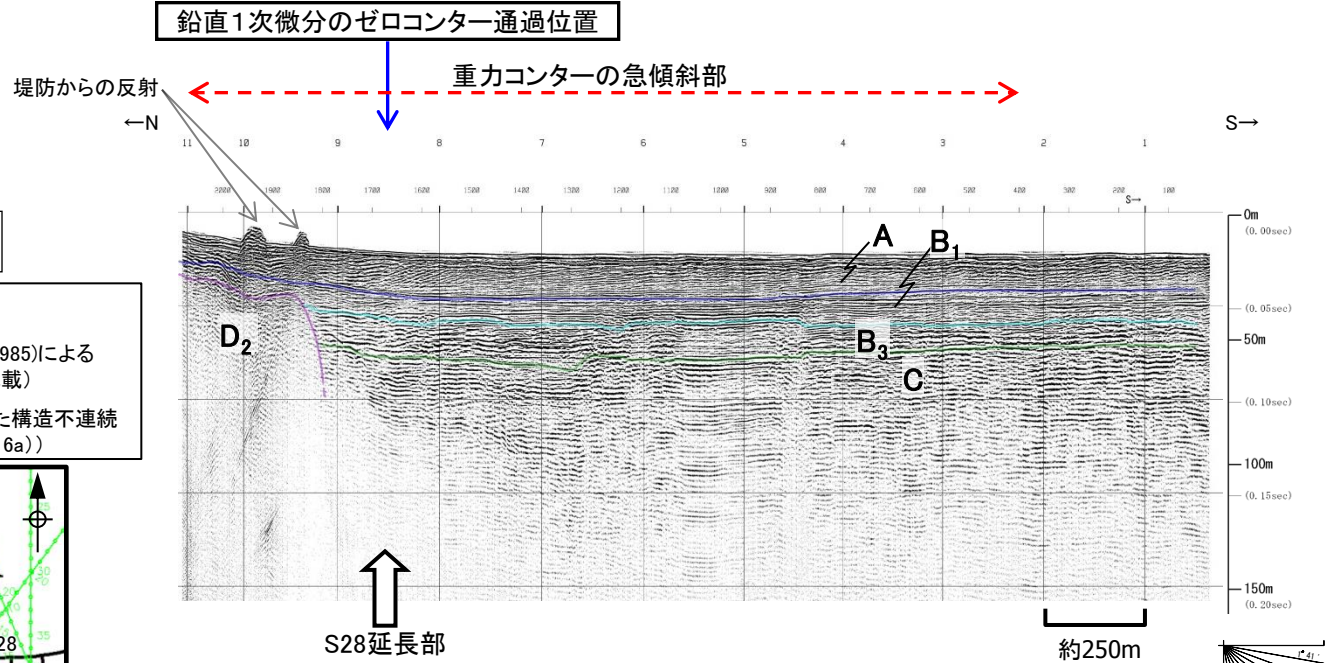
D-D'断面図(音波探査解析図: No.203BM7-マー・マルチチャンネル)
