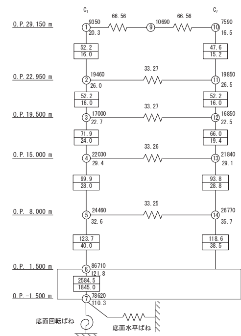
地震応答解析モデル(EW方向)
