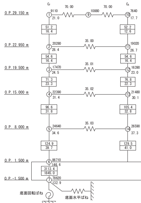
地震応答解析モデル(NS方向)
