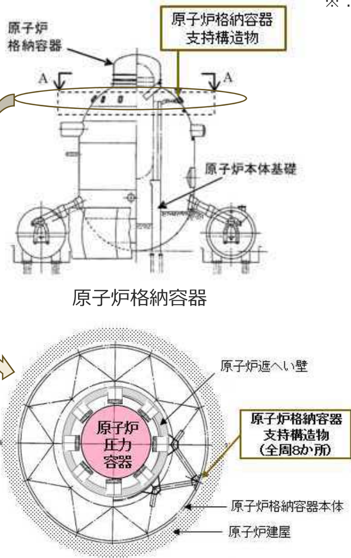
A-A'断面図
