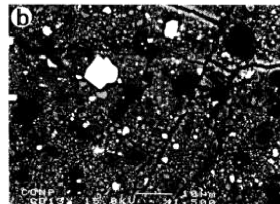
第7図 断層ガウジとシュードタキライト互層のSEM像(XX面)。a: 断層ガウジの断面にさらにシュードタキライトの層が含まれる。b: aの拡大。Pt: シュードタキライト。
