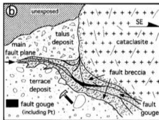
第3図 平林露頭(第1図のLoc. 1)の写角 (a) と詳細スケッチ (b)。断層破碎帯は花崗岩側に形成されたクレーサイト・岩塊角礫・断層ガウジおよびシュードタキライトから構成される。
