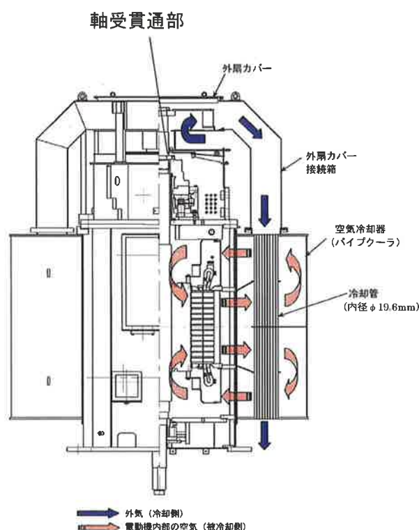
図4 海水ポンプモータの冷却方式
