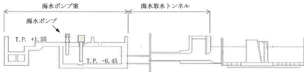
図-2 海水ポンプ室及び海水取水トンネルの形状
