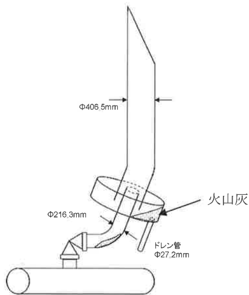
図1 主蒸気安全弁排気管の構造図
