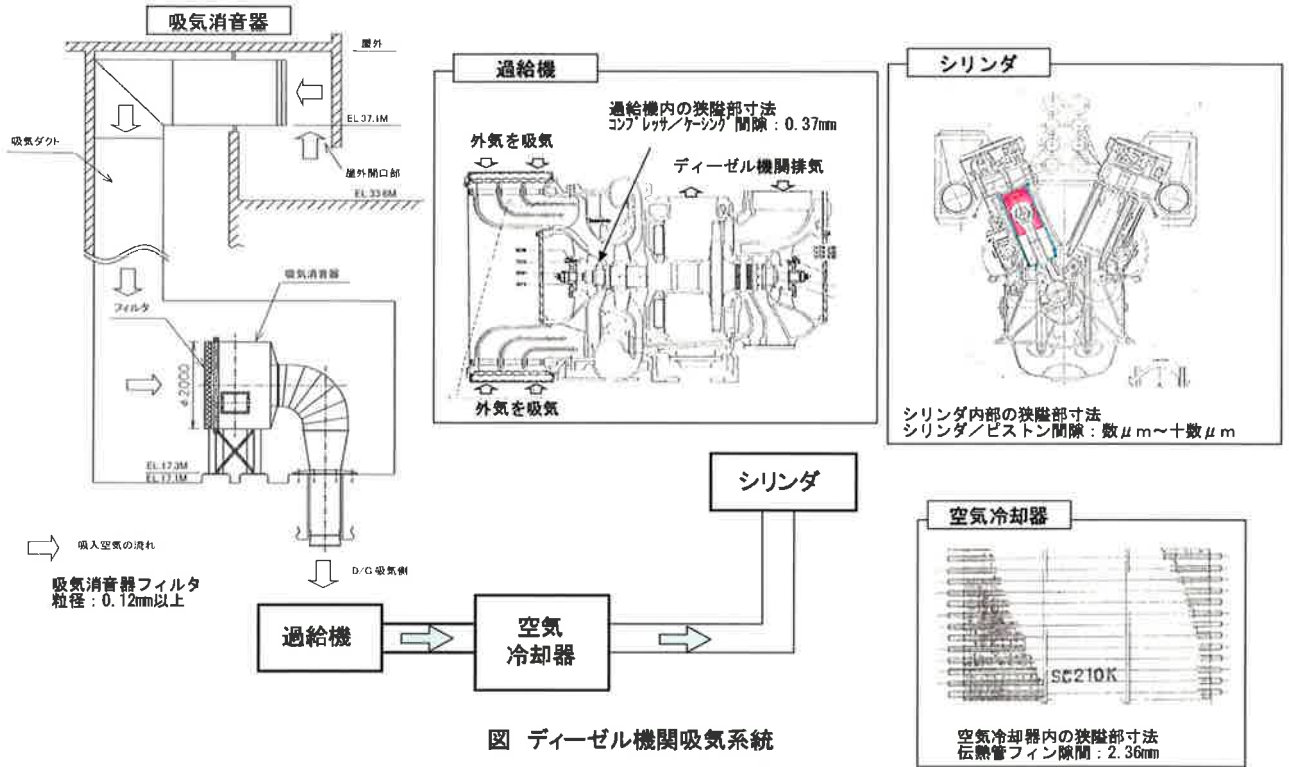
図 1 ディーゼル機関の吸入空気の流れ
