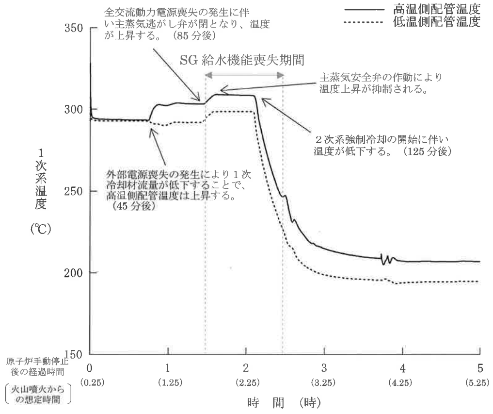
第5図 1次系温度 (高温側、低温側)
