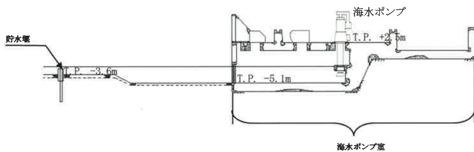
図-2 海水ポンプ室の形状
