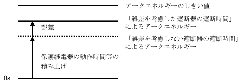
図 6-1 アーク放電の遮断時間の考え方
