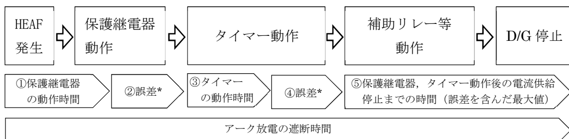
図 6-2 遮断器の遮断時間に含まれる誤差の考え方 (2/2)
