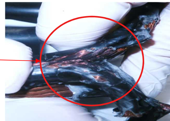
導体の状態 (相間が一体になっている)
