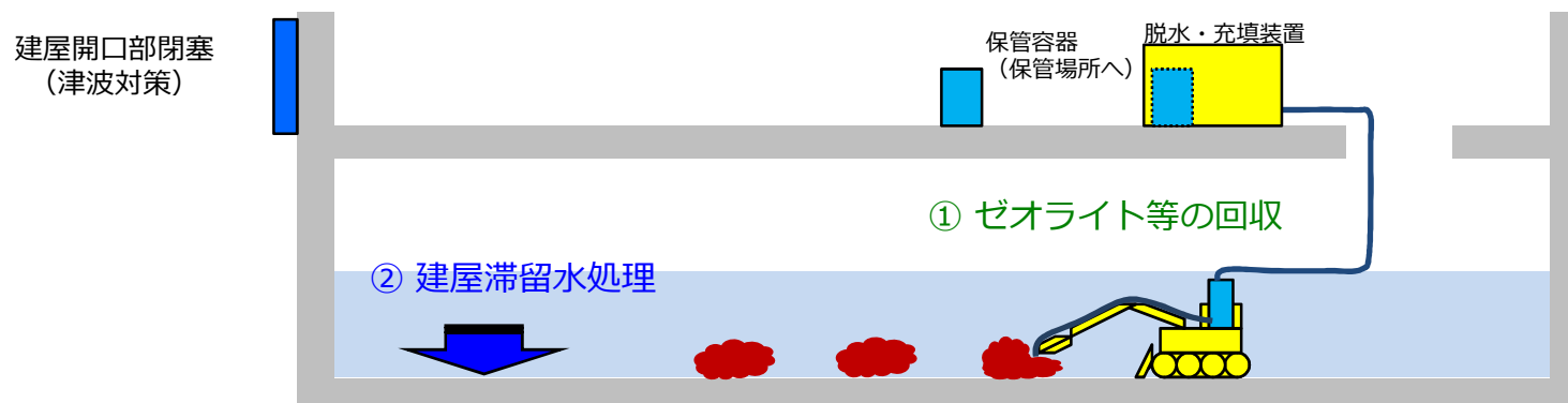
ゼオライト土嚢等の対応方針の概念図
