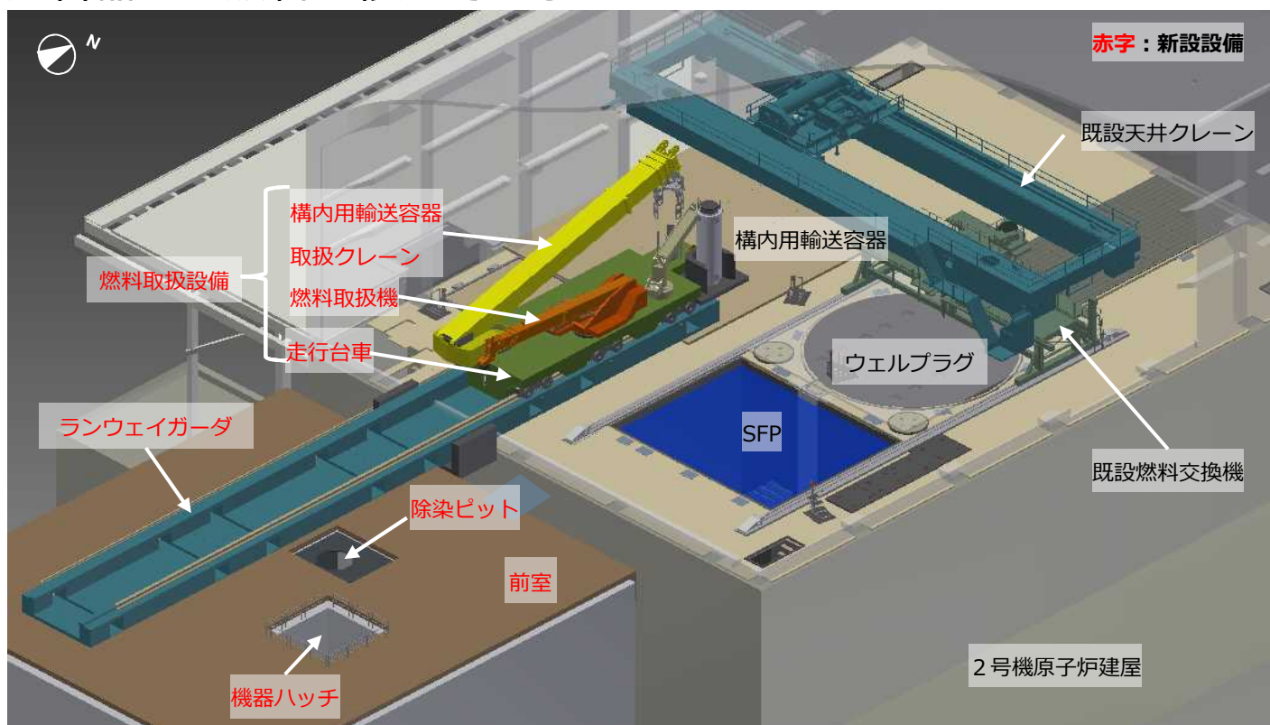
燃料取扱設備概念図
