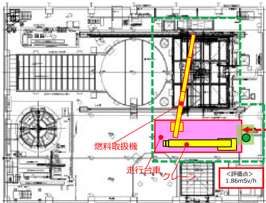
燃料取扱機油圧系統不具合イメージ
