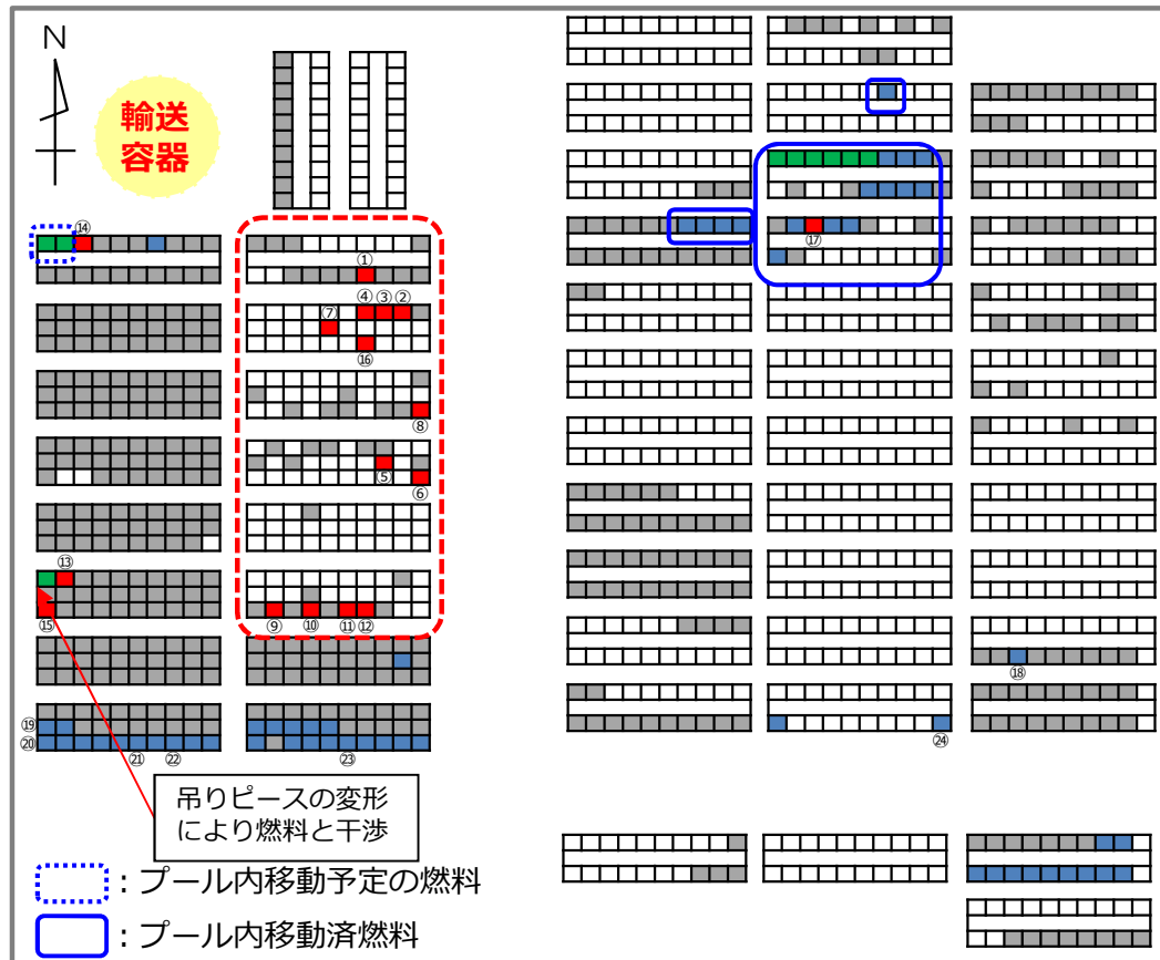
3号機使用済燃料プール（69回目までの取り出し状況を反映）
