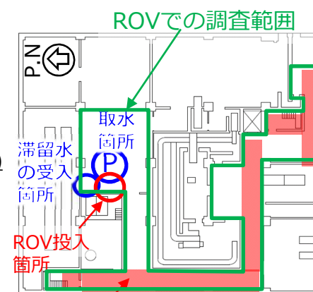
土嚢の存在を確認した範囲
