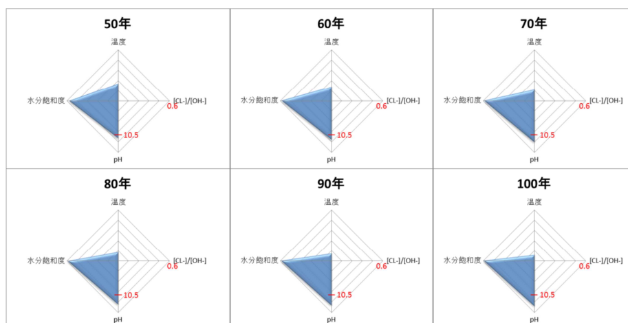
図 4.2-16 オーバーパックの不動態破壊型局部腐食の生起可能性に関するレーダーチャート（モンモリロナイト溶解速度 1/10 のケース）
