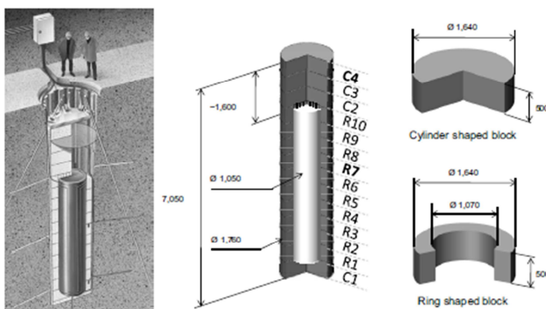
図 4.3-5 CRT の概略図 (24)
