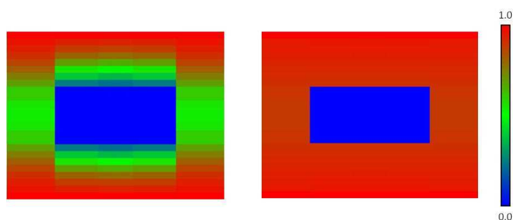
図 4.2-15 30 年後の水分飽和度分布(左:温度勾配水分拡散係数 10 倍,右:リファレンス)
