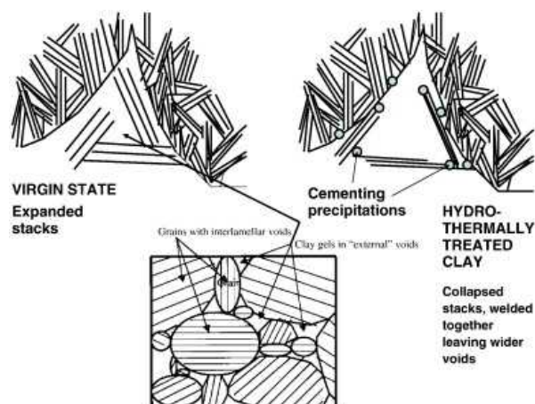
図 4.3-9 加熱による空隙の拡大に伴う透水係数の増大とケイ酸塩鉱物の沈殿に伴う剛性の増大を引き起こすと考えられるメカニズム
