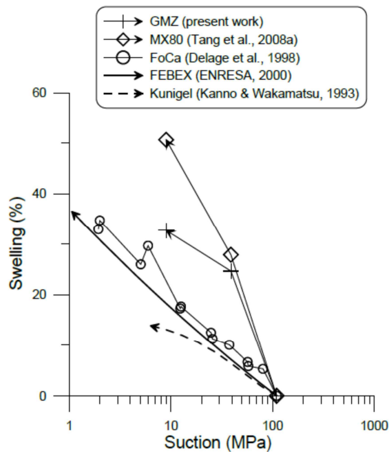
図 4.3-8 同一の初期サクションからの各種ベントナイトの膨潤挙動の比較 (27)
