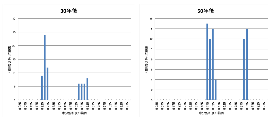
図 4.2-14 オーバパック表面水分飽和度ばらつきの時間変遷（温度勾配水分拡散係数 10 倍）
