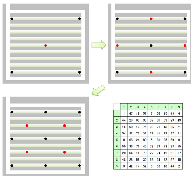
図 4.2-4 既に定置した廃棄体の中間に新たな廃棄体を定置するルールの概念
