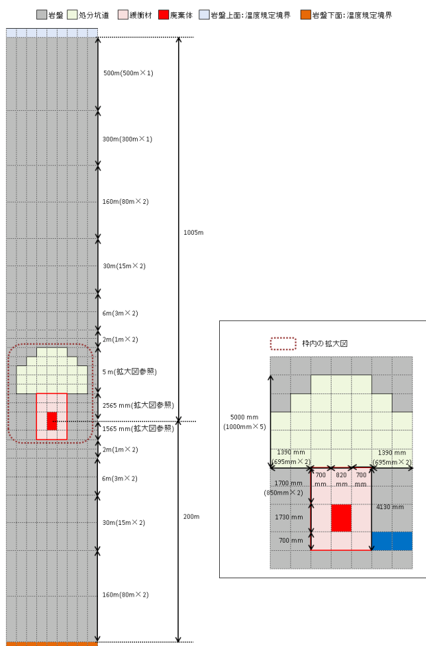
図 4.2-5 廃棄体 1 本のセルのジオメトリ（廃棄体を含む垂直断面）
