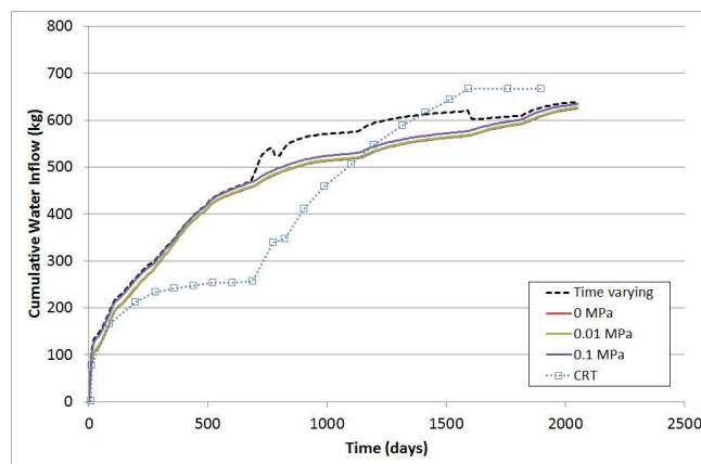
図 4.3-13 緩衝材への水の累積流入量についての試験結果（水色）と QPAC 解析結果の比較
