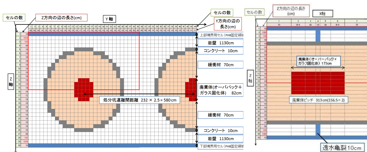
図 4.2-7 例題 2 における多変量セルラーオートマタの解析体系
