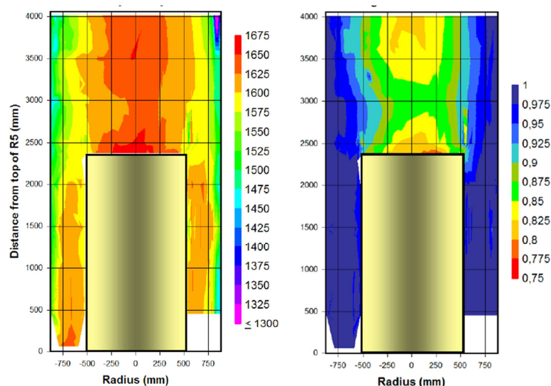
図 4.3-6 最大 5 年間の加熱・冠水の後に掘削したときの CRT での緩衝材の状態 乾燥密度 ( \text{kg/m}^3 ) (左) と飽和度 (右) (24)
