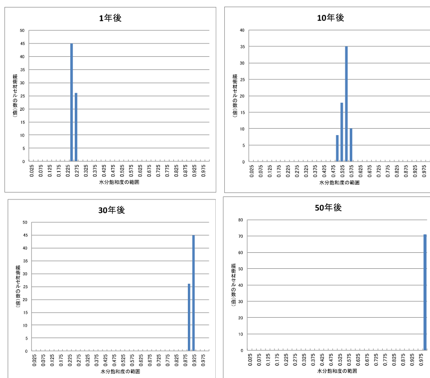
図 4.2-9 オーバーパック表面の水分飽和度のばらつきの時間変遷
