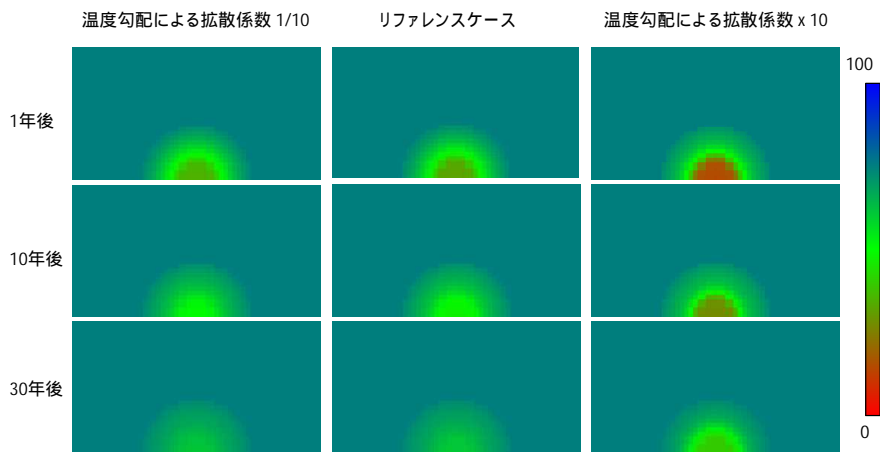
図 4.2-13 温度勾配による水分拡散係数の変動の影響（温度）
