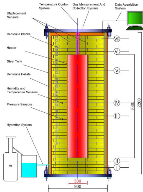
図 4.3-7 中国におけるモックアップ・テストの構成 (28)
