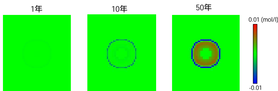
図 4.2-11 石英の累積溶解・沈殿量分布
