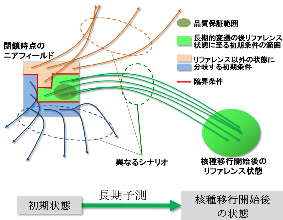
図 4.1-1 ニアフィールド環境長期変遷におけるシナリオ分岐に関する概念
