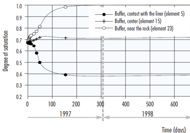
図 4.3-4 FEBEX 原位置試験の緩衝材中ベントナイト飽和過程のモデリング (23)
