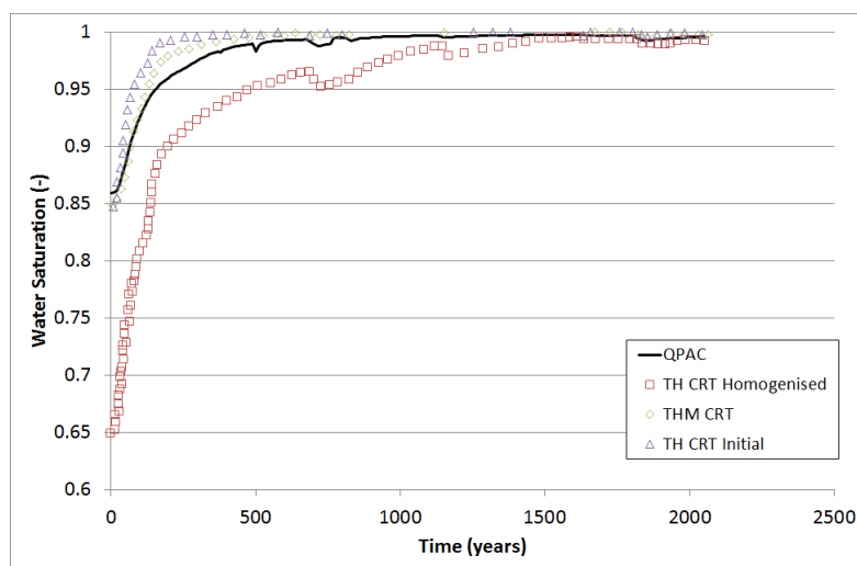
図 4.3-12 緩衝材中間点水分飽和度についての CODE_BRIGHT と QPAC 解析結果の比較
