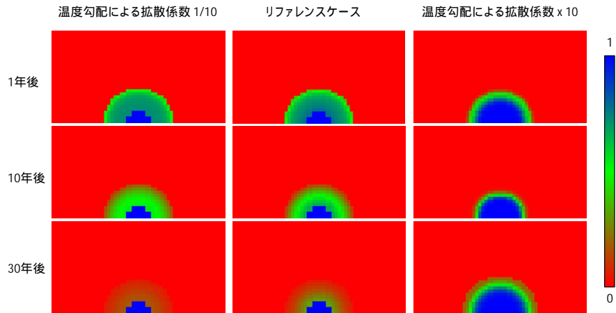
図 4.2-12 温度勾配による水分拡散係数の変動の影響（水分飽和度）
