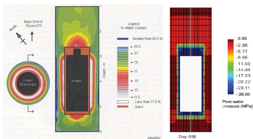
図 4.3-2 Buffer/Container 実験の試験終了時緩衝材内の水分布の測定結果(左: Graham et al. (22) ) と同等の間隙水圧モデルによる計算結果(右: Guo (18) )
