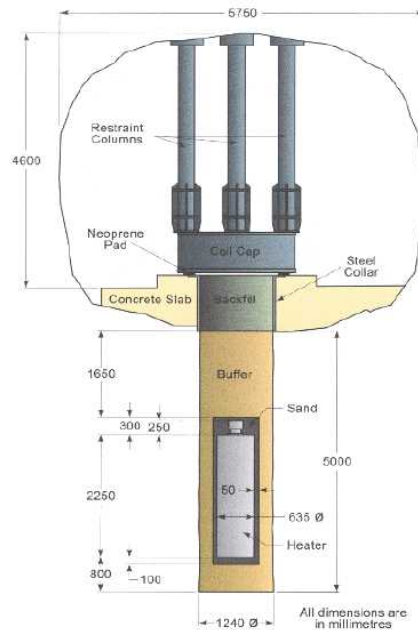
図 4.3-1 Buffer/Container 実験のジオメトリ (18)
