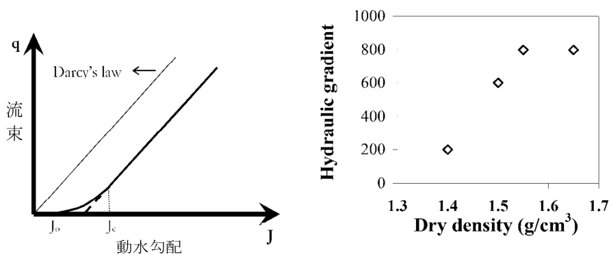
図 4.3-15 Dixon et al. (33) による非線形流動モデルの概念（左）及び FEBEX ベントナイトを対象とした測定可能な流動開始の動水勾配についての試験結果（右） (32)
