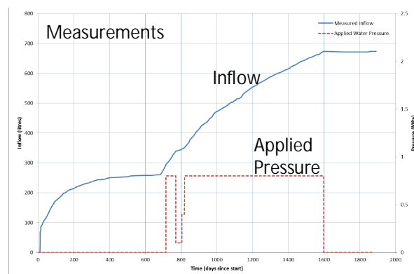
図 4.3-14 CRT 試験における外側境界条件（水圧）と累積流入量の関係
