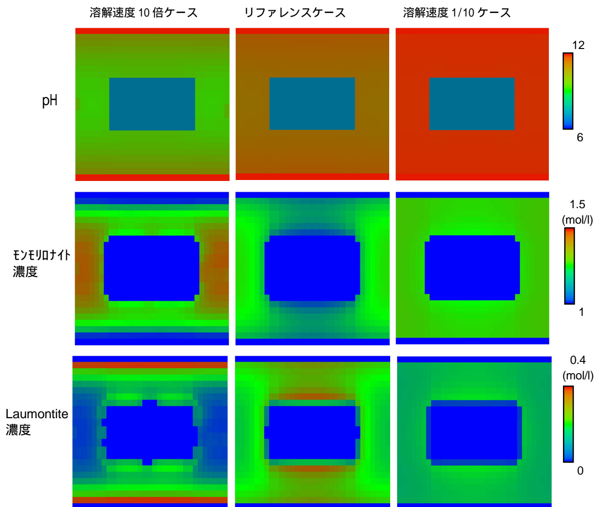
図 4.2-17 モンモリロナイト溶解速度の影響( 廃棄体中央坑道方向鉛直断面 ,1000 年後 )
