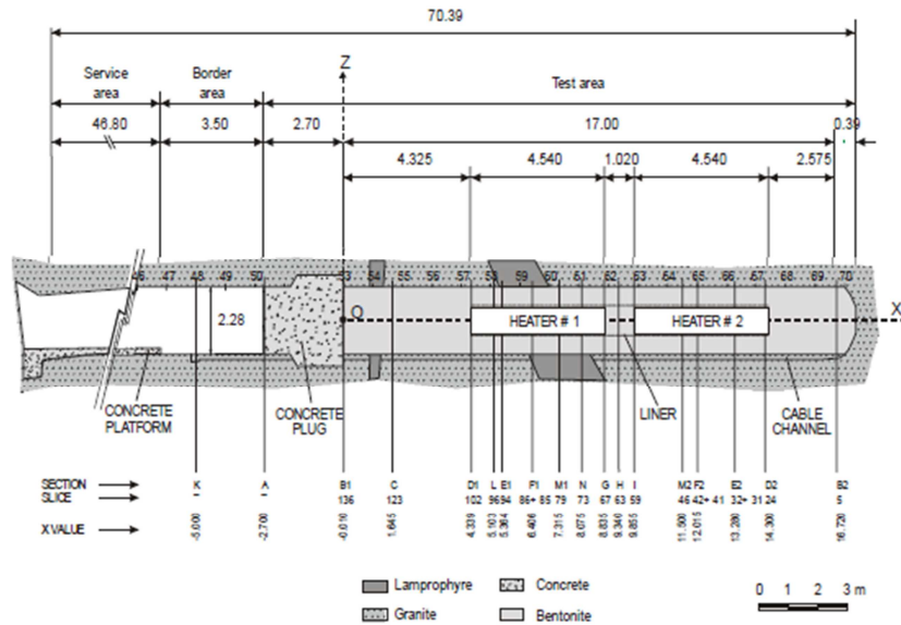
図 4.3-3 FEBEX 原位置試験の詳細レイアウト (23)
