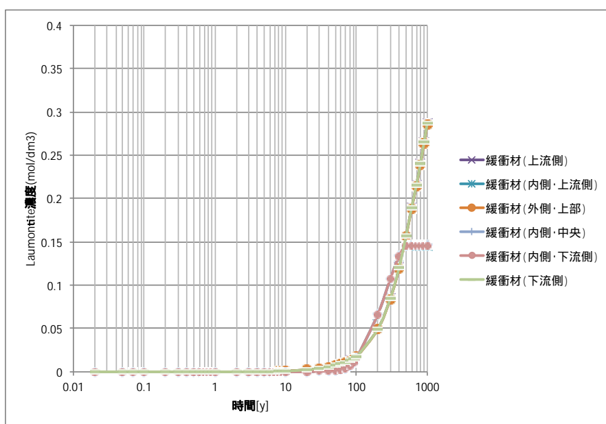
図 4.2-10 緩衝材中各部での Laumontite 生成量の時間変化
