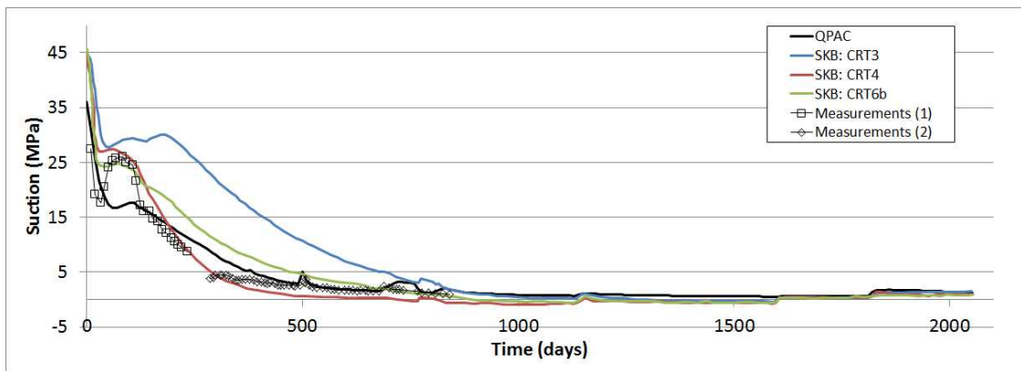
緩衝材内側表面付近のサクシオン時間変化
