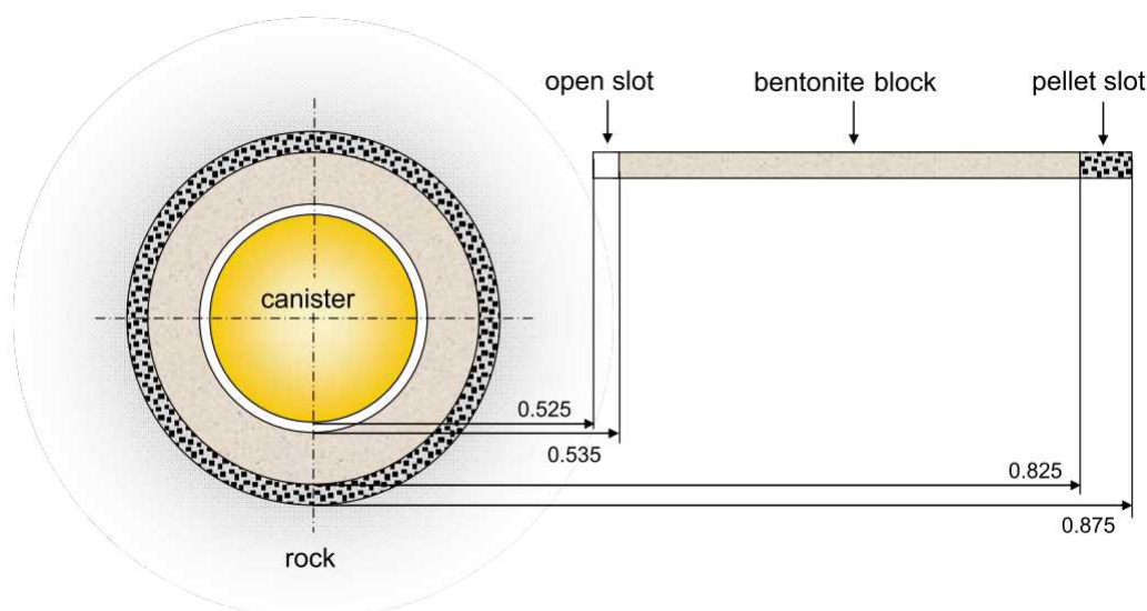
図 4.3-10 CRT 試験に対応する 1 次元モデル体系 (CODE_BRIGHT 及び QPAC 共通)
