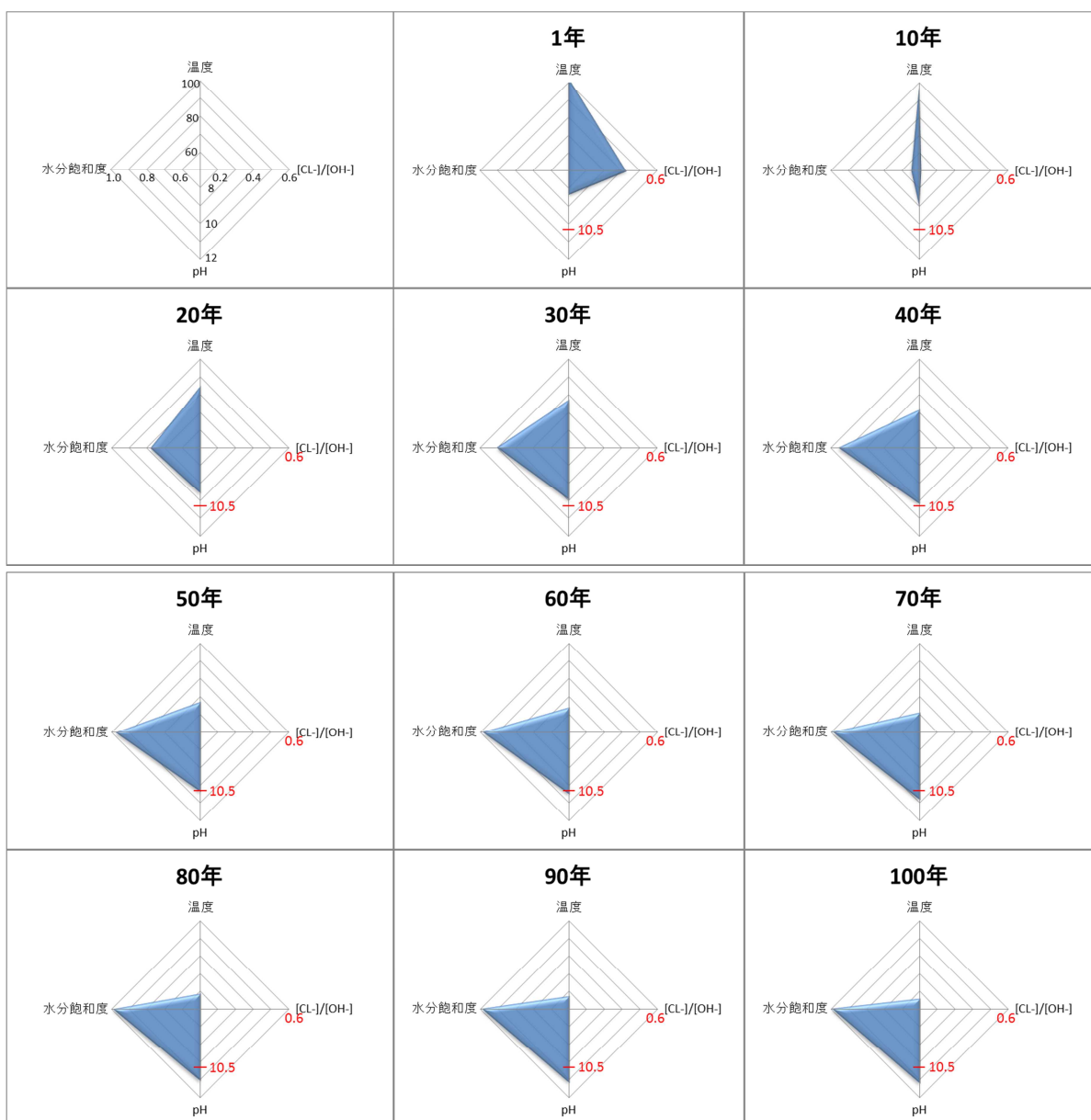
図 4.2-8 オーバーパックの不動態破壊型局部腐食の生起可能性に関するレーダーチャート
