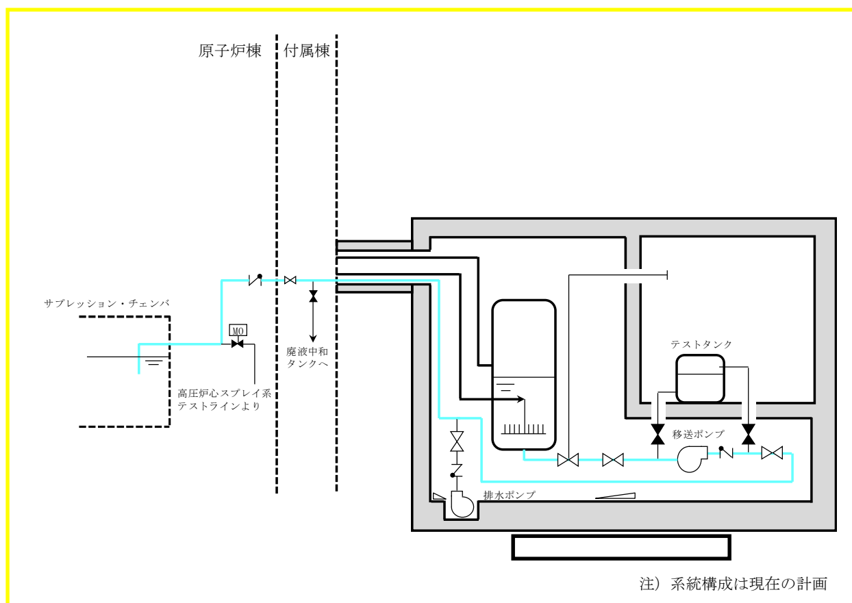
第9図 移送ライン系統概要図
