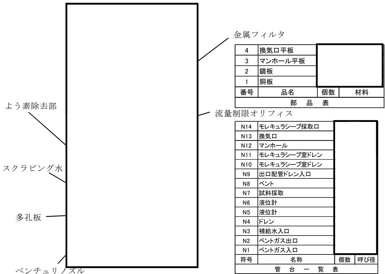
第 2.3.2-1 図 フィルタ装置概略図
