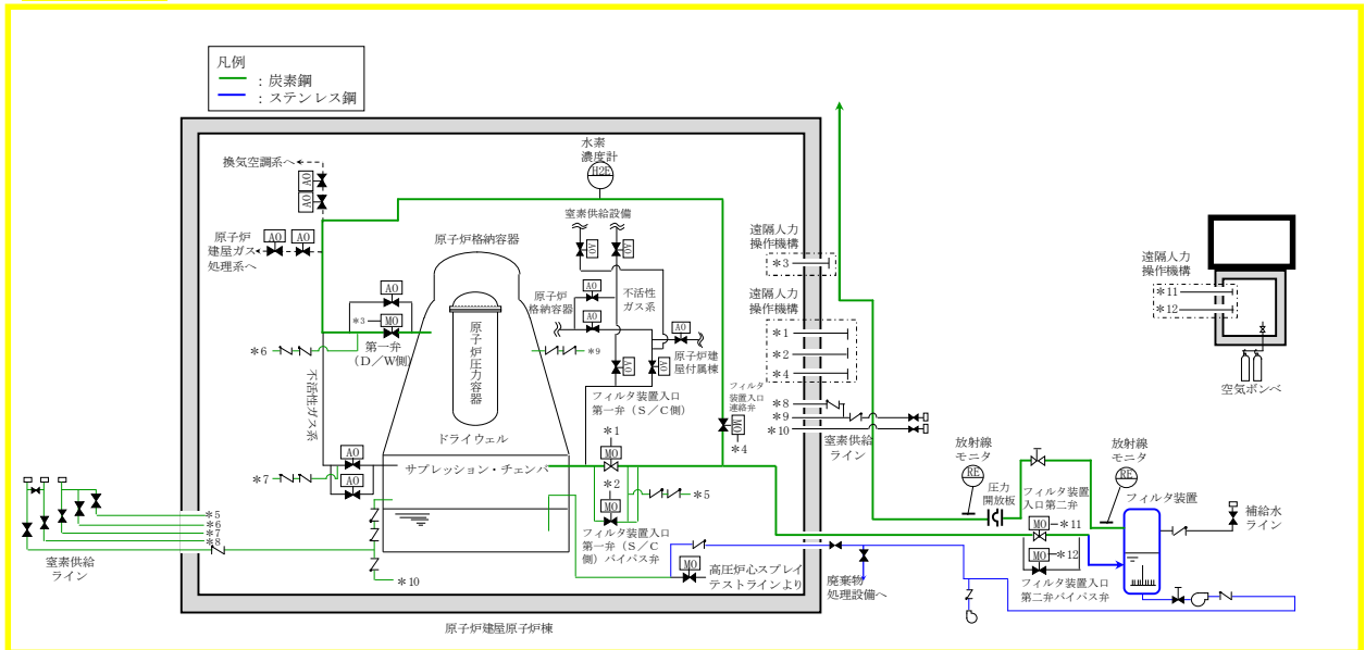
第 2.3.1-2 図 フィルタ装置及び配管の材質範囲
