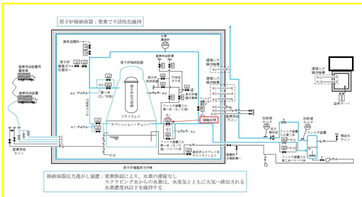
第 4 図 ベント停止後状態概要図
