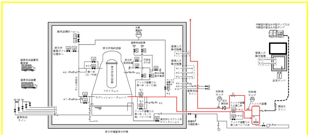
第4.2.2-1図 スクラビング水補給時の系統状態概要図
