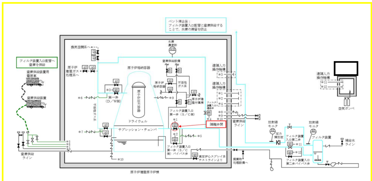
第 4.1.3-8 図 窒素供給概要図 (ベント停止後)
