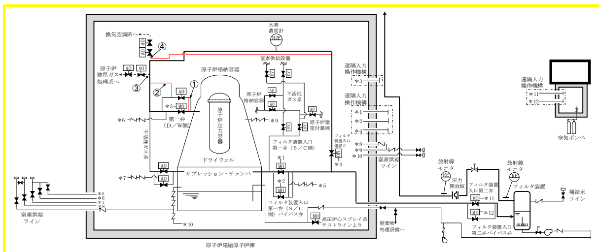
第 4 図 ベントライン設置概要図
