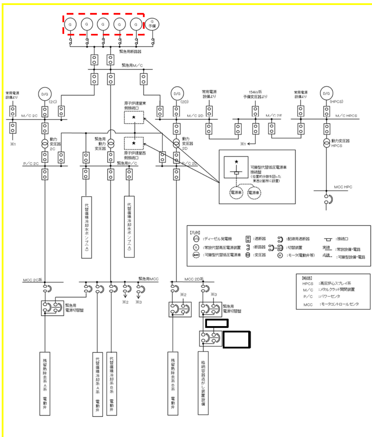
第 1 図 常設代替交流電源設備による電源給電範囲 (交流電源)
