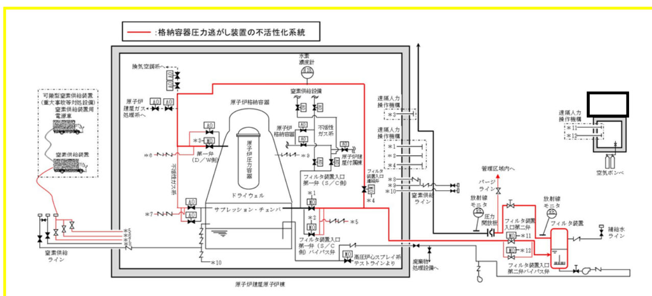
第 1 図 格納容器圧力逃がし装置の不活性化系統
