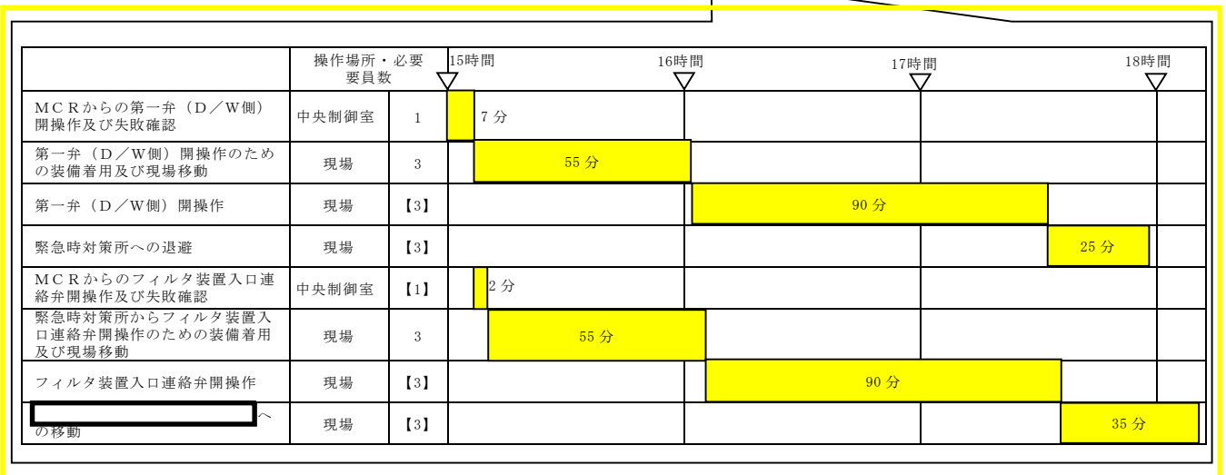
第4.1.3-5図 ベント準備操作のタイムチャート (1/2)
