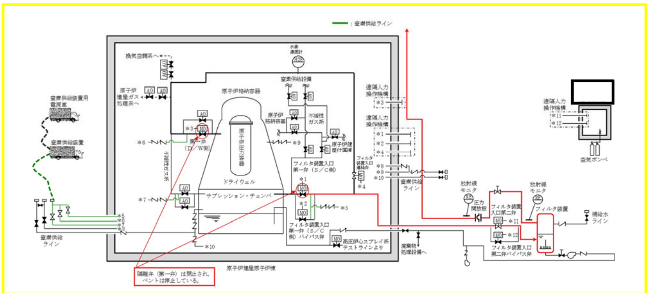
第4.2.3-1図 窒素供給時の系統状態概要図
