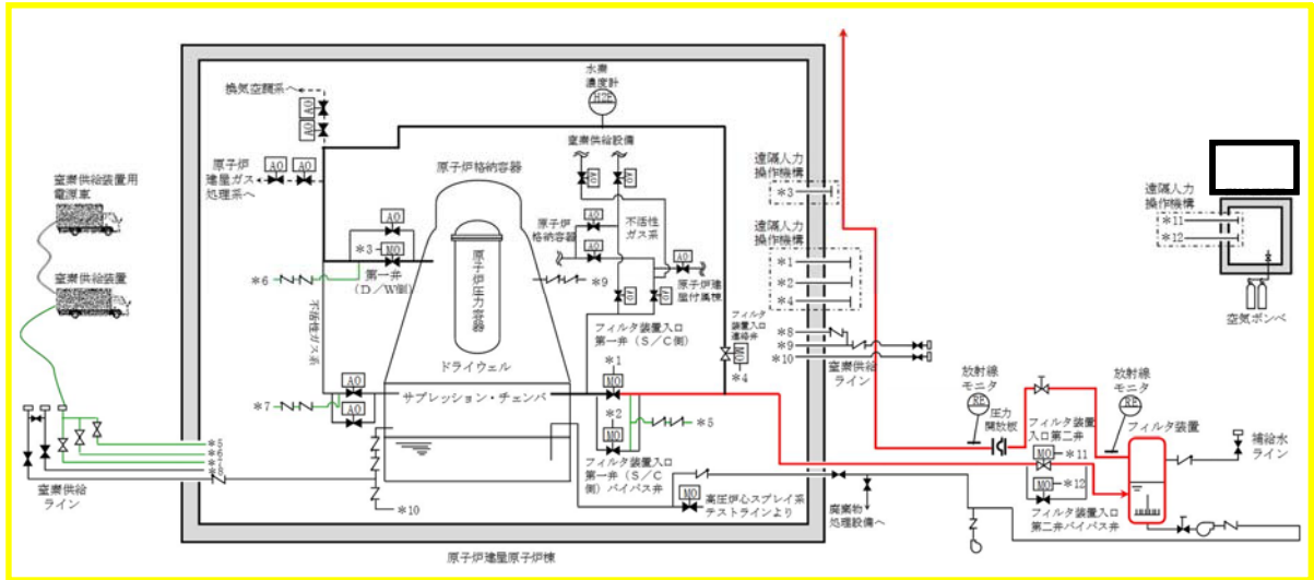
第 2.4.4-1 図 窒素供給設備概要図
