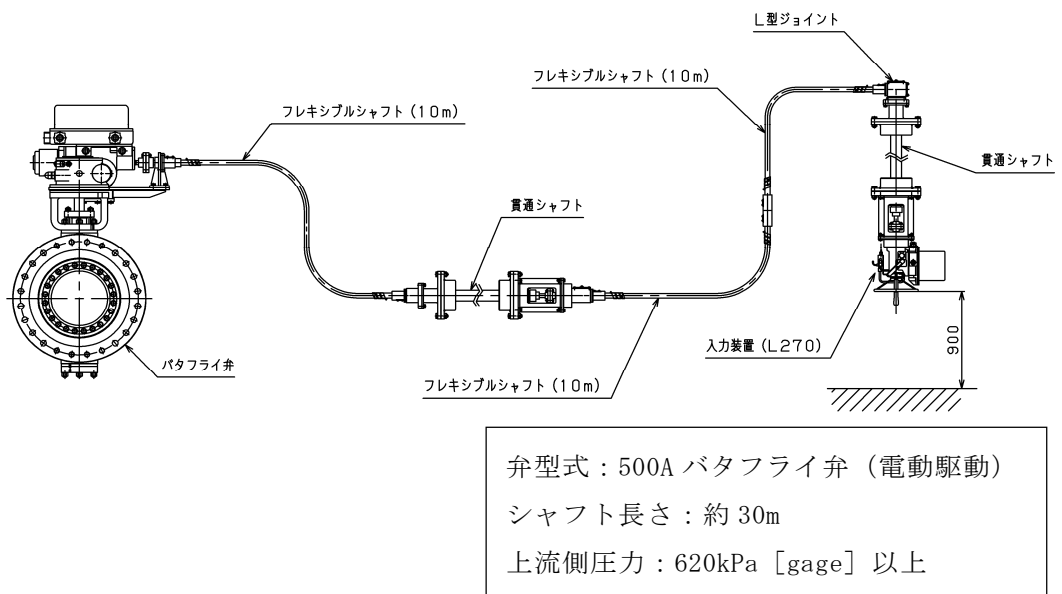
第3図 モックアップ試験の概要 (1/2)
