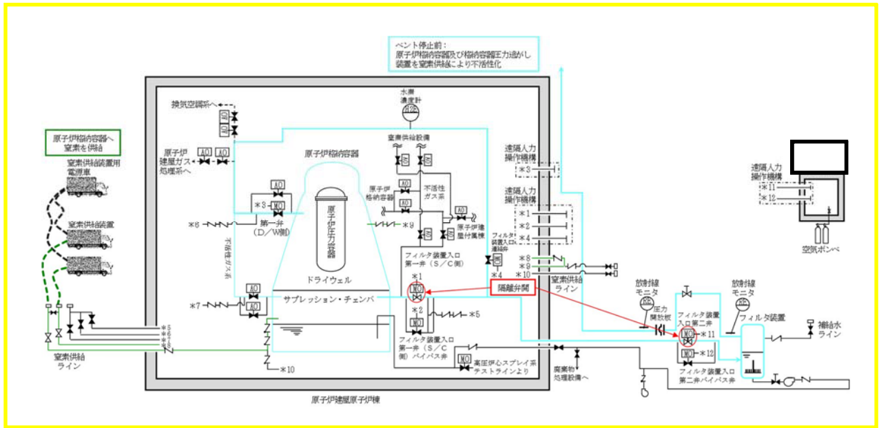
第 4.1.3-7 図 窒素供給概要図 (ベント停止前)
