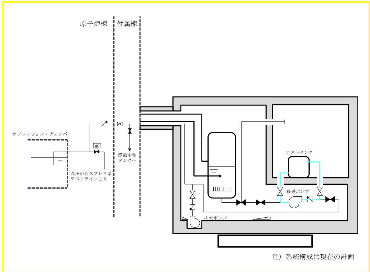
第 4.4-2 図 排水設備（移送ポンプ）作動試験概要図
