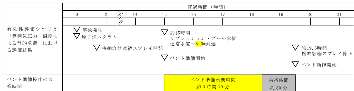
【炉心損傷を判断した場合のベント準備（第一弁（D/W側）の場合）】
