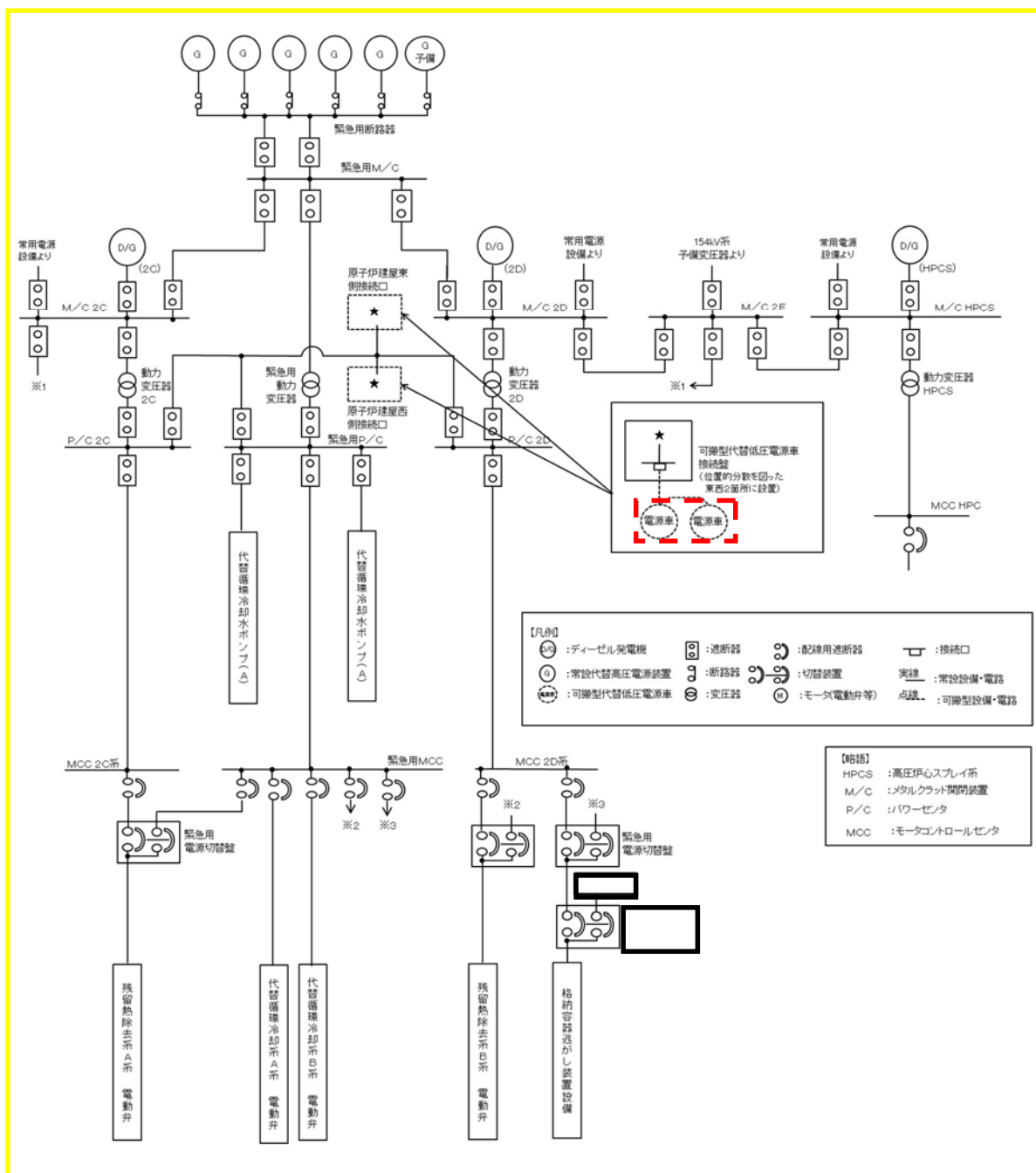
第 3 図 可搬型代替交流電源設備による電源給電範囲 (交流電源)
