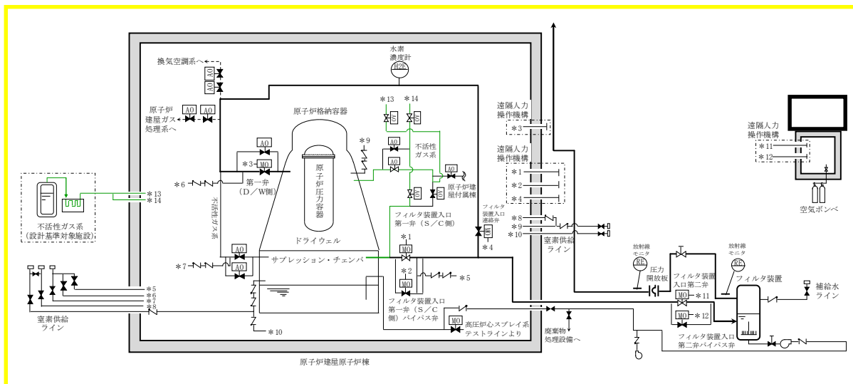
第 7 図 格納容器への窒素供給手段の概略図
