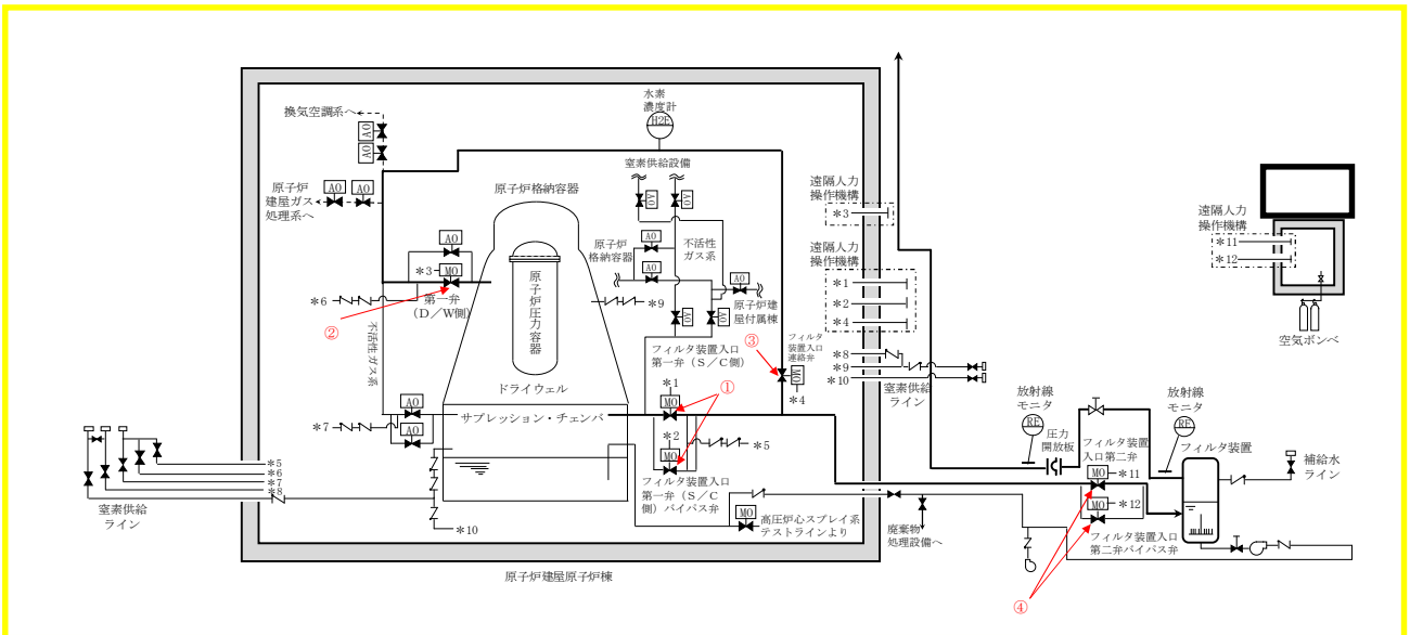
第 4.4-1 図 格納容器圧力逃がし装置機能検査対象弁
