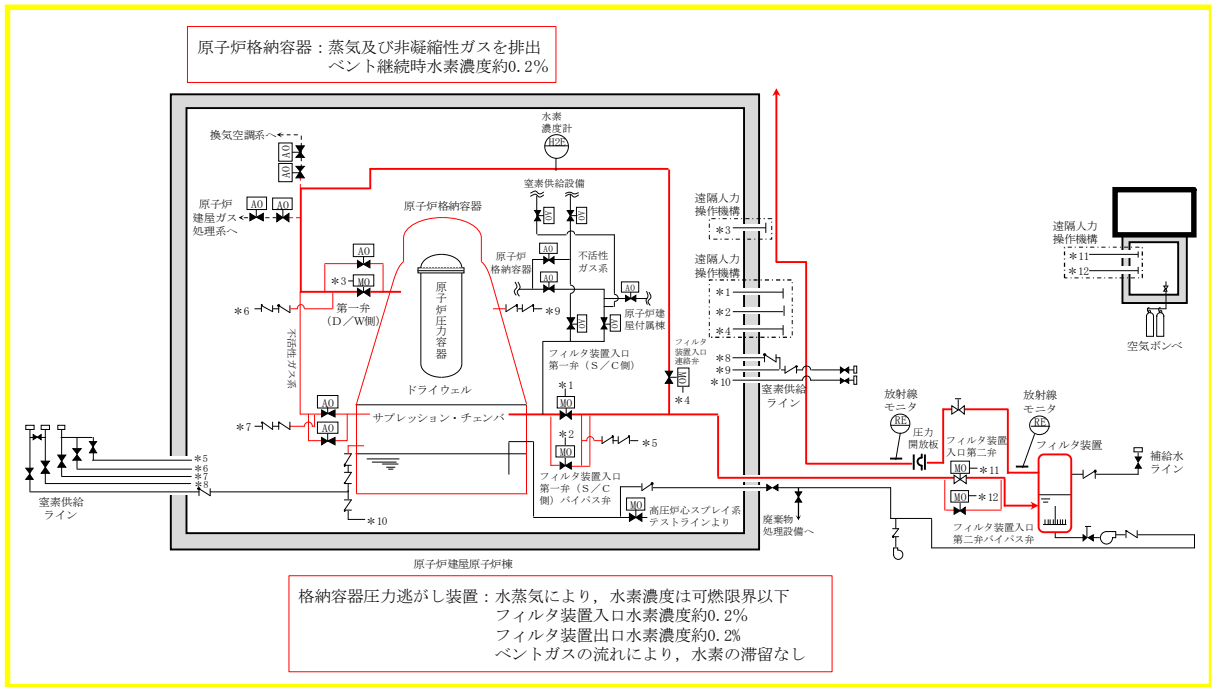
第2図 ベント実施時状態概要図
