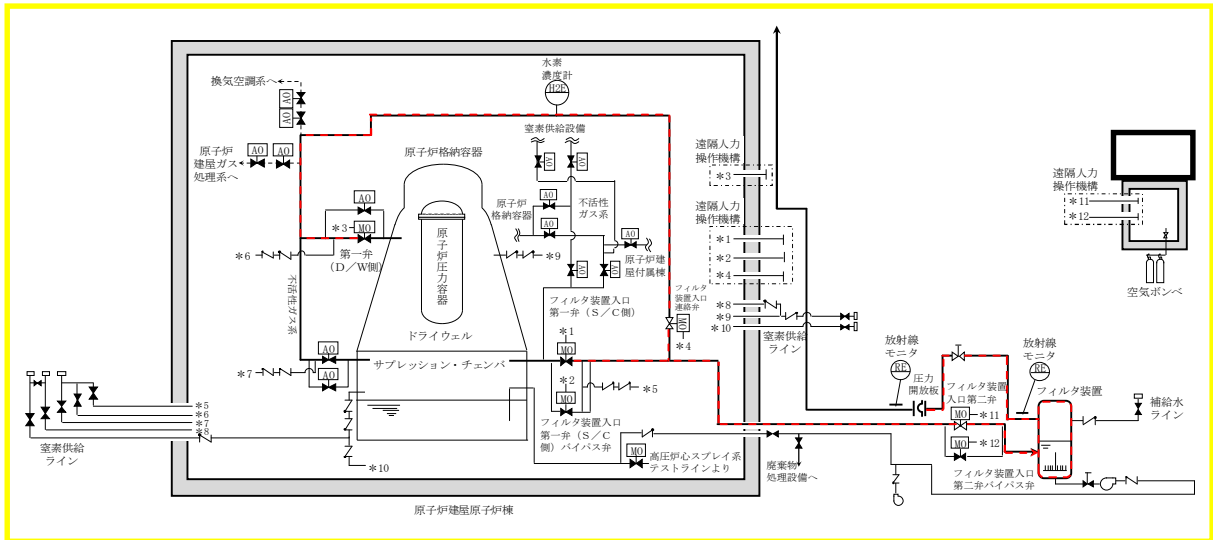
第4.4-3図 漏えい試験の試験概要図
