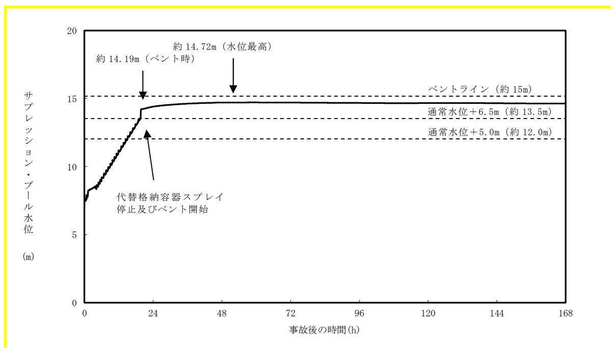
第 1 図 雰囲気圧力・温度による静的負荷（格納容器過圧・過温破損）
