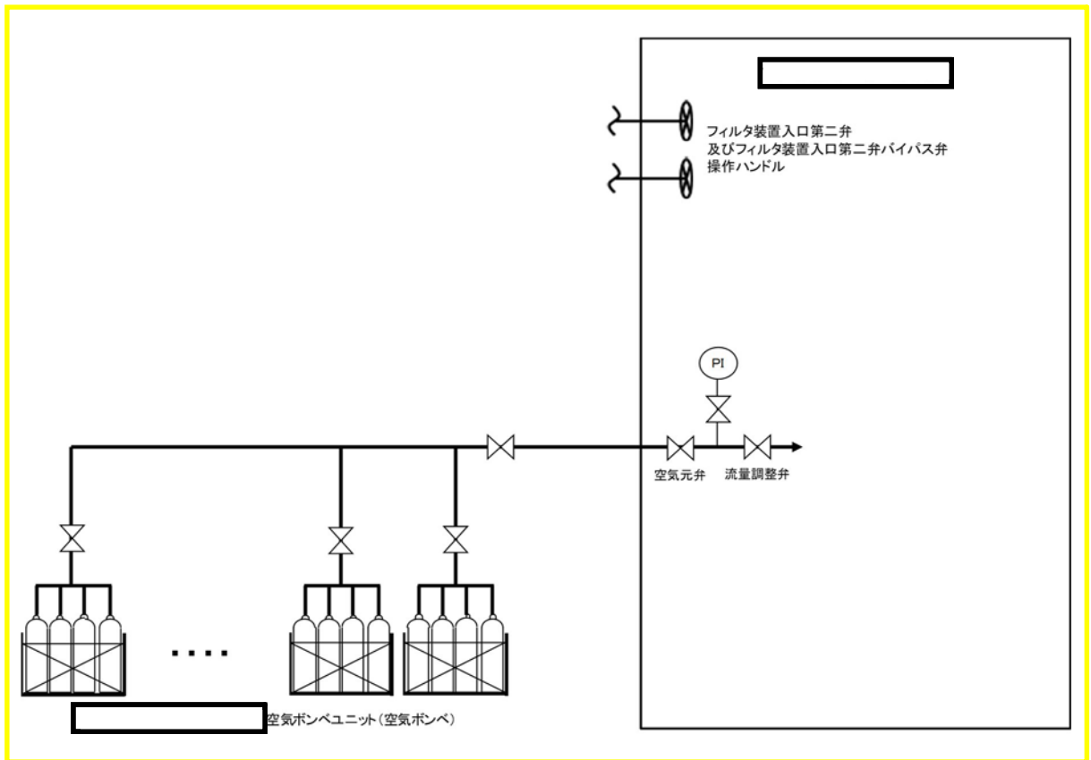
第 50-5-8 図 [ ] 空気ポンプユニット概要図
