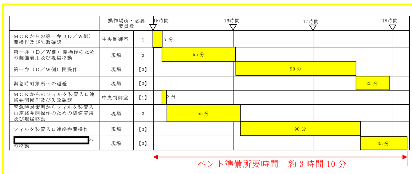
第1図 ベント準備所要時間タイムチャート
