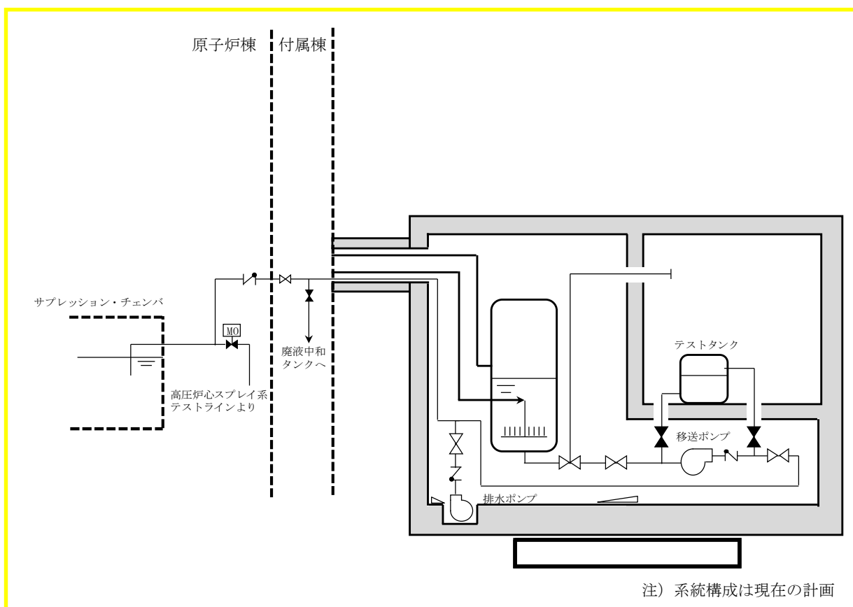
第 1 図 排水設備の構成
