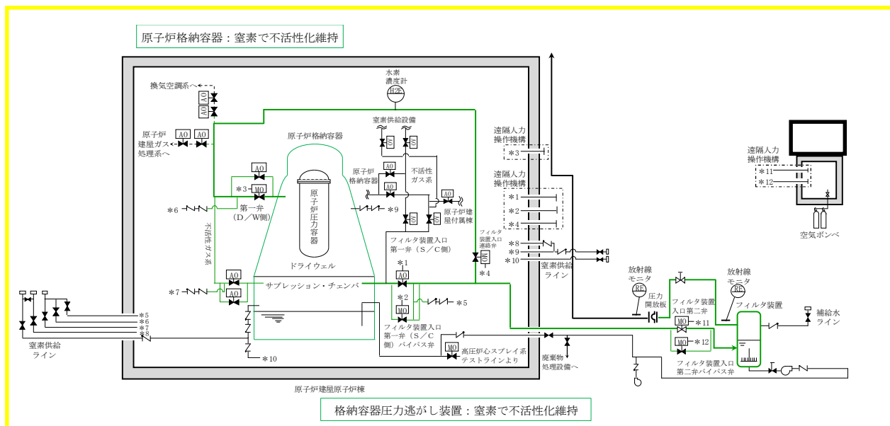
第1図 系統待機時の状態概要図
